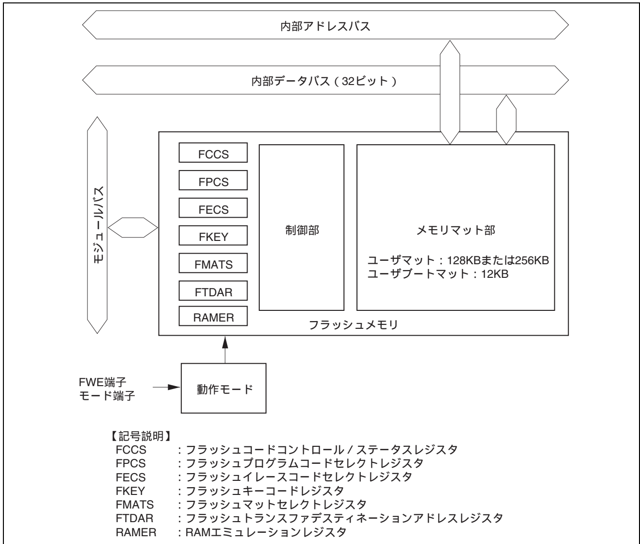
図3 フラッシュメモリのブロック図
