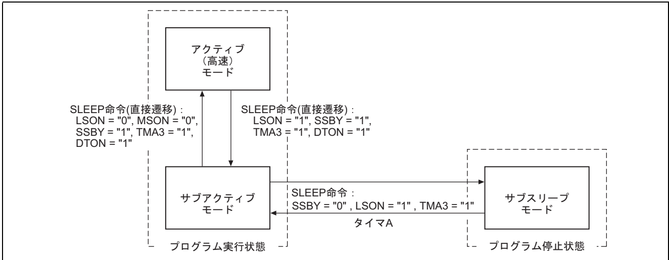
図1 サブスリープモードへのモード遷移図
