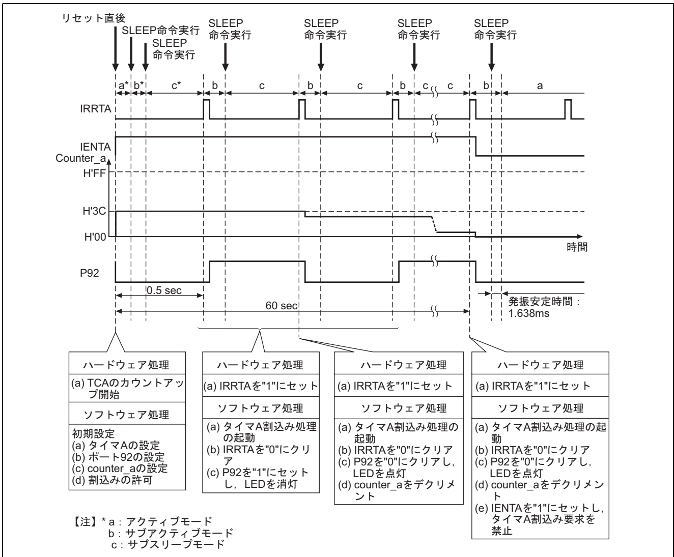
図 2 サブスリープモードへの遷移の動作説明
