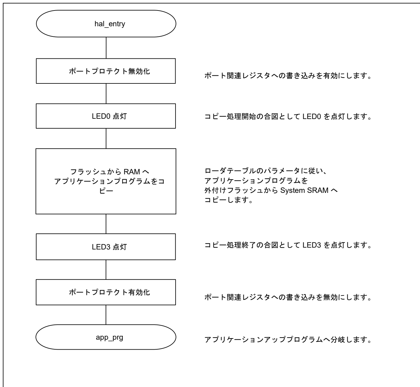
図 3.6 hal_entry 処理(ローダプログラム)
