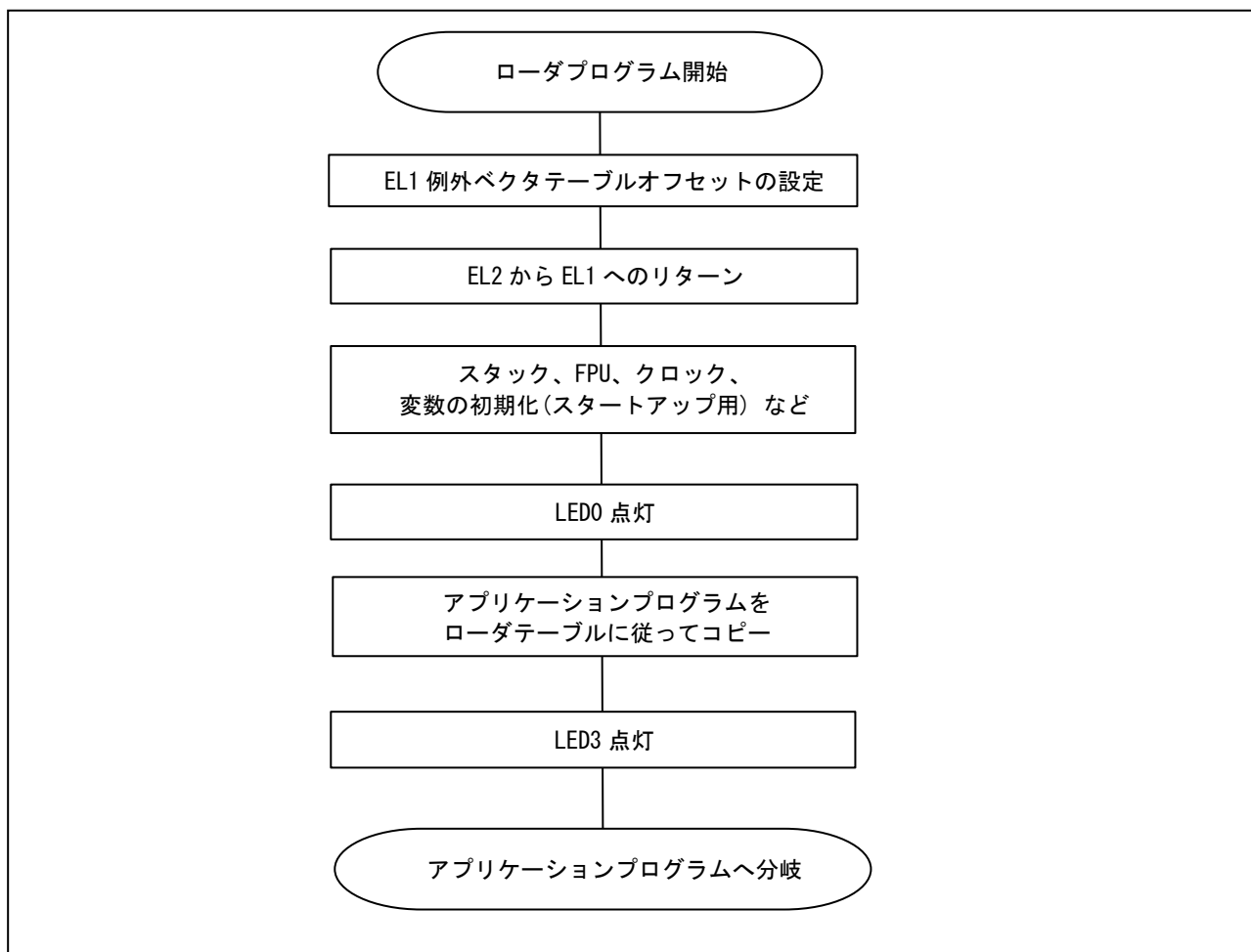
図 3.2 ローダプログラムの動作概要
