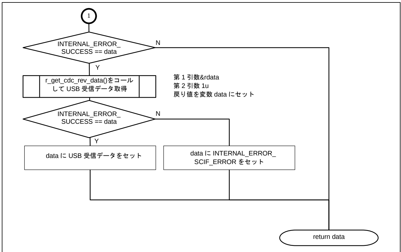
図 5.11 scif_getc 関数処理
