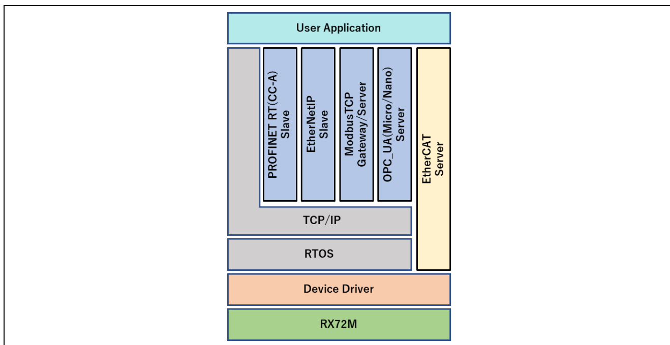
図 2.1 RX72M プロトコルスタックソフトウェア全体構成
