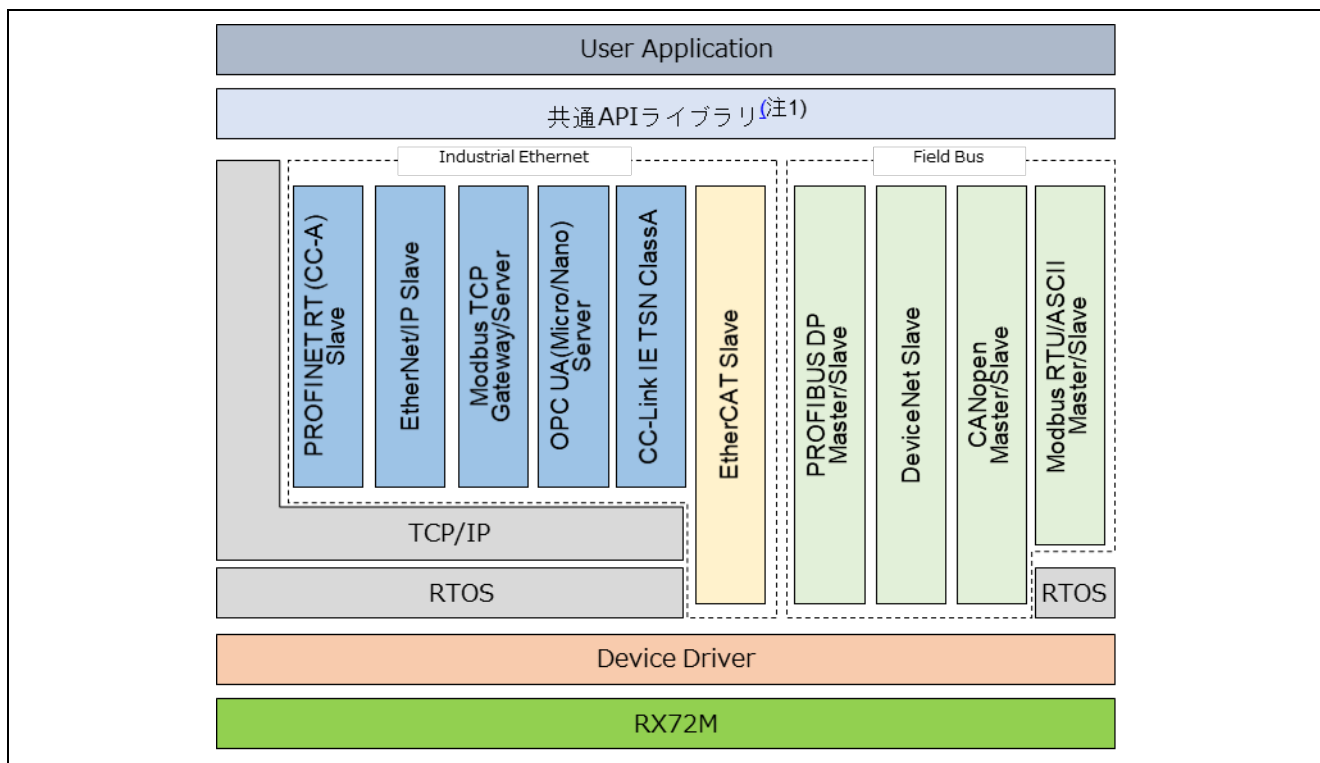
図 2.1 RX72M プロトコルスタックソフトウェア全体構成
