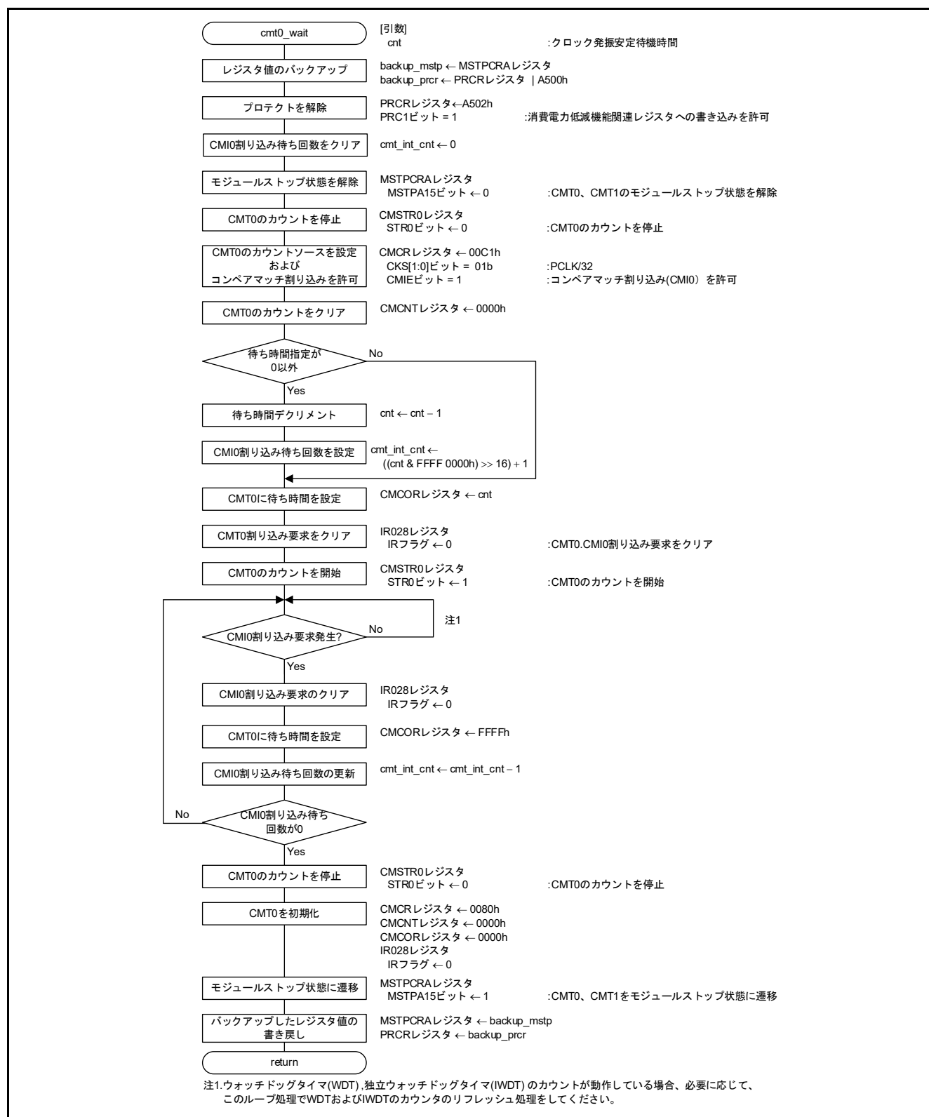
図3.12 CMT0によるソフトウェアウェイト
