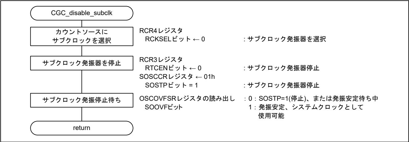
図 3.11 サブクロックの停止設定
