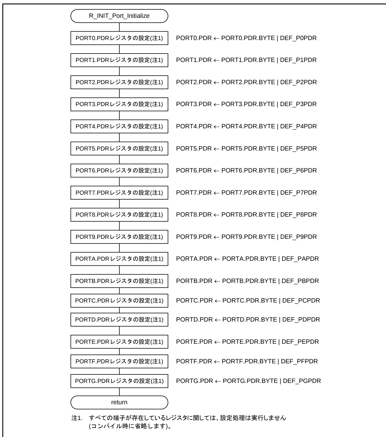
図 3.3 存在しないポートの初期設定
