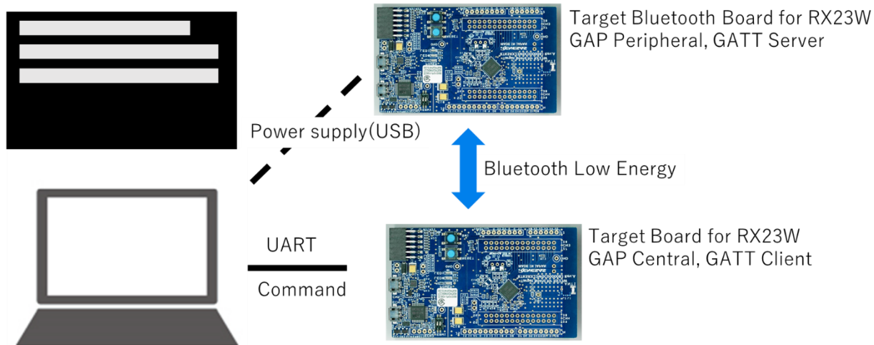
図 1.1 サンプルプログラムの動作セットアップ
