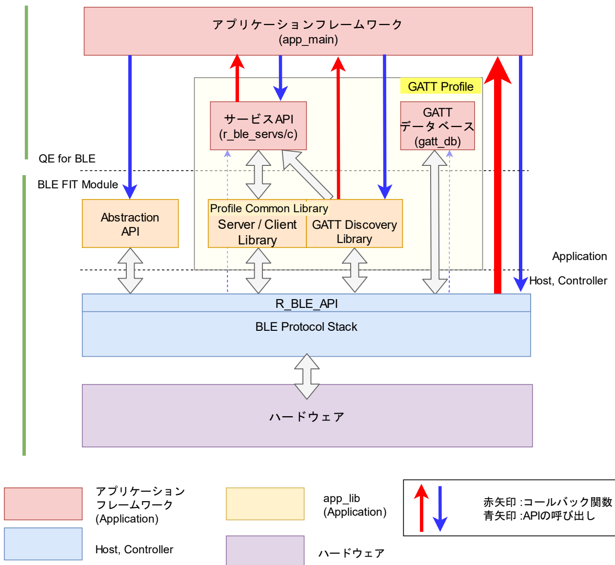
図 4.2 QE for BLE が生成するアプリケーションフレームワーク
