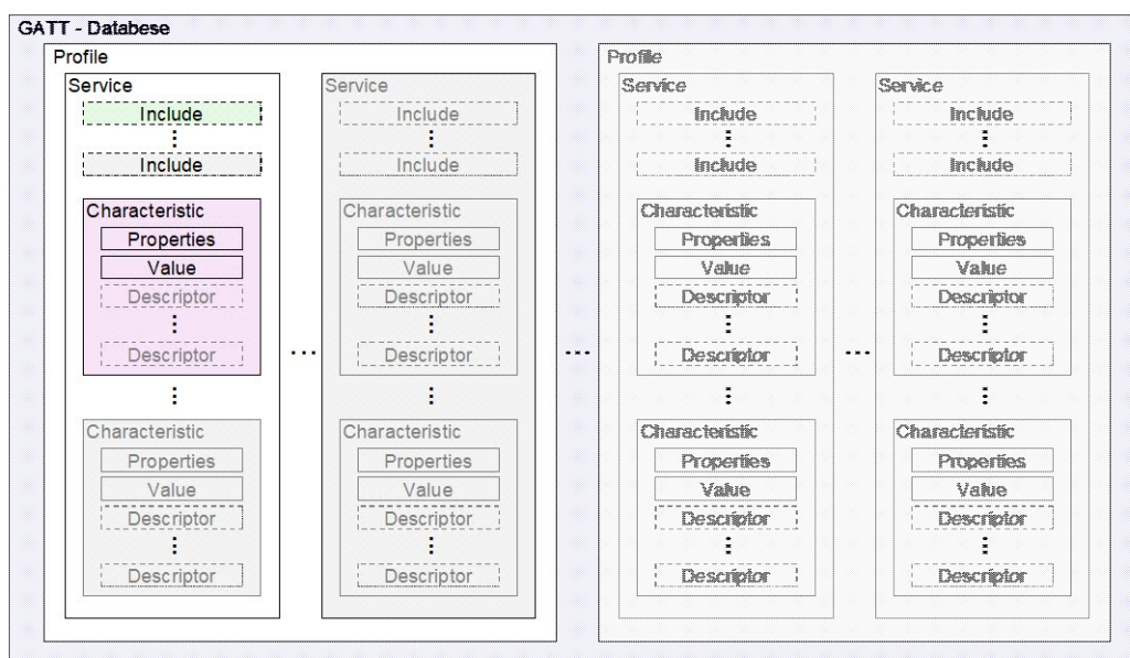
図 10-1 GATT データベースの構成
