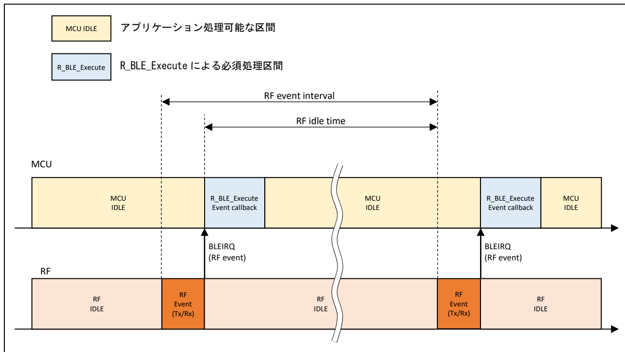
図 1-9 RF スリープを伴わない場合の MCU/RF 動作概要
