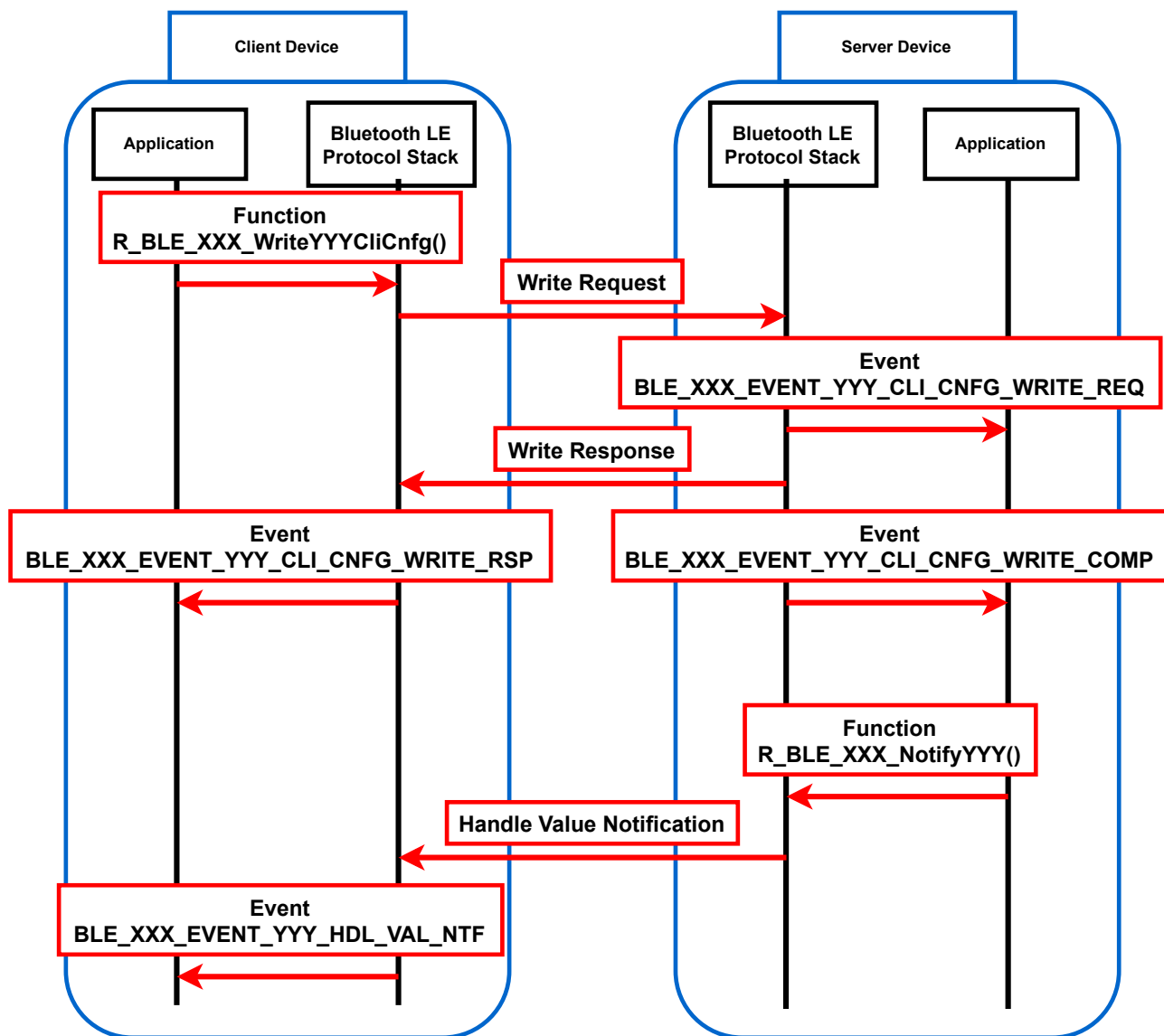
図 10-5 Notification 動作の実行手順
