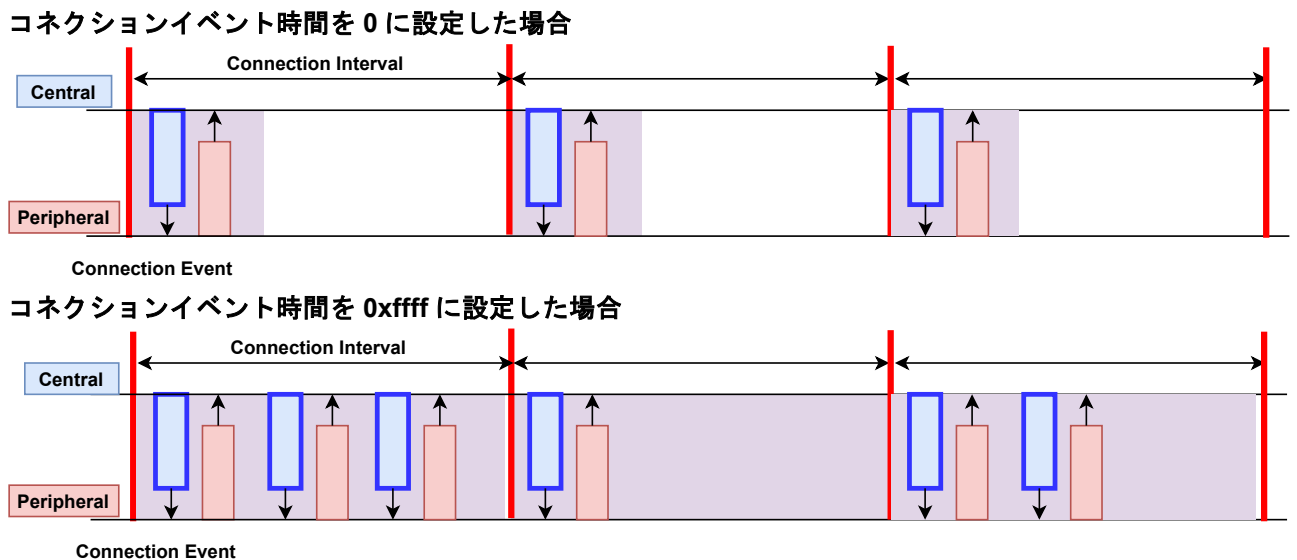
図 8-4 コネクションイベント時間とパケット交換の模式図
