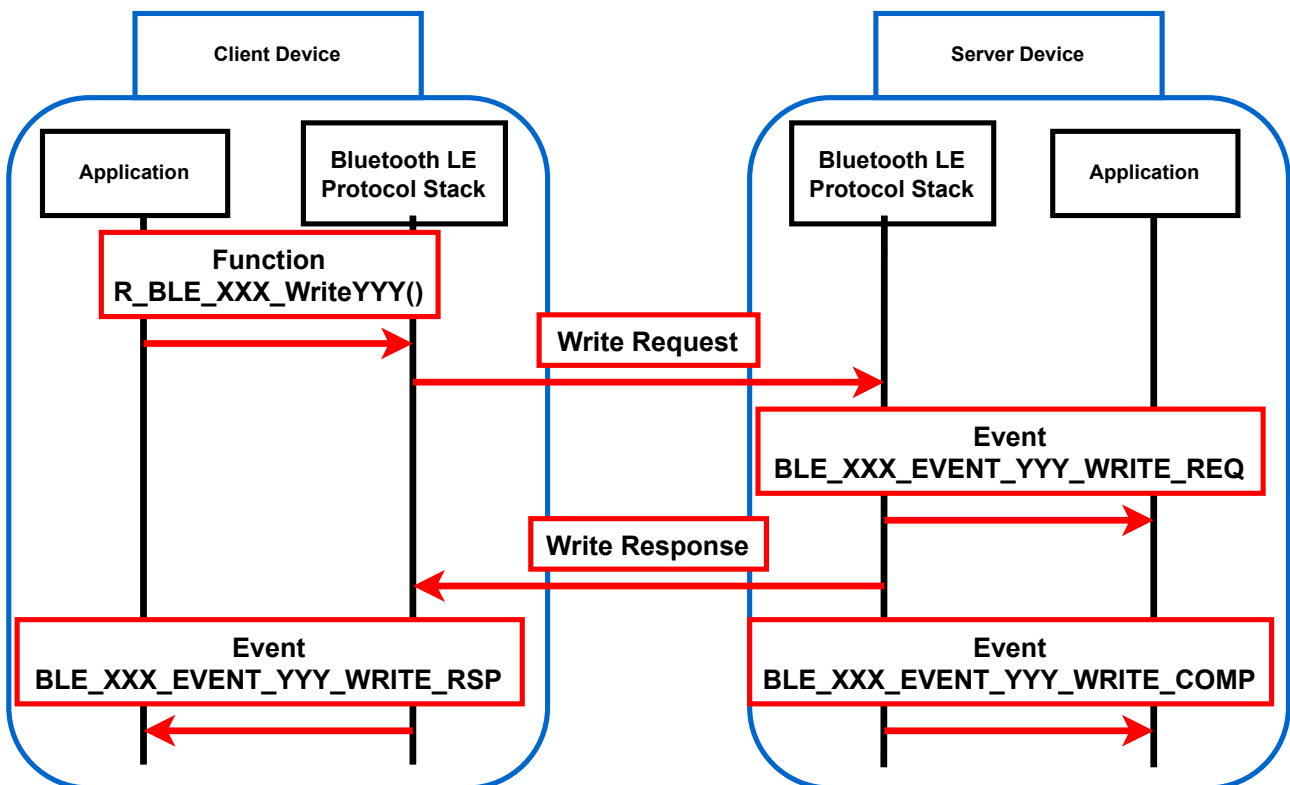
図 10-3 Write 動作の実行手順
