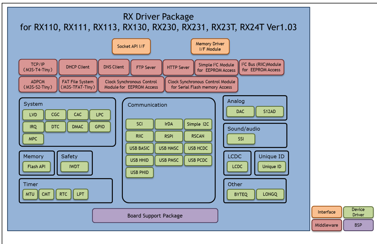
図 3-2 RX110, RX111, RX113, RX130, RX230, RX231, RX23T, RX24T グループ用 RX Driver Package FIT モジュール構成イメージ
