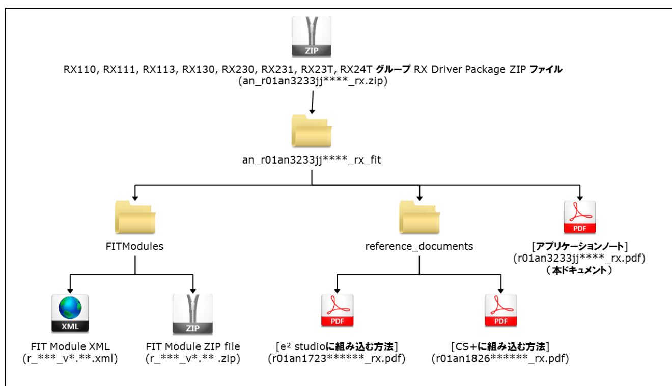
図 3-1 RX110、RX111、RX113、RX130、RX230、RX231、RX23T、RX24T グループ用 RX Driver Package フォルダ構成
