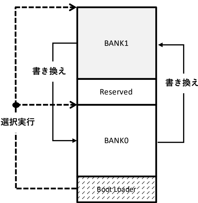
図 8-1 リニアモードのコードフラッシュ使用イメージ
