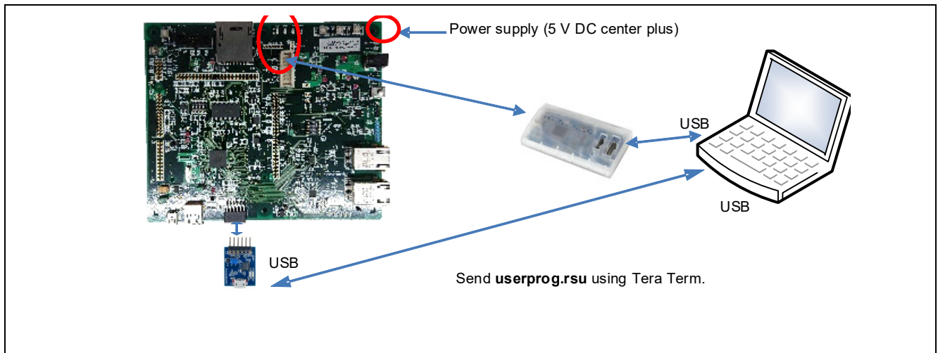
図 6-24 UART を使用したファームアップデートを行うときの RSK RX72M と PC の接続
