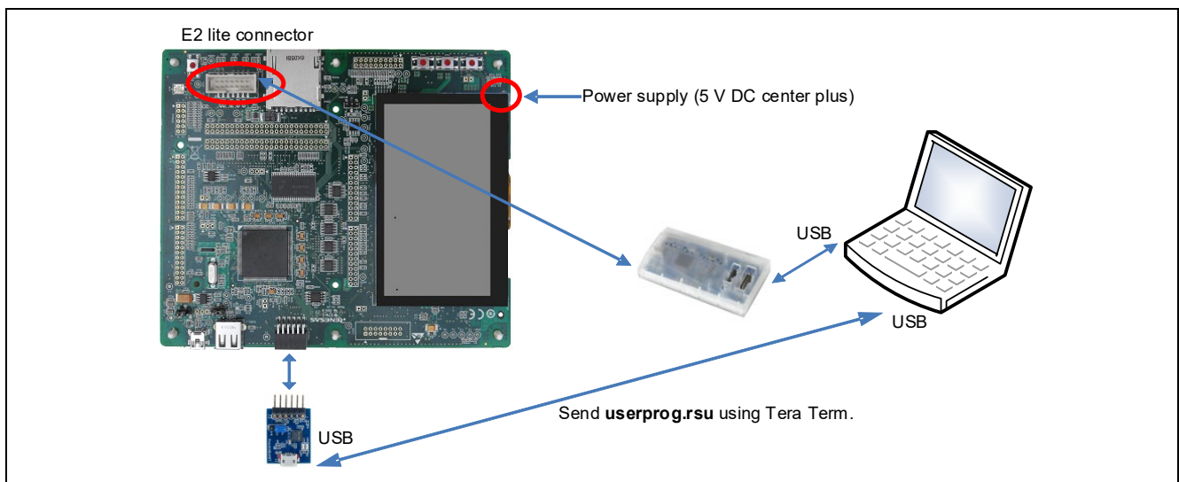
図 6-17 UART を使用したファームウェアアップデートを行うときの RSK RX65N-2MB と PC の接続
