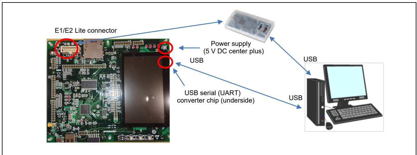
図 6-7 RSK RX72N と PC の接続
