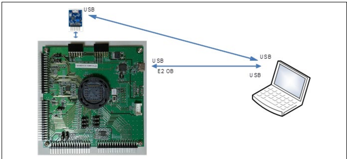
図 6-2 MCB RX26T と PC の接続
