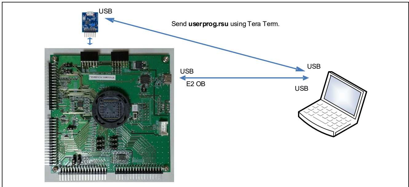
図 6-16 UART を使用したファームウェアアップデートを行うときの MCB RX26T と PC の接続
