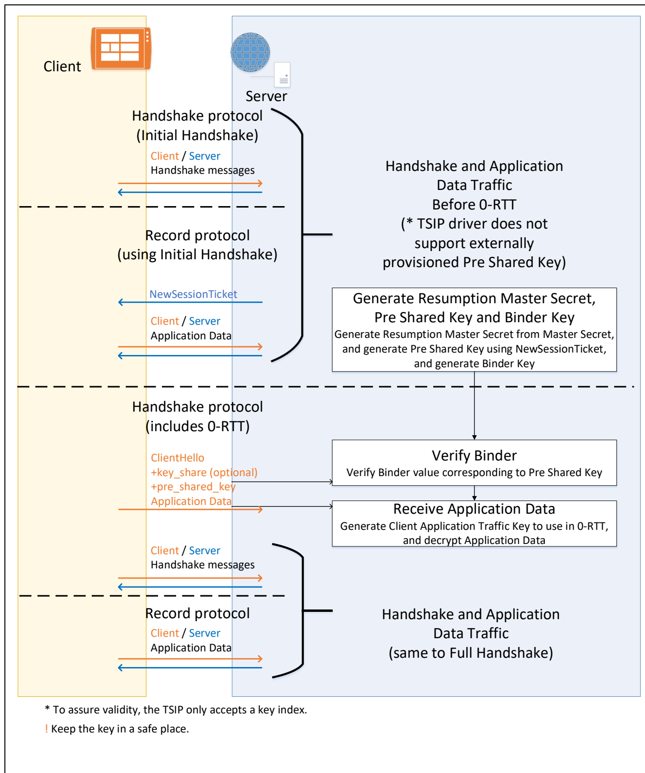
図 3-44 TLS1.3 サーバ機能 0-RTT の実施方法
