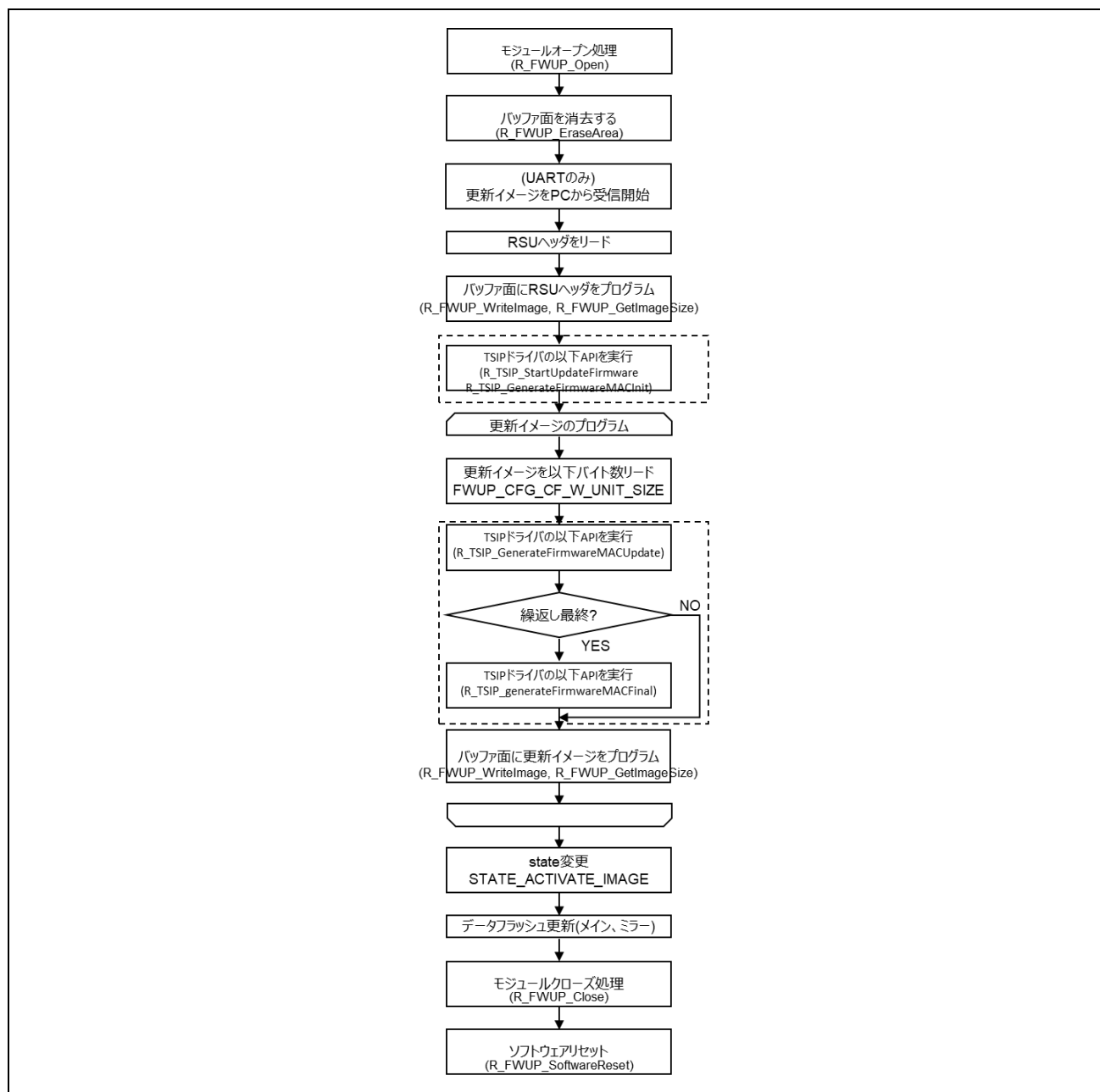
図 6-43 ファームアップデートフロー
