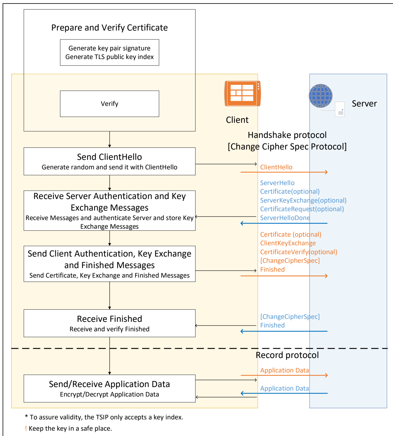
図 3-8 TLS1.2 クライアント機能の実施方法
