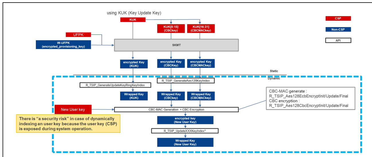
図 7-1 Encrypted Key の動的な生成方法
