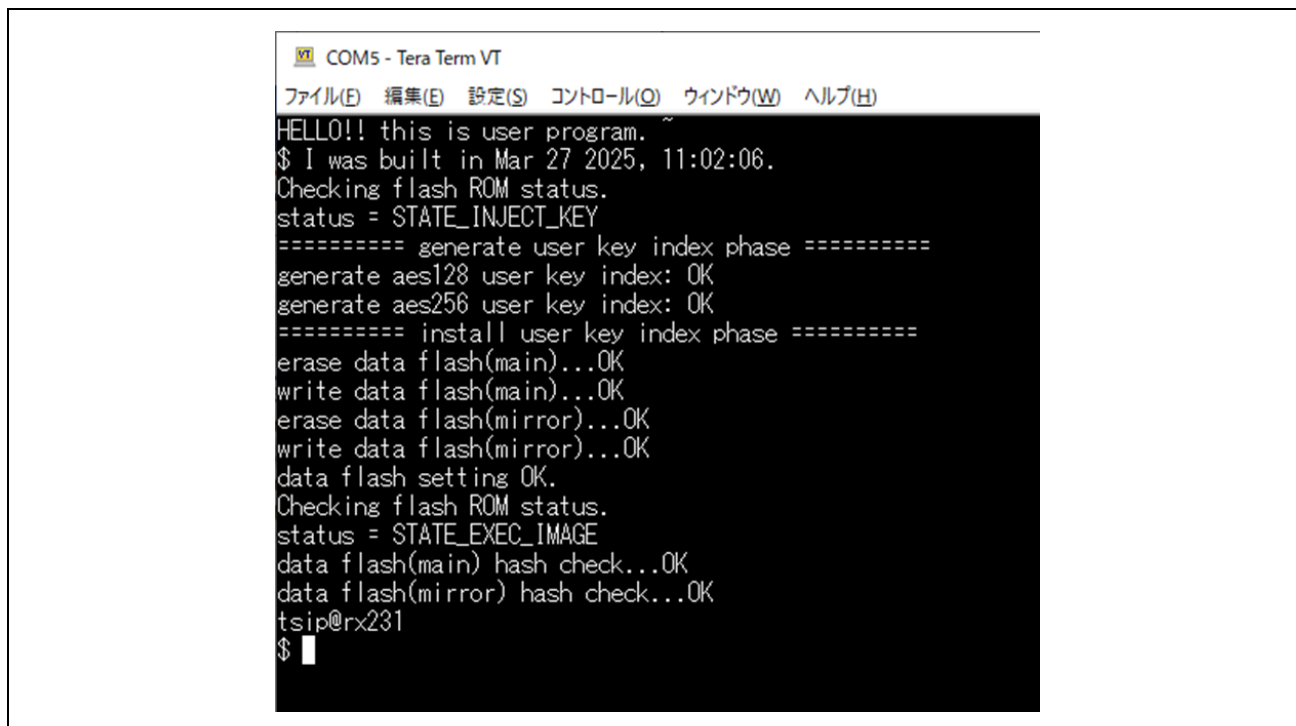
図 6-11 Tera Term 表示(RSK RX231 初回起動時)
