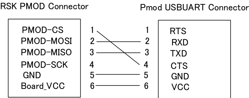
図 6-35 RX RSK と Pmod USBUART の接続図
