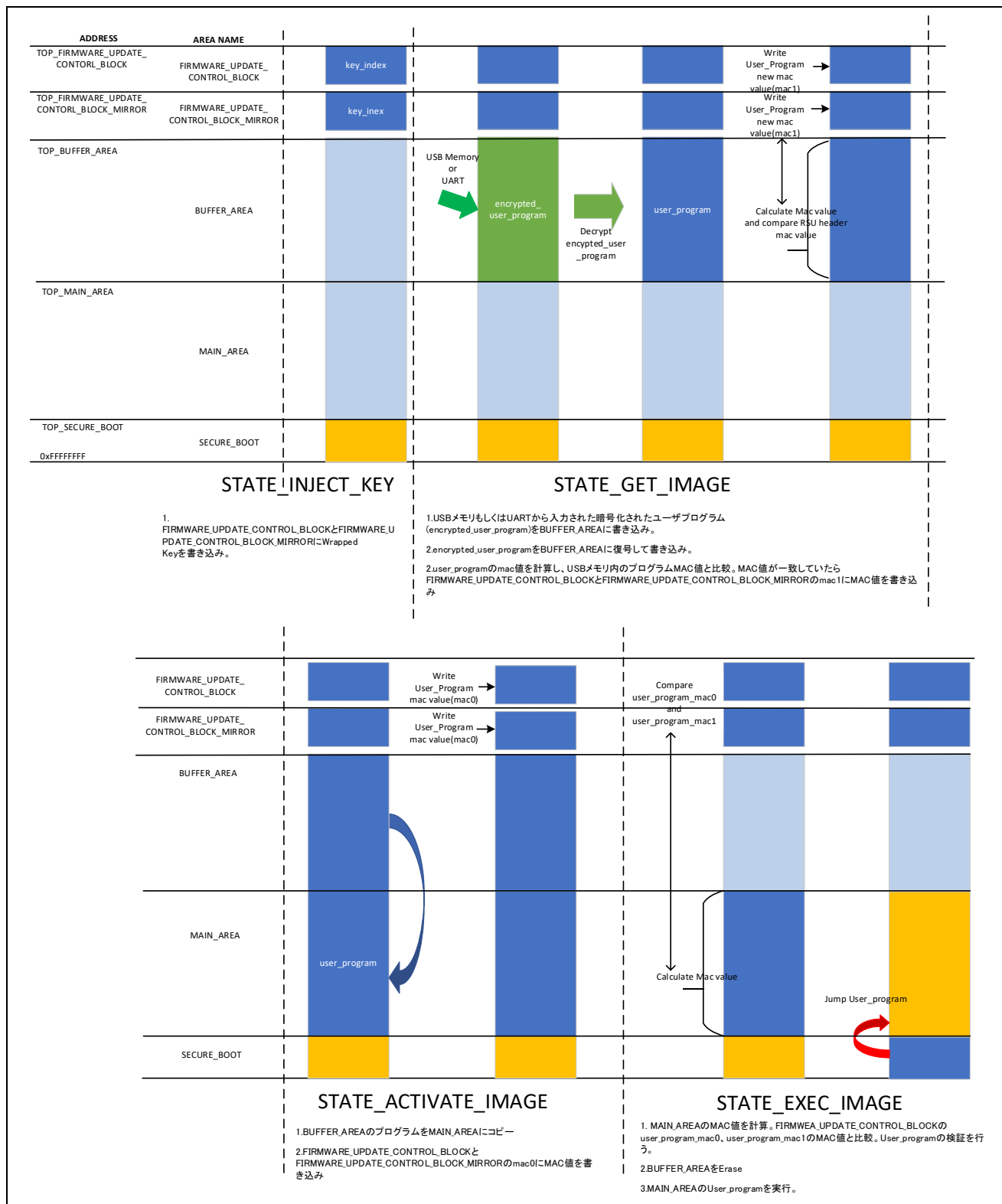
図 6-41 セキュアブート 各 state の内蔵 Flash メモリ状態(Dual Bank 非搭載デバイス)
