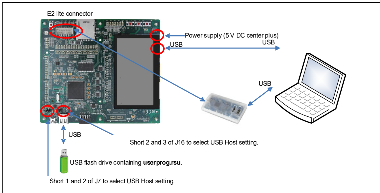
図 6-19 USB を使用したファームアップデートを行うときの RSK RX65N-2MB と PC の接続
