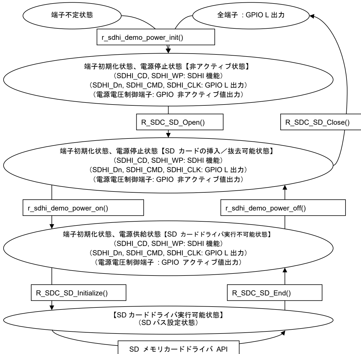
図 5-1 状態遷移図
