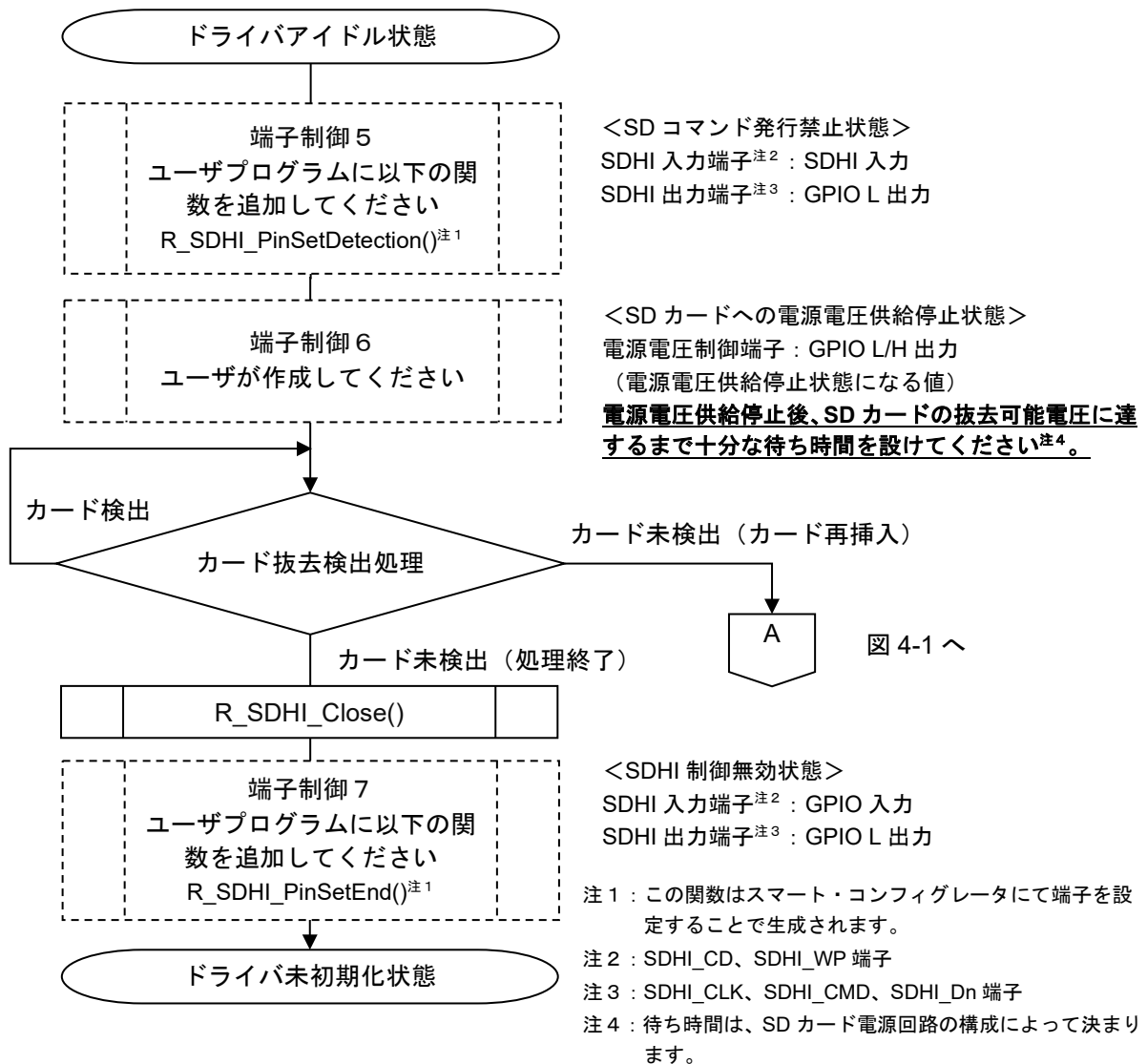
図 4-2 SD カードの抜去と電源停止タイミング
