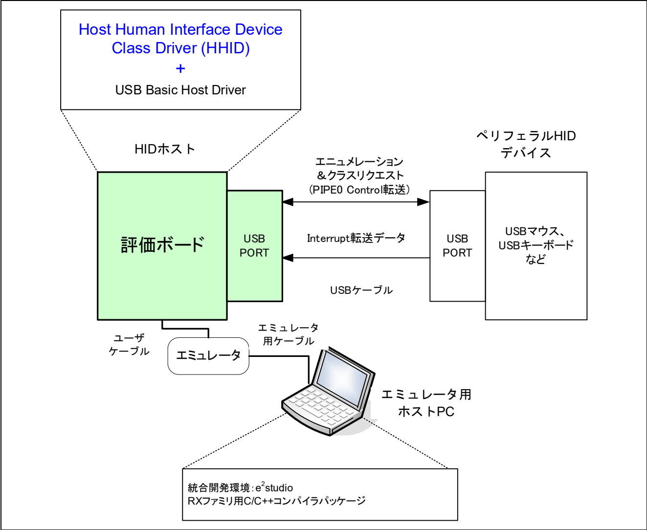
Figure 3-1 動作環境例
