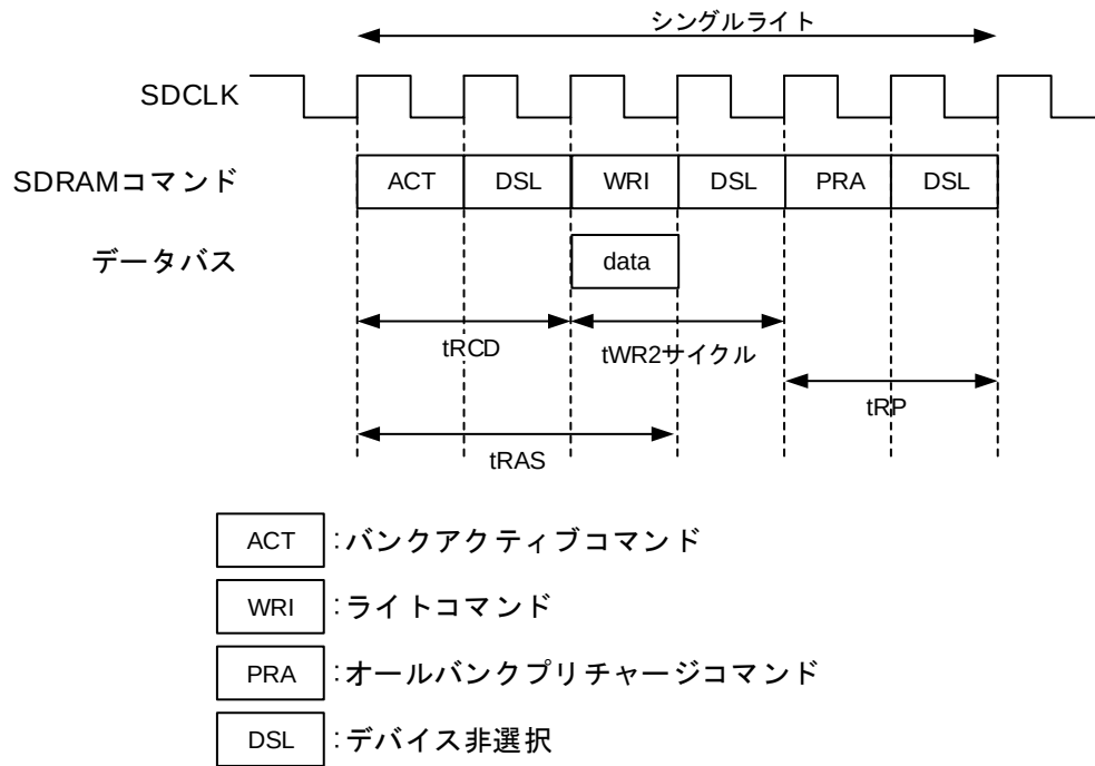
図 6.5 ライトタイミング(表 6.4 で示した SDRAMC 設定時)
