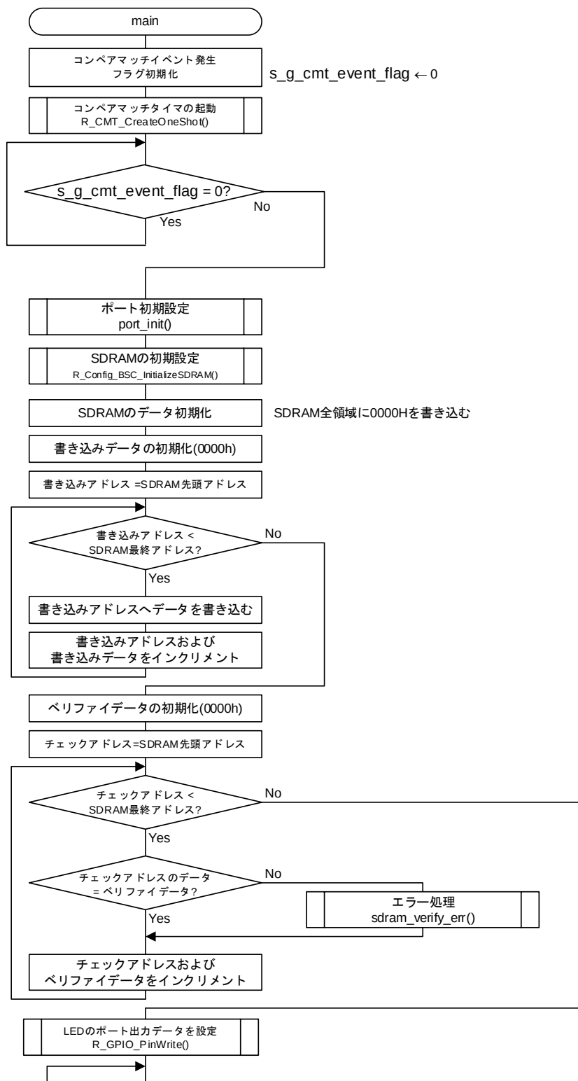
図 6.16 スマート・コンフィグレータを使用しているサンプルコードのメイン処理
