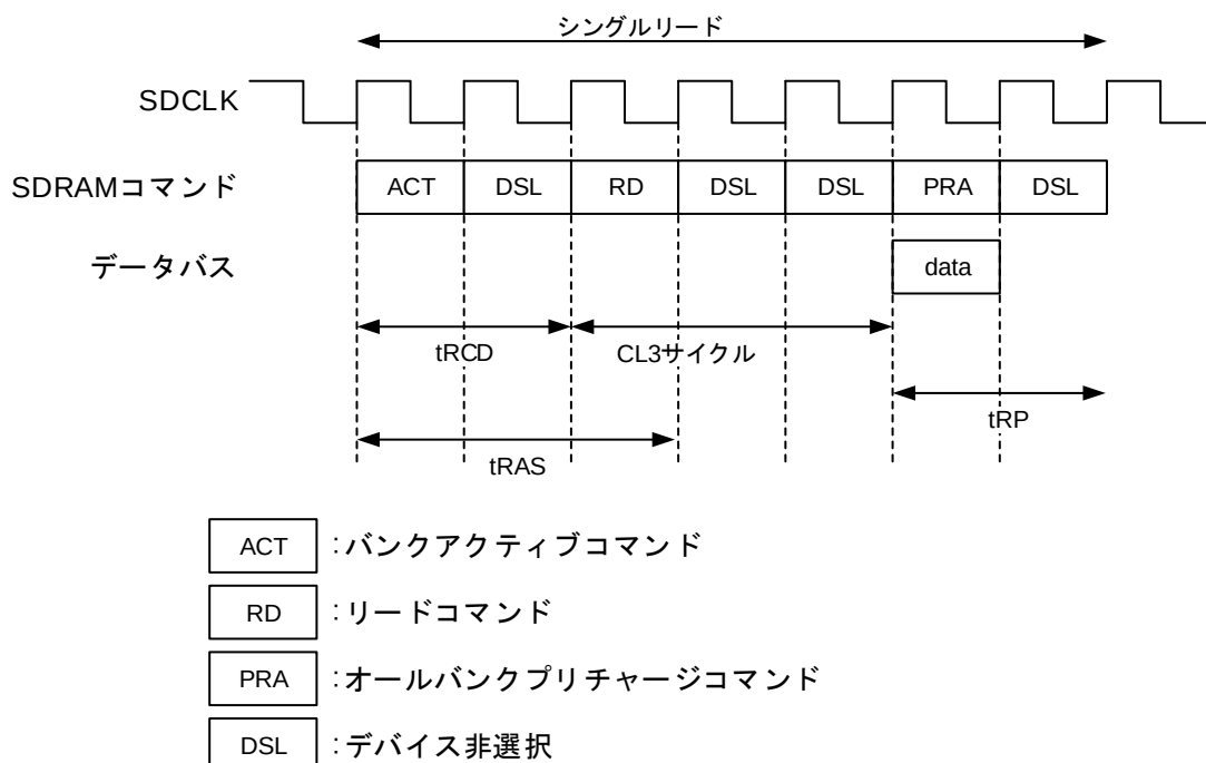
図 6.4 リードタイミング(表 6.4 で示した SDRAMC 設定時)
