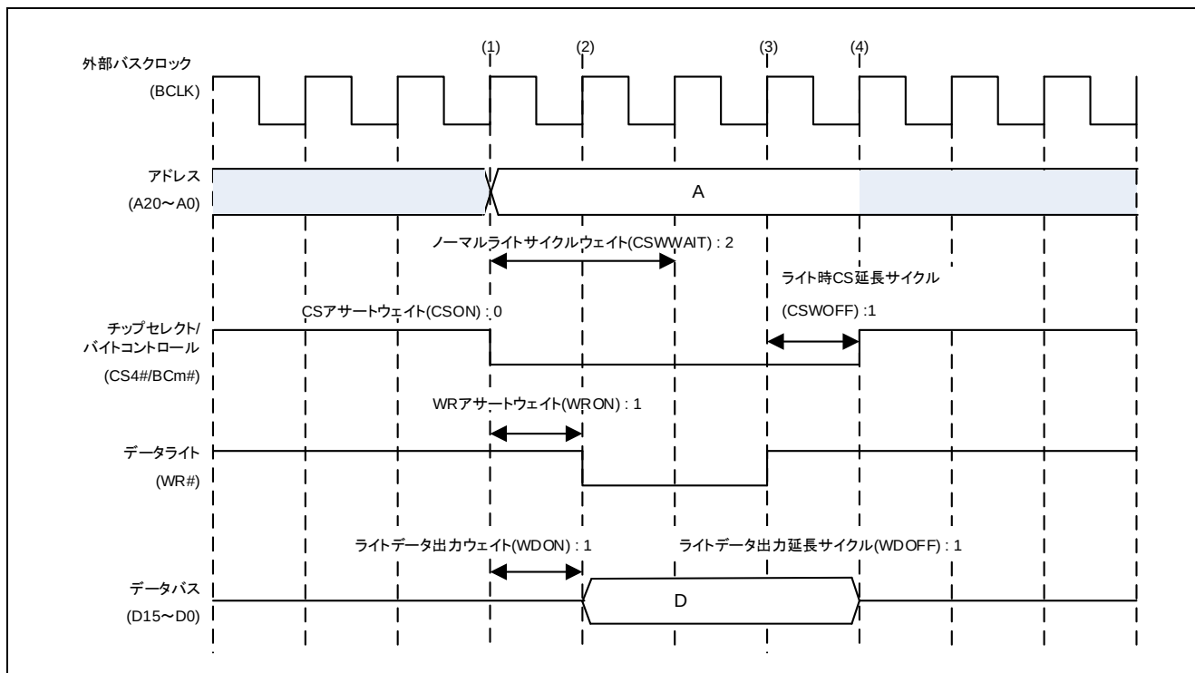
図 5.2 バスタイミング（ノーマルライト、1 ライトストローブモード）（m=0~1）
