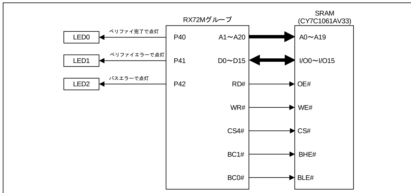
図 3.1 ブロック図
