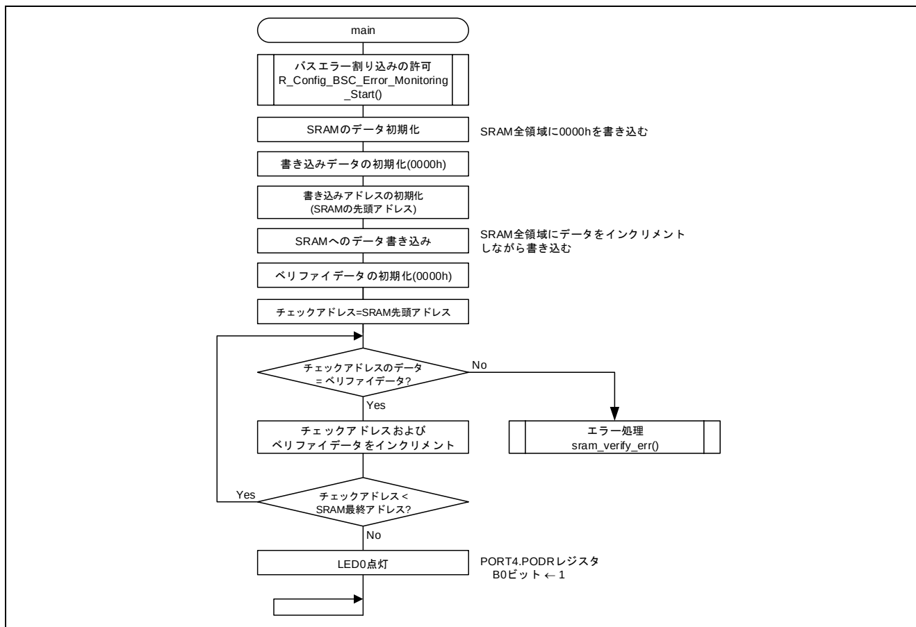
図 5.4 メイン処理
