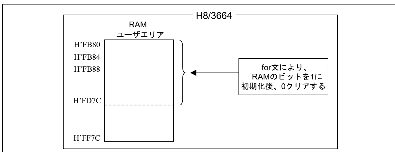
図 1 for 文による RAM クリア図
