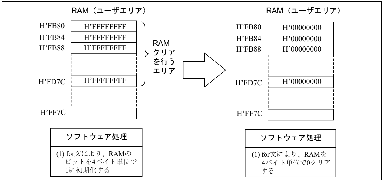
図 2 動作説明
