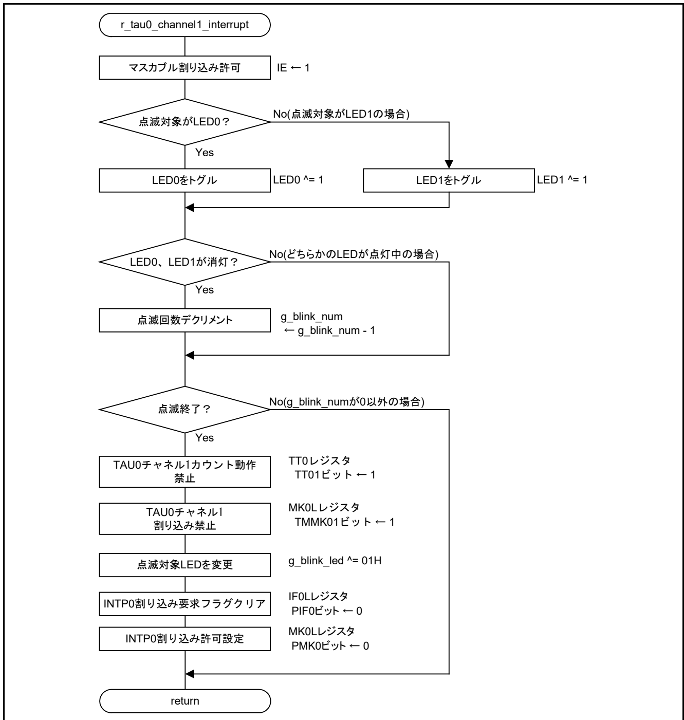
図 6.18 TAU01 割り込みハンドラ
