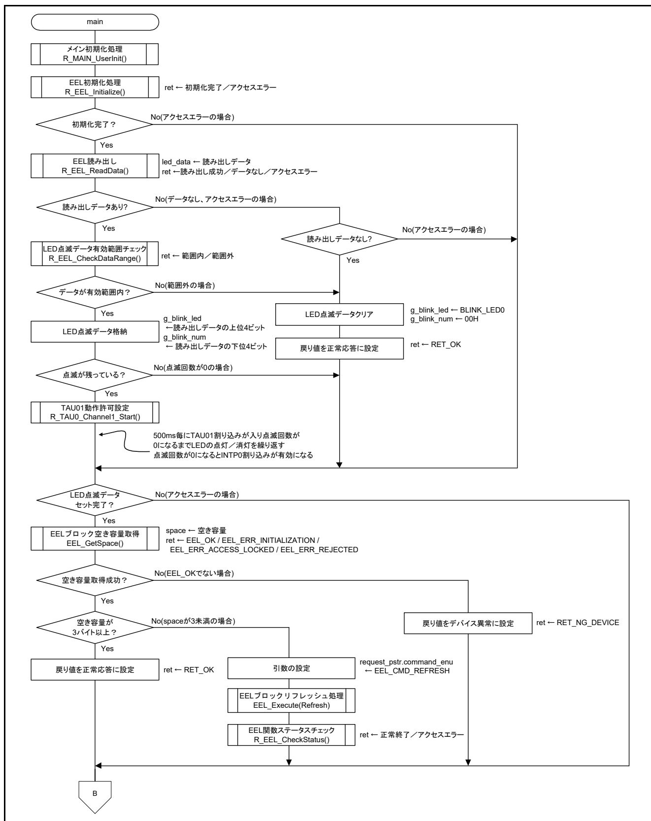
図 6.10 メイン処理(1/2)
