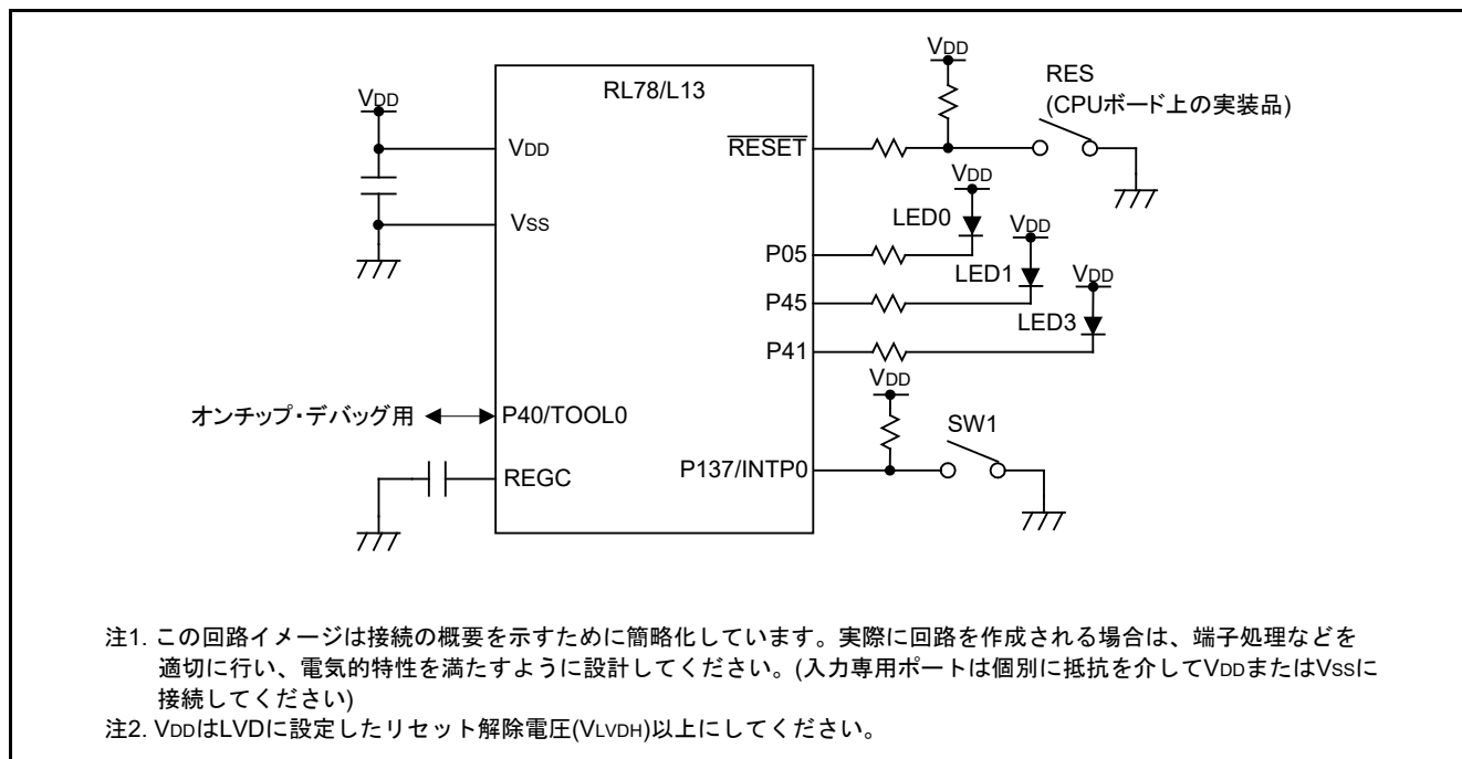
図5.1 接続例
