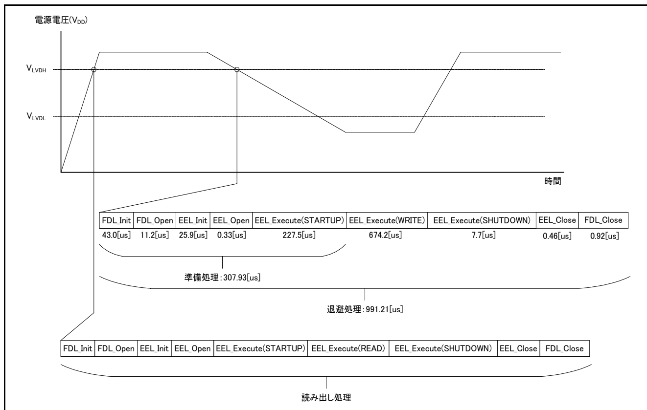
図2.4 データ退避処理（一括）
