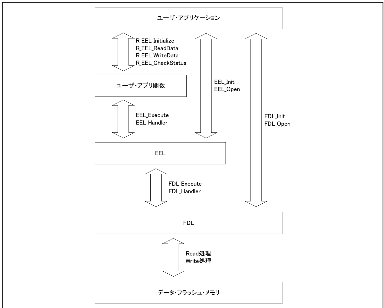
図2.2 アプリケーション全体像
