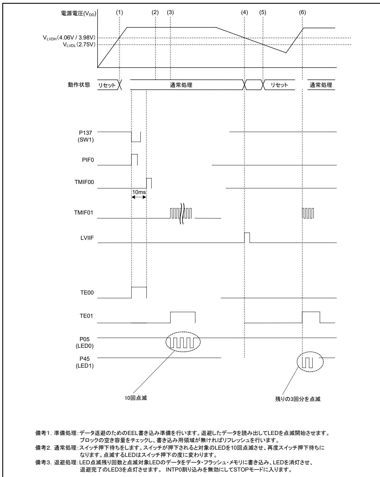
図6.1 タイミング図
