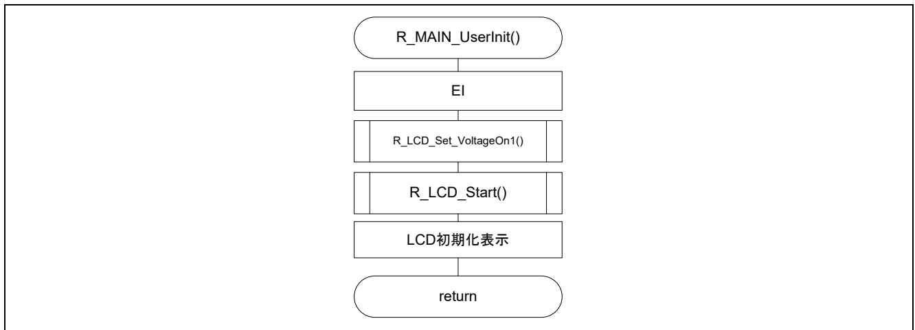
図 4.13 LCD 初期化表示設定
