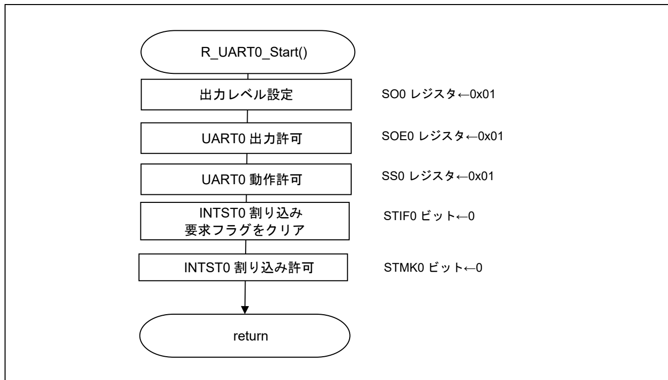
図 4.18 シリアル・アレイ・ユニット動作開始関数
