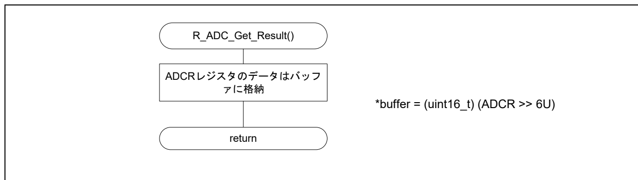
図 4.15 温度データ取得処理
