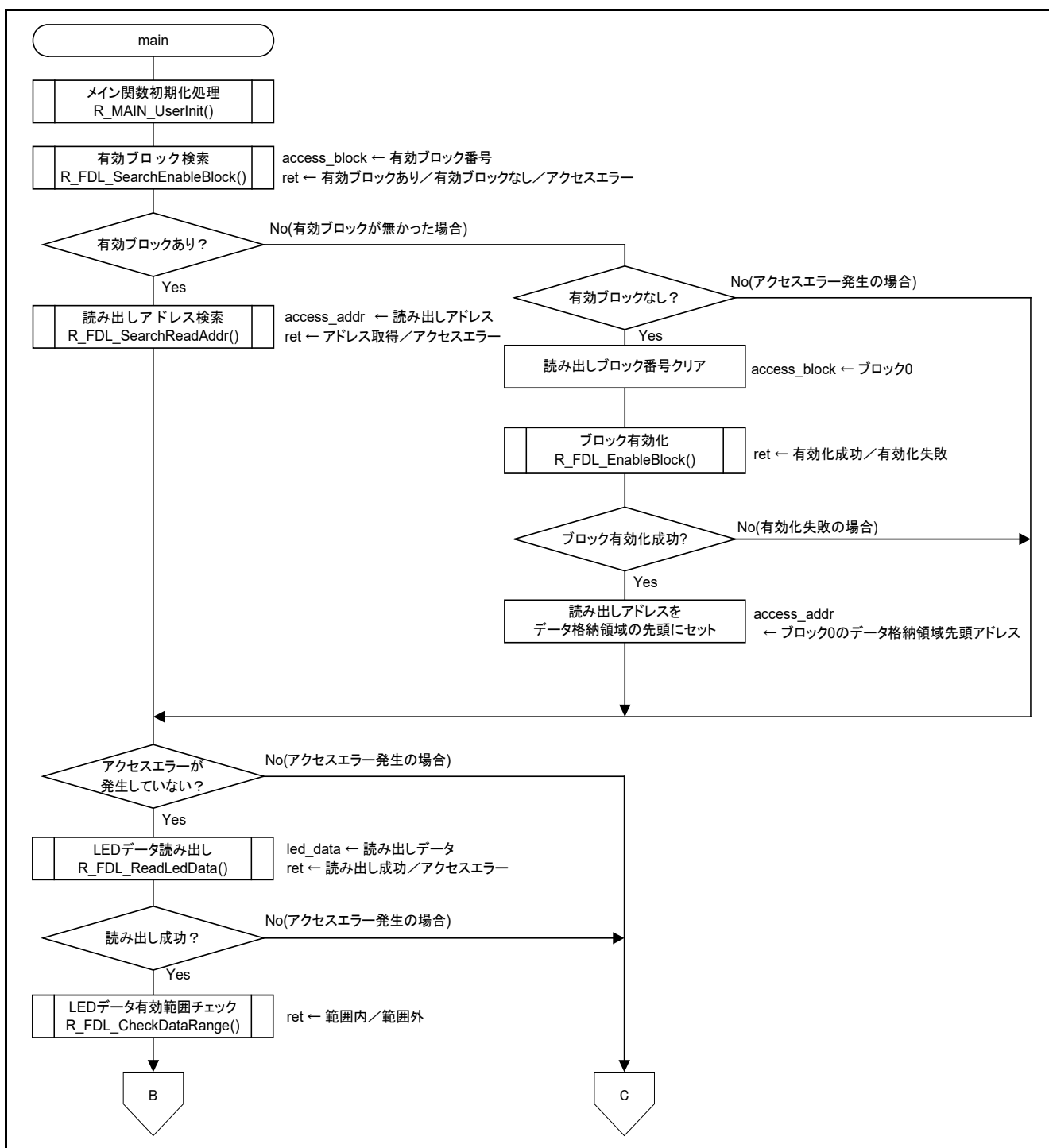
図 6.10 メイン処理(1/3)
