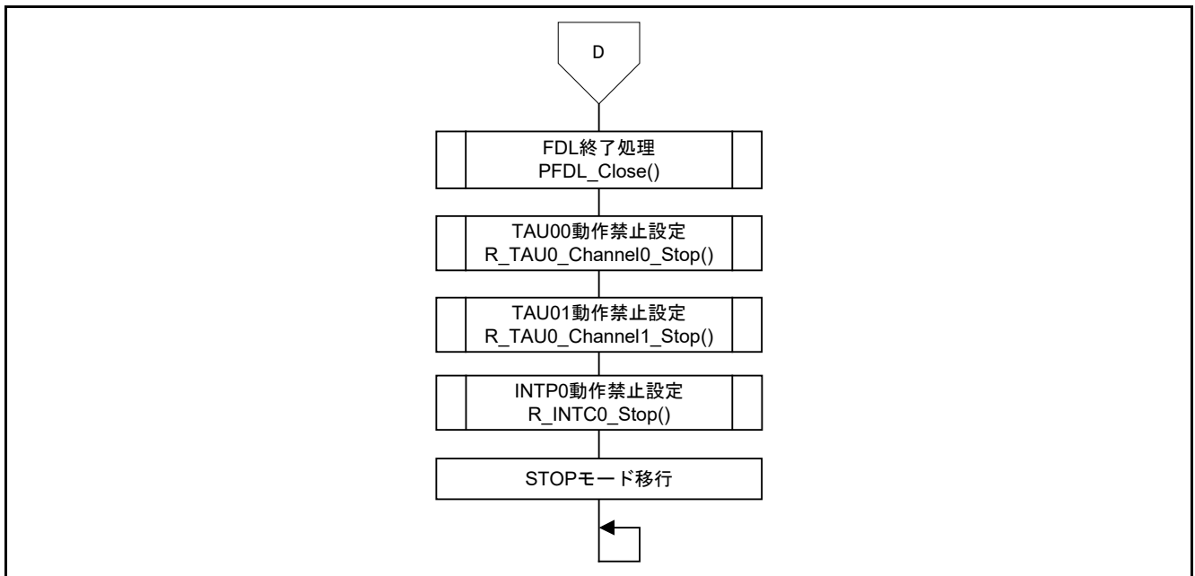
図 6.12 メイン処理(3/3)
