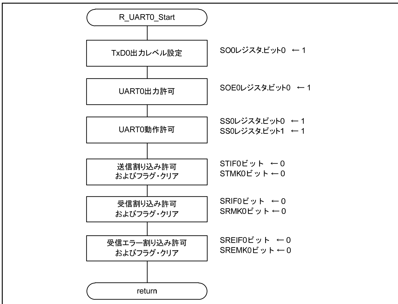
図 5.16 UART0 動作開始関数
