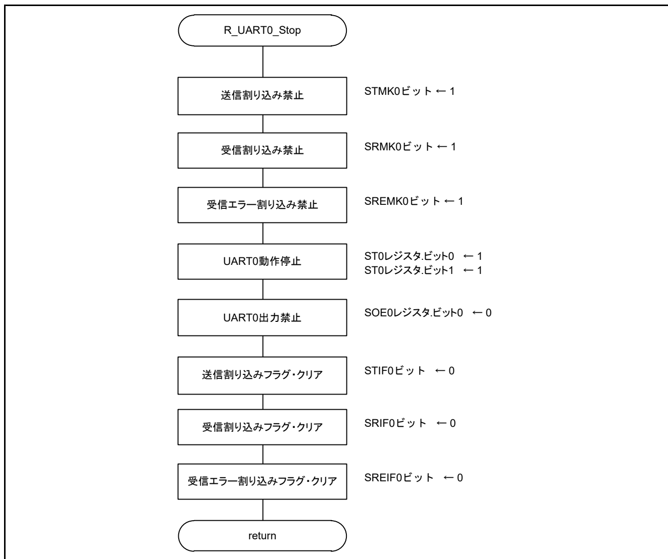
図 5.18 UART0 動作停止関数
