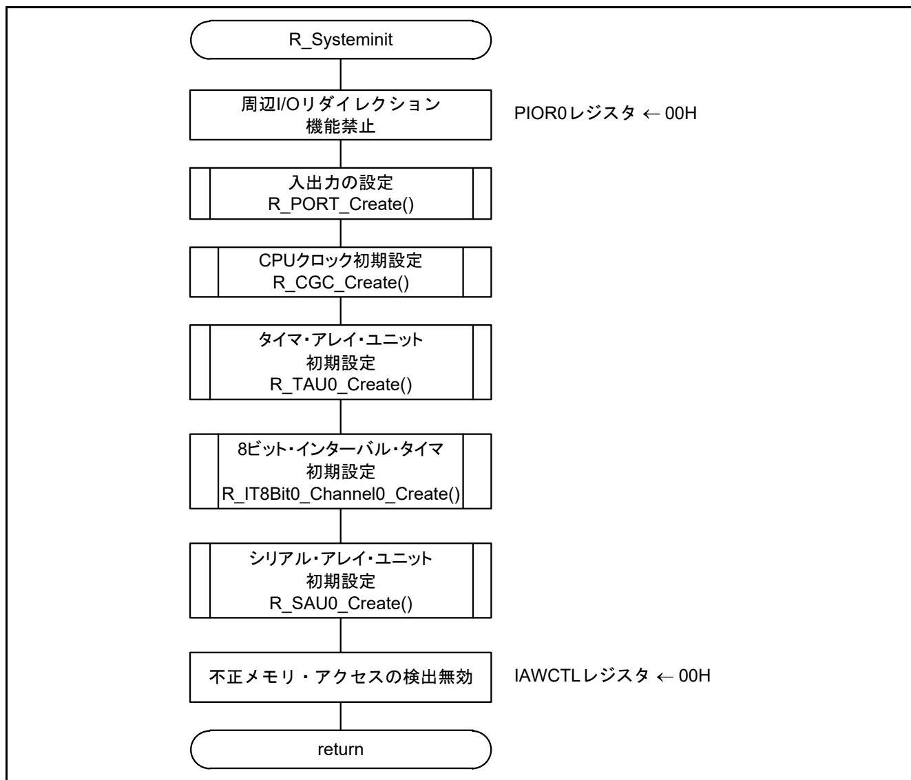
図 5.3 周辺機能初期設定関数
