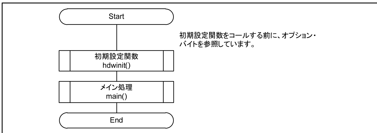
図 5.1 全体フロー
