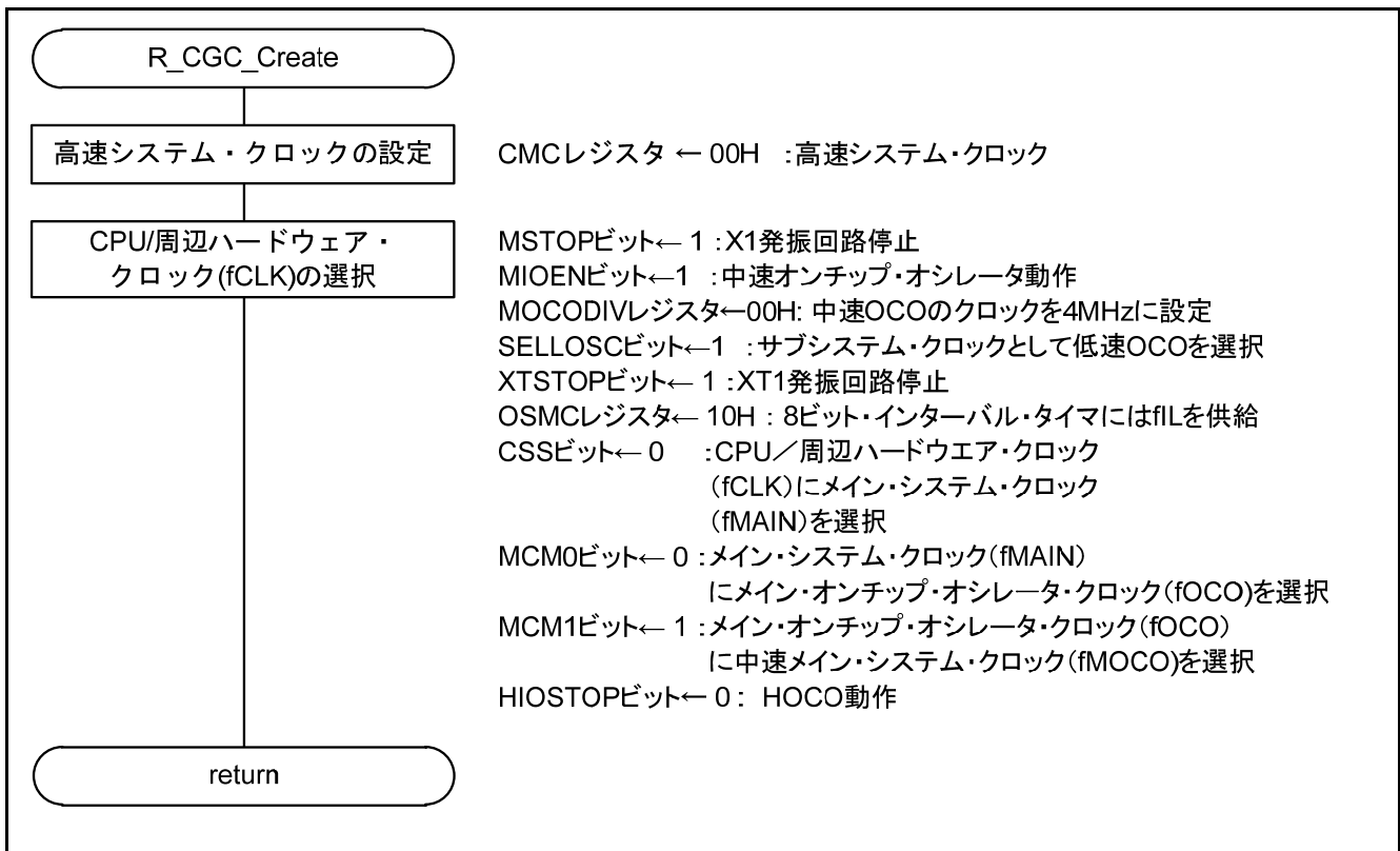
図 5.5 CPU クロック初期設定関数
