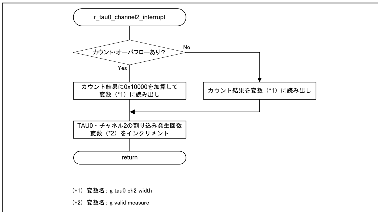
図 5.24 TAU チャンネル 02 カウント完了割り込み関数
