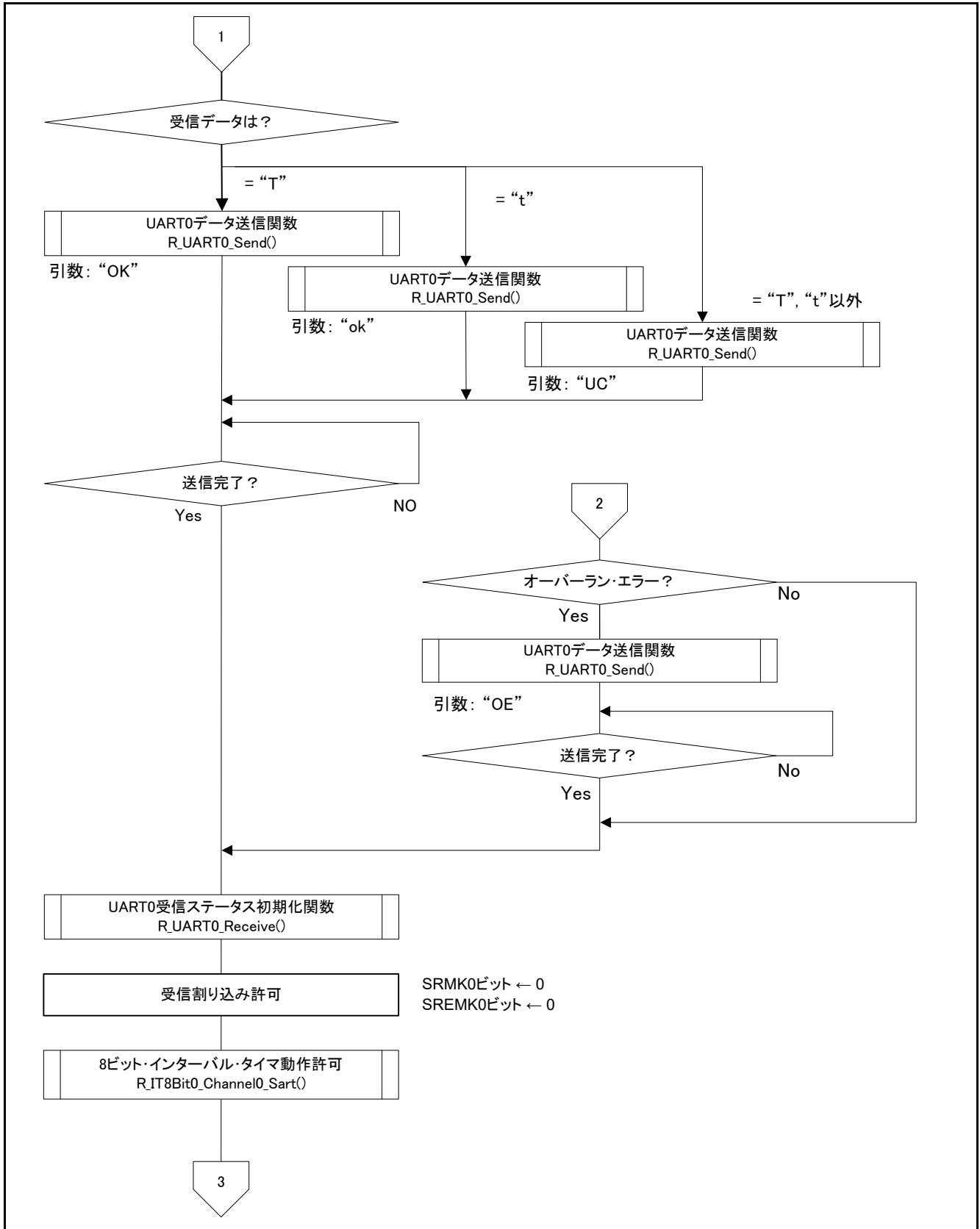
図 5.13 メイン処理 (2/2)
