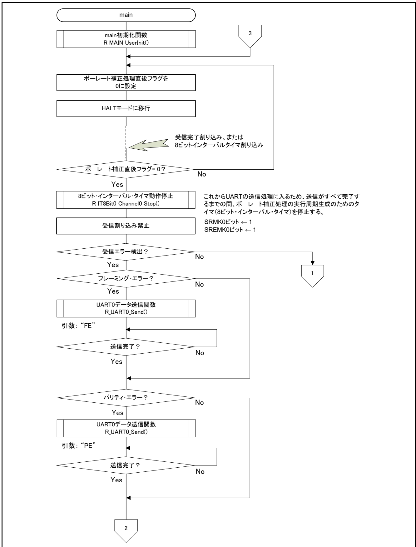
図 5.12 メイン関数 (1/2)
