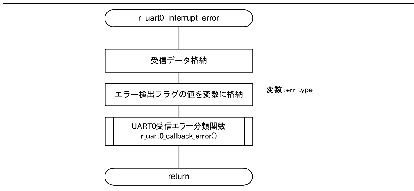
図 5.20 UART0 受信エラー割り込み関数
