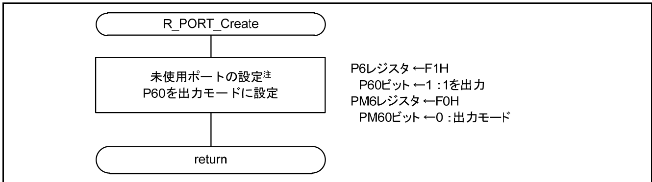
図 5.4 入出力ポートの設定
