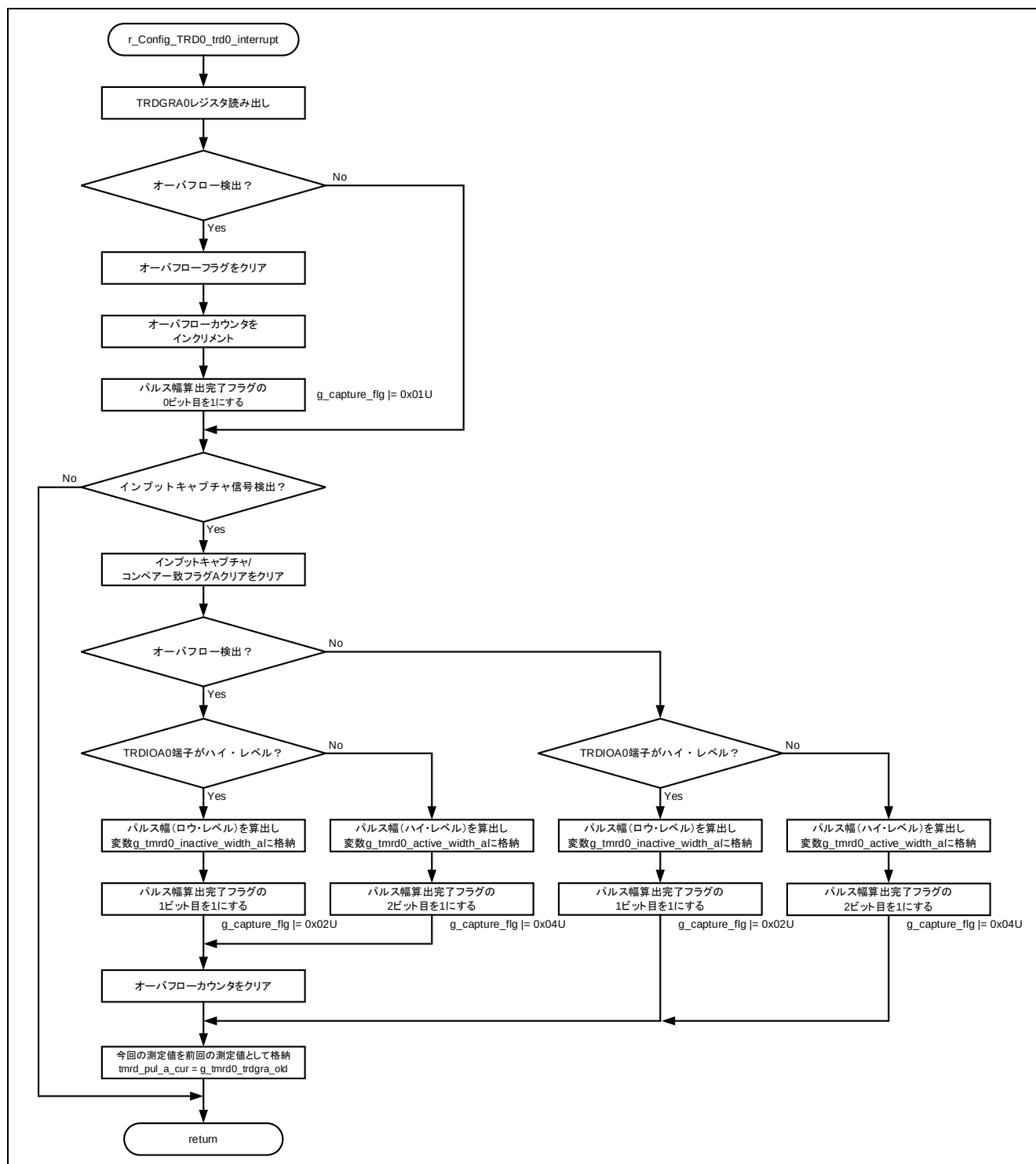
図 4-7 r_Config_TRD0_trd0_interrupt 関数
