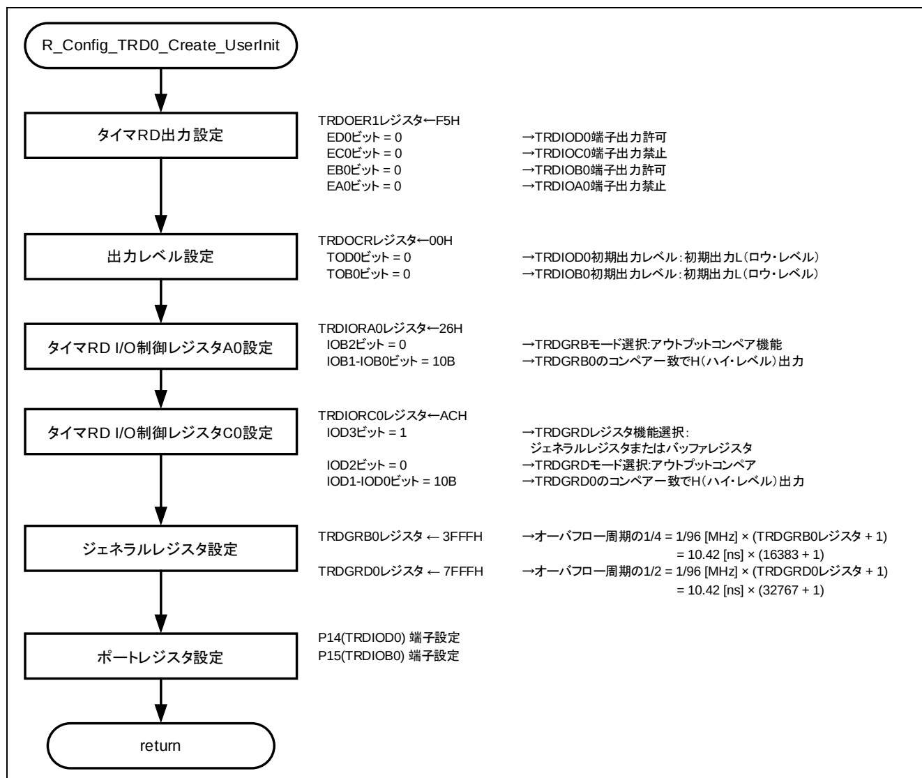
図 4-6 R_Config_TRD0_Create_UserInit 関数
