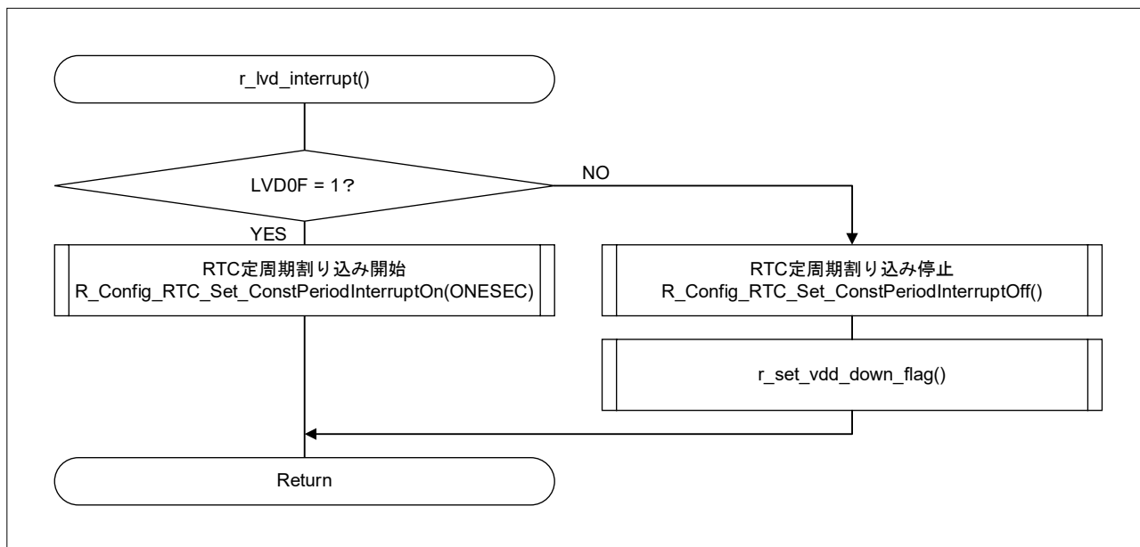
図 4-16 LVD0 割り込み処理
