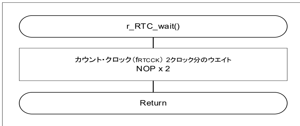
図 4-8 RTC 動作開始時 HALT/STOP モード移行ウェイト処理
