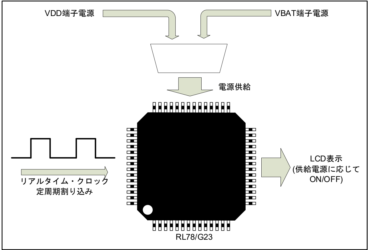
図 1-1 VBAT の動作概要
