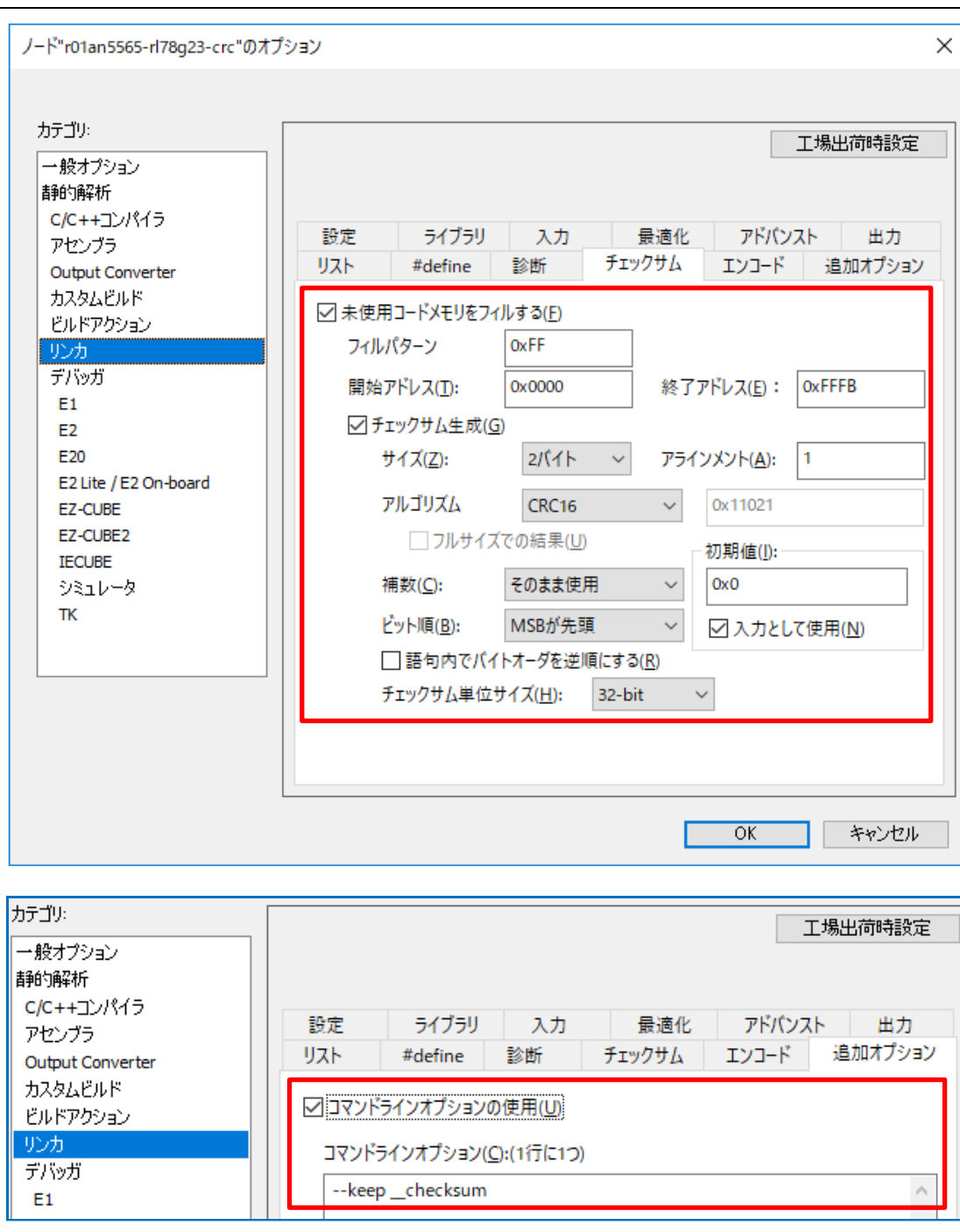
図 4 - 5 オブジェクト・コンバート・オプション設定 (IAR のオプション画面)
