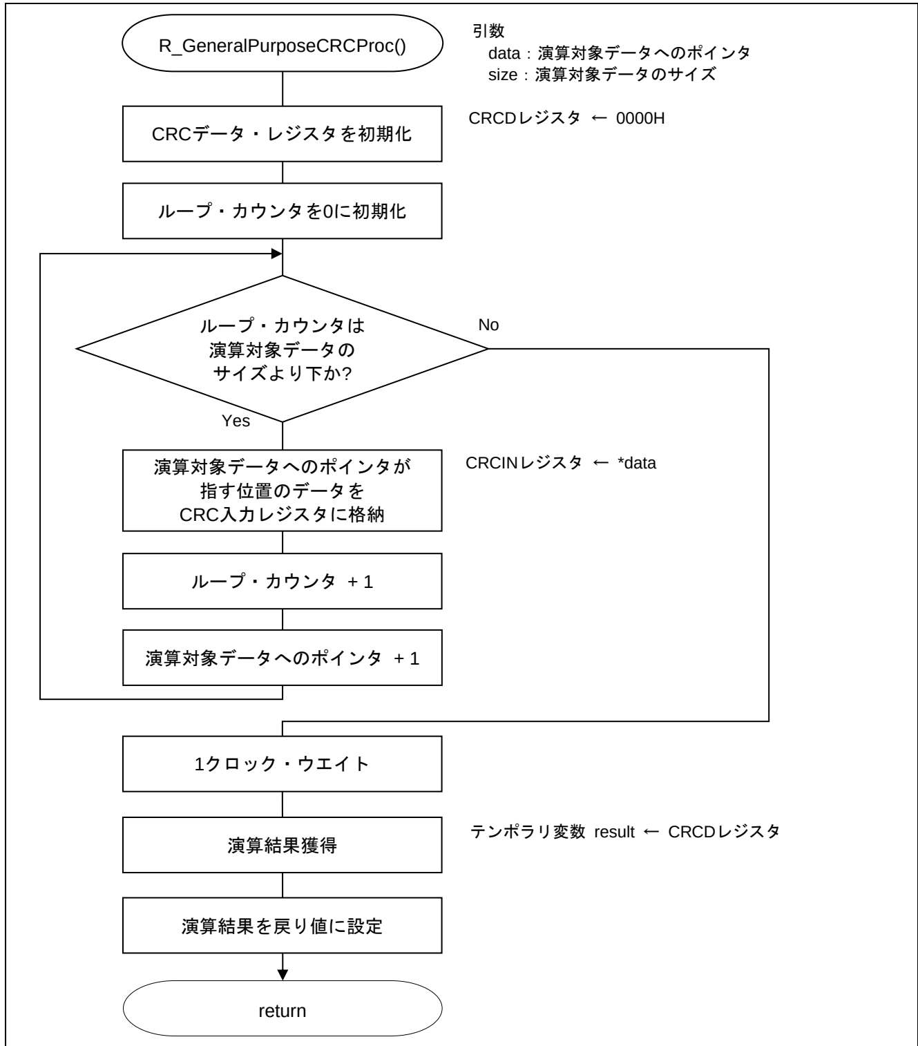
図 4 - 13 汎用 CRC 演算処理
