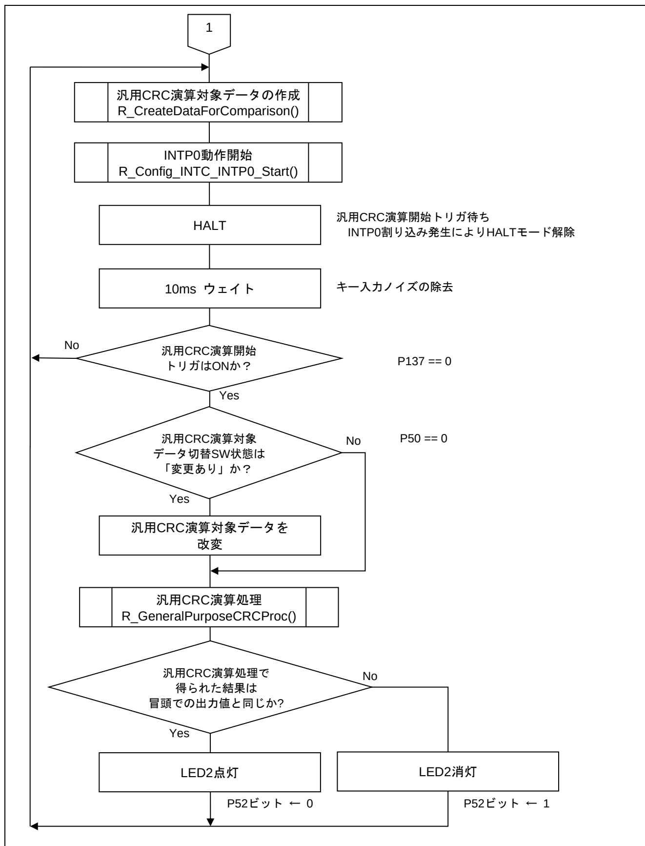
図 4 - 2 メイン処理 (2/2)
