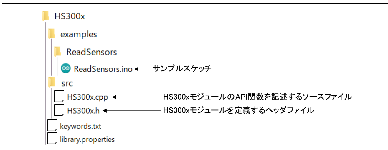
図 4-1 サンプルコードのファイル構成
