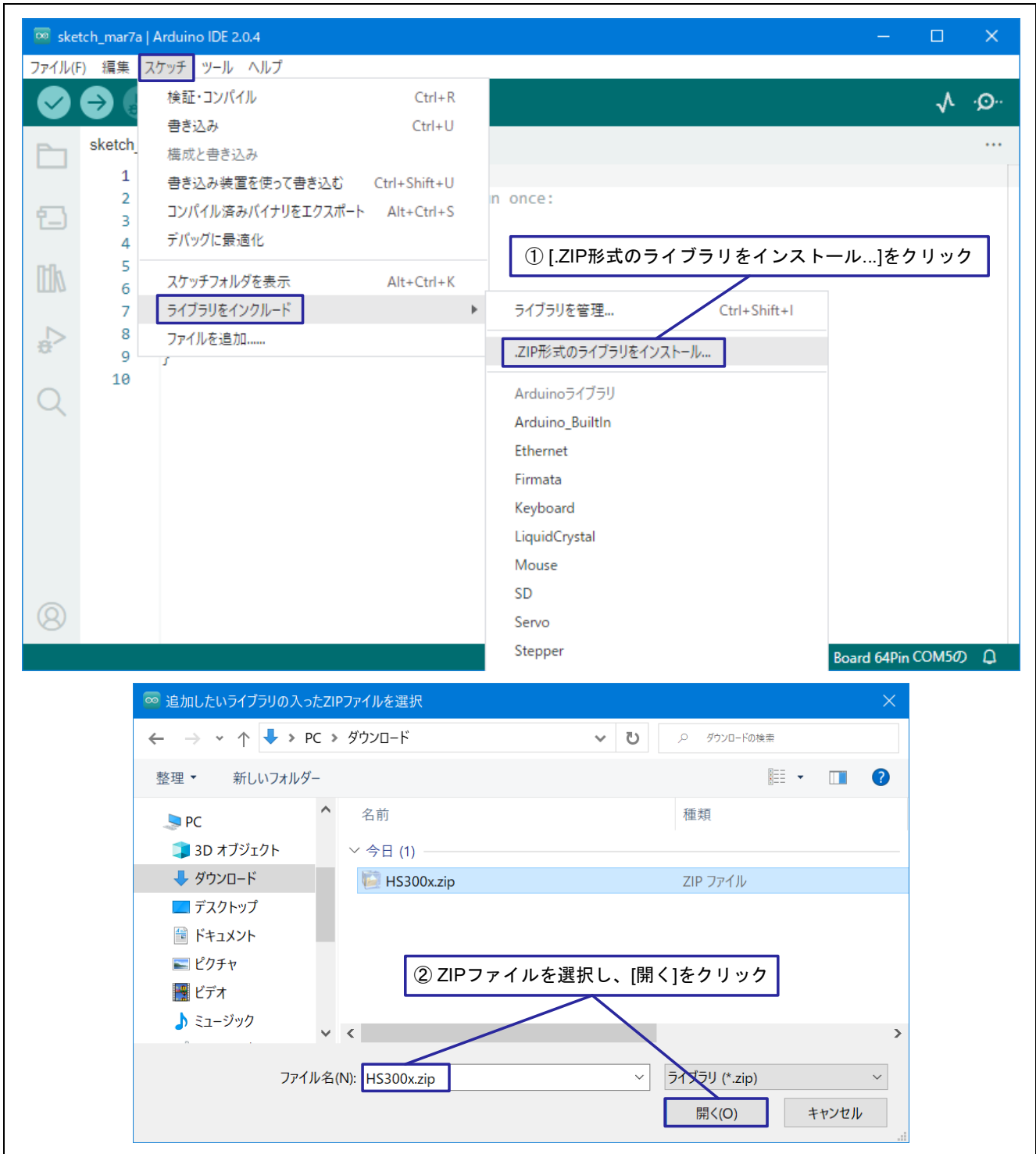
図 4-2 HS300x モジュールのインクルード
