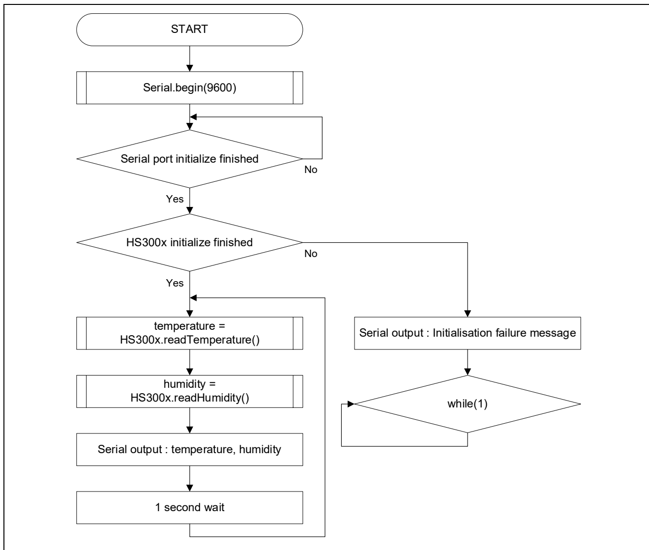
図 4-7 サンプルスケッチのフロー
