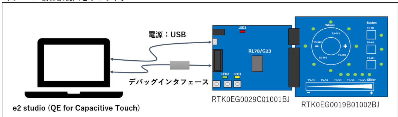
図 2.1 機器接続図
