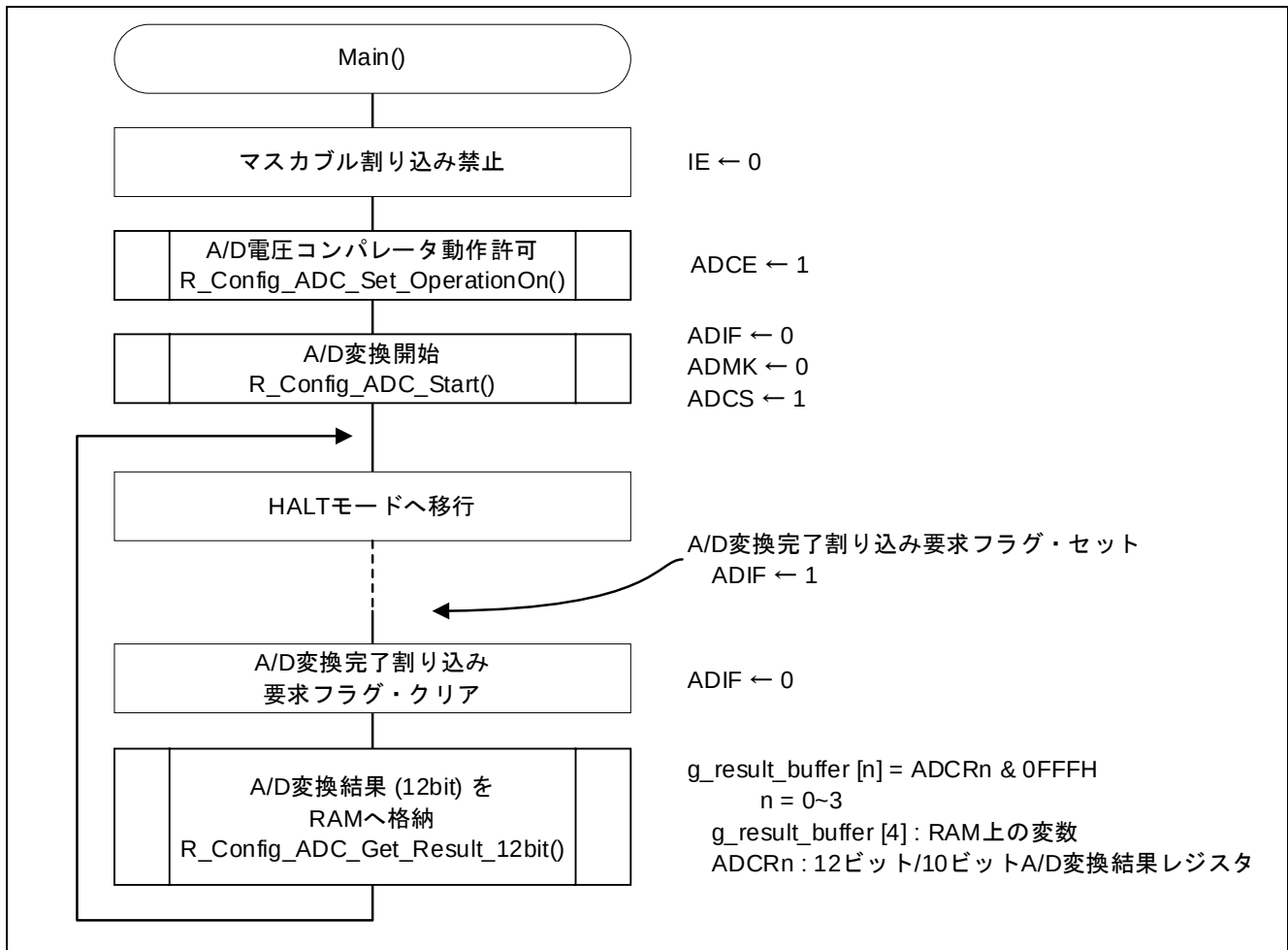
図 4 - 1 メイン処理
