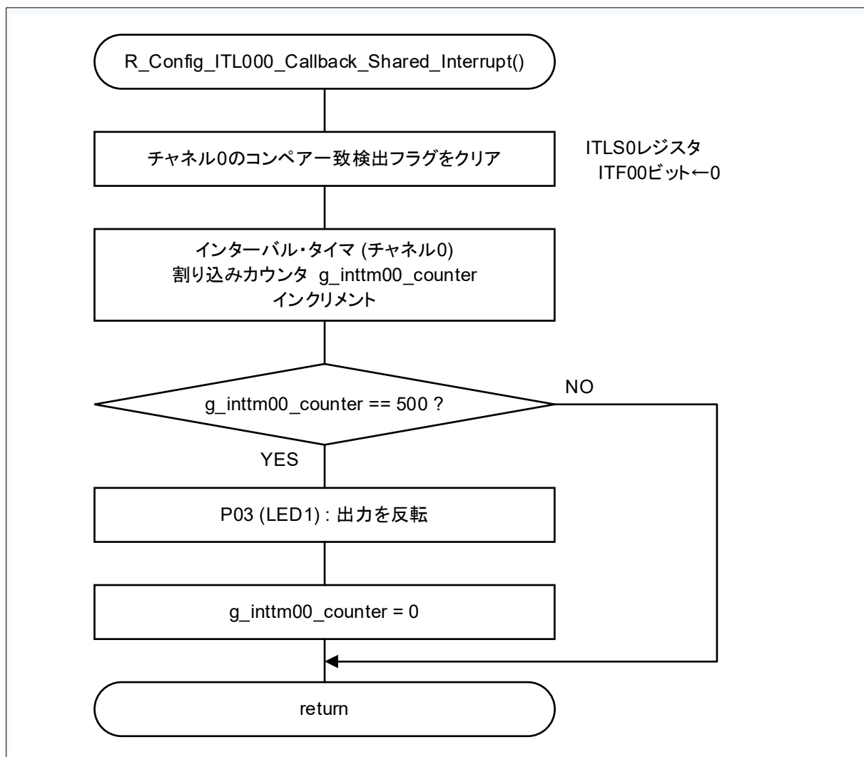
図 4-3 インターバル・タイマ・チャンネル0 割り込み処理
