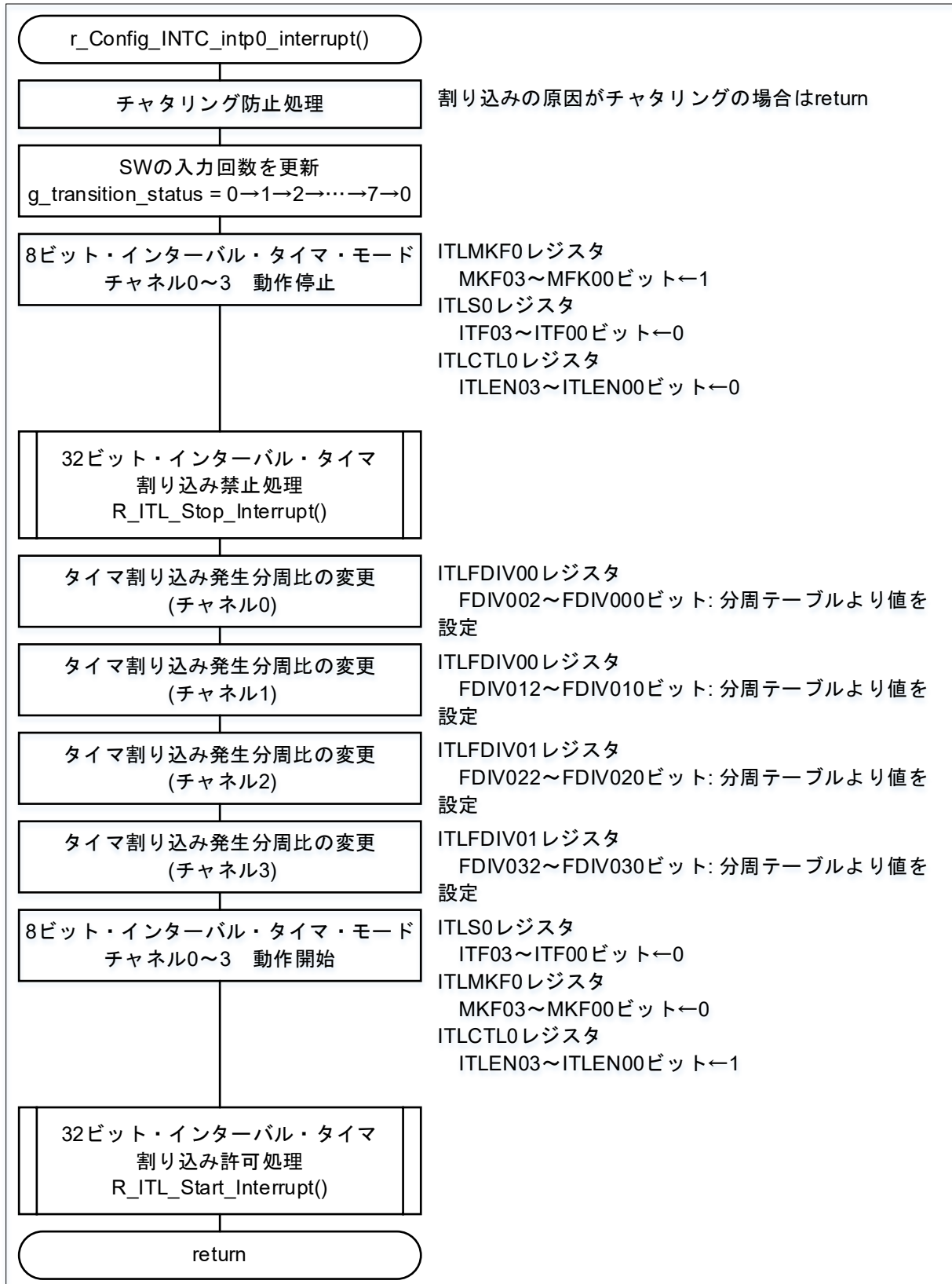
図 4-7 INTP0 割り込み処理
