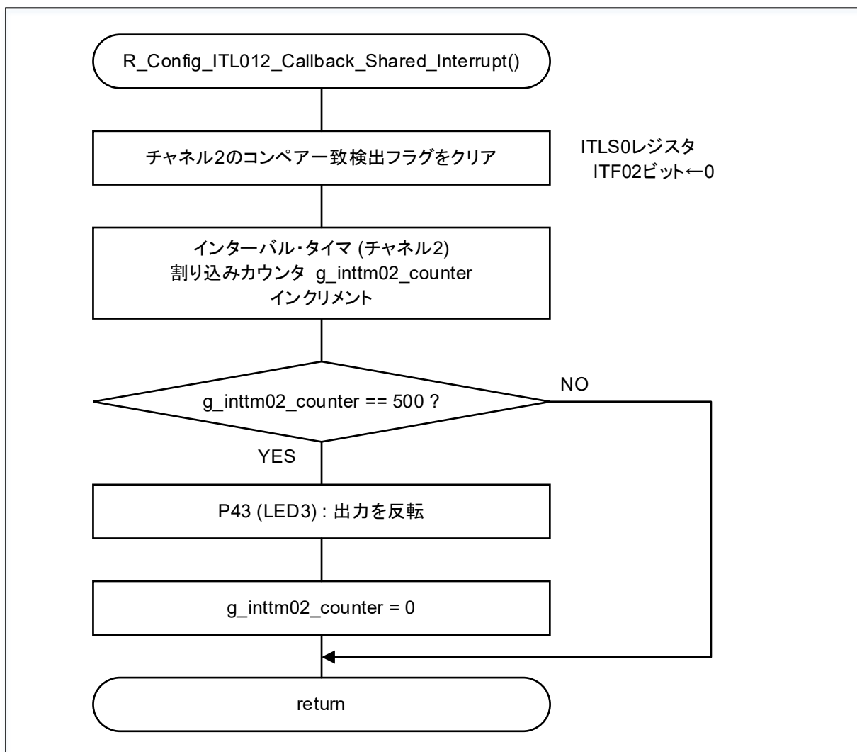
図 4-5 インターバル・タイマ・チャンネル 2 割り込み処理
