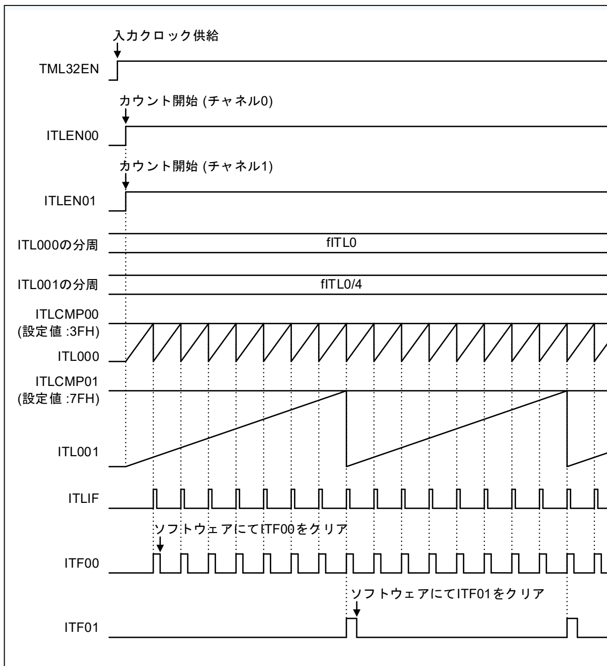
図 1-2 タイマ割り込み動作概要 (8ビット・カウンタ・モード)
