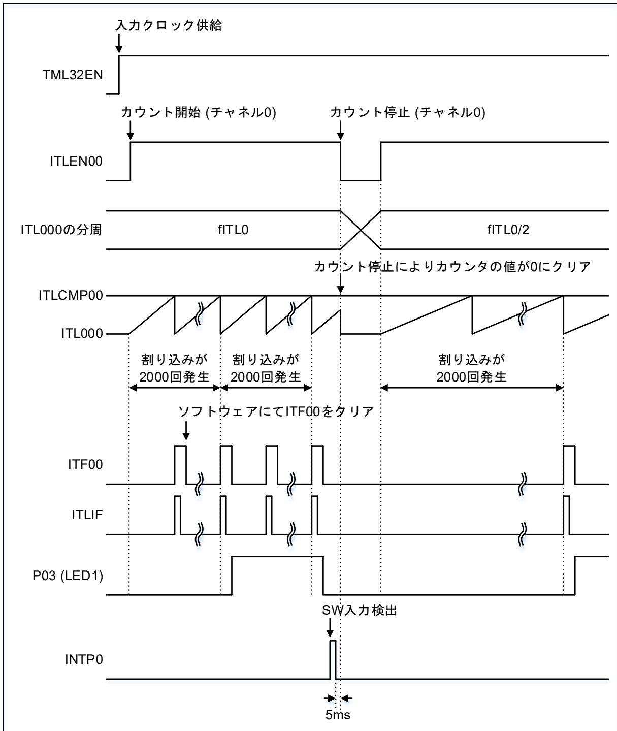
図 1-1 タイマと割り込みの動作概要 (8 ビット・カウンタ・モード チャンネル 0 動作例)
