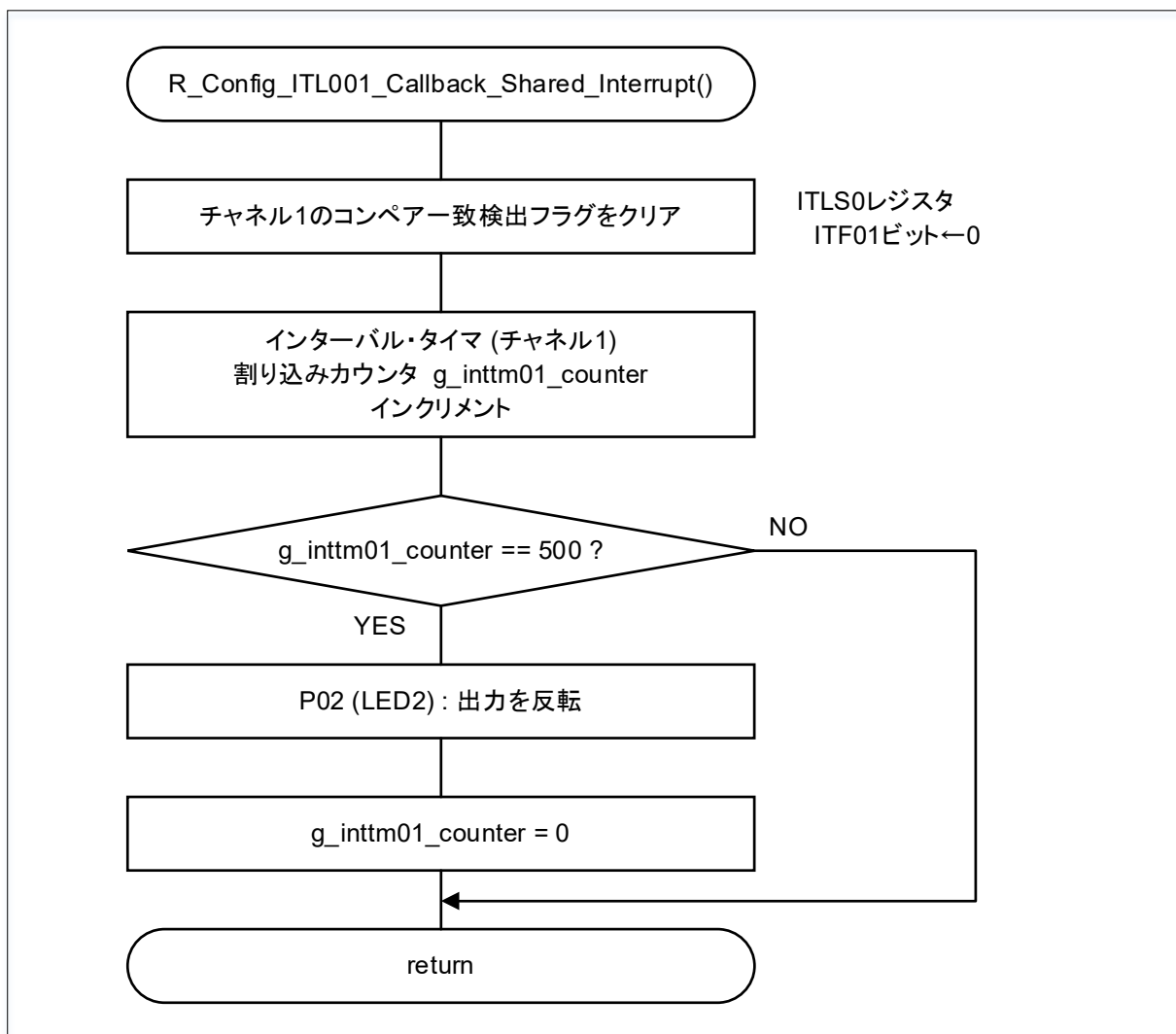
図 4-4 インターバル・タイマ・チャンネル1 割り込み処理
