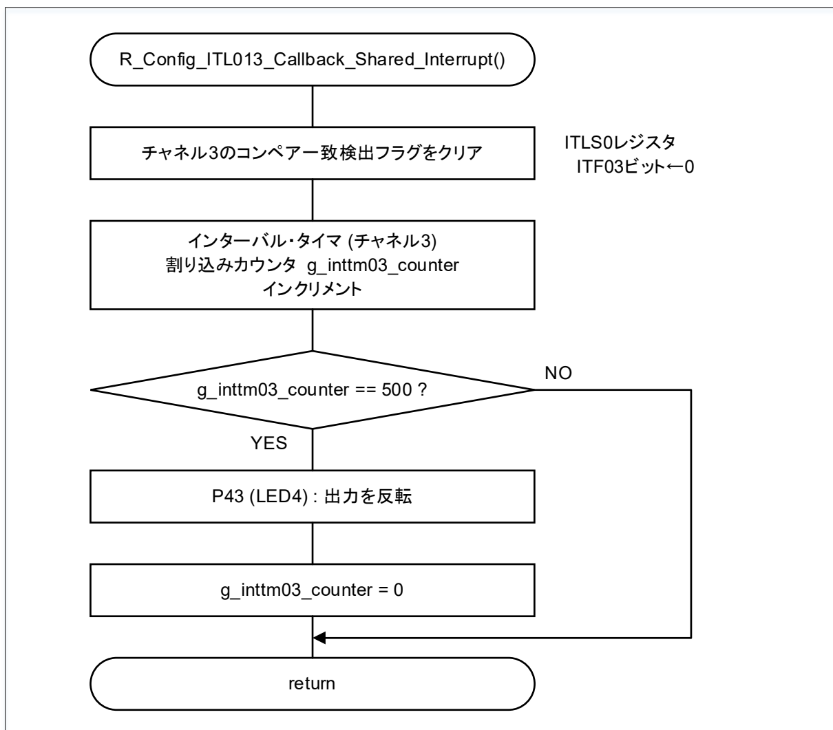
図 4-6 インターバル・タイマ・チャンネル3 割り込み処理
