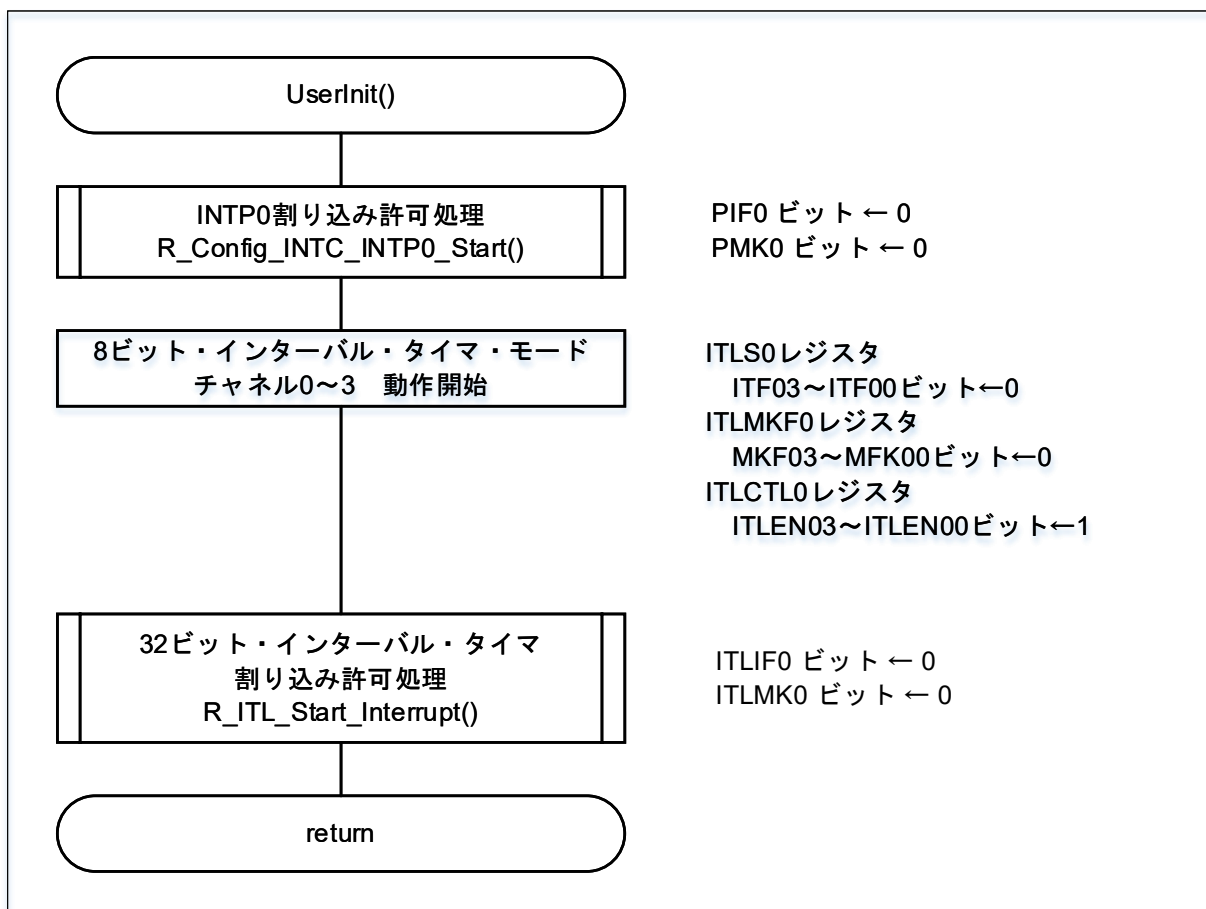
図 4-2 メイン・ユーザー初期設定
