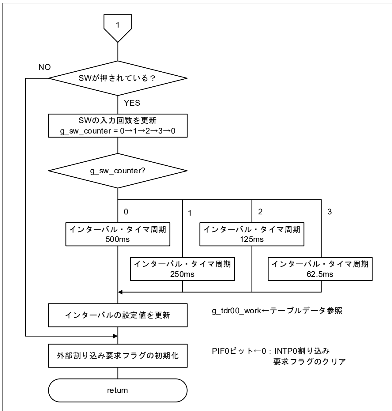
図 4-4 外部割り込み処理 (2/2)
