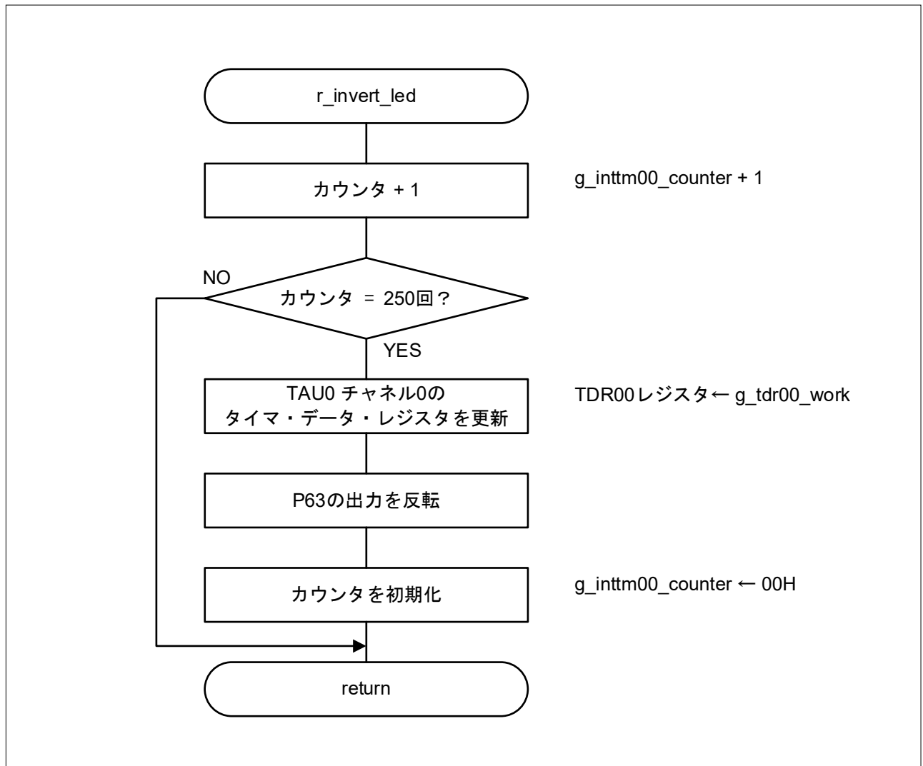
図 4-5 LED 点灯／消灯処理
