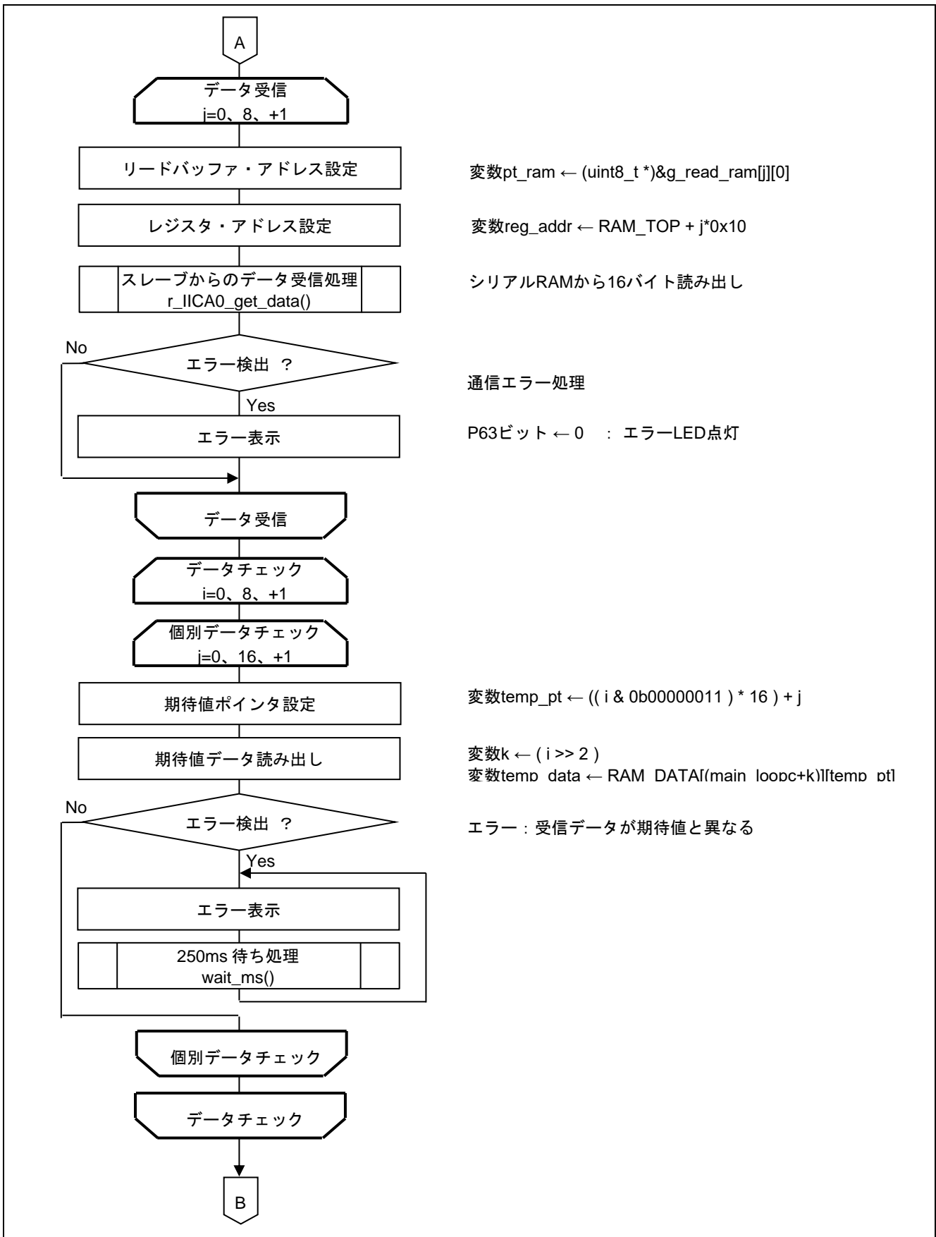
図 5.2 メイン処理 (2/3)
