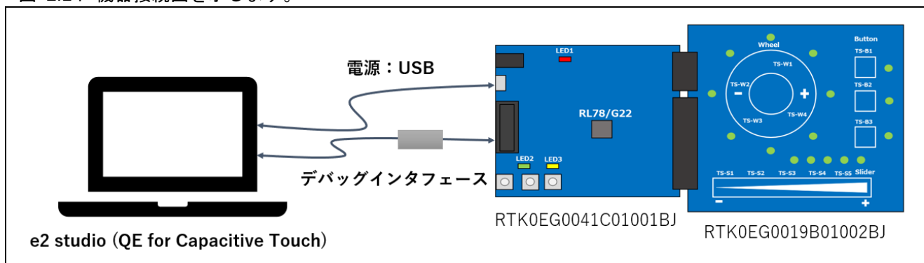
図 2.1 機器接続図
