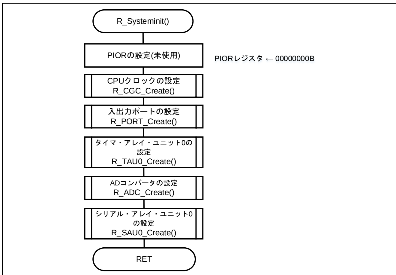
図 3.4 システム関数
