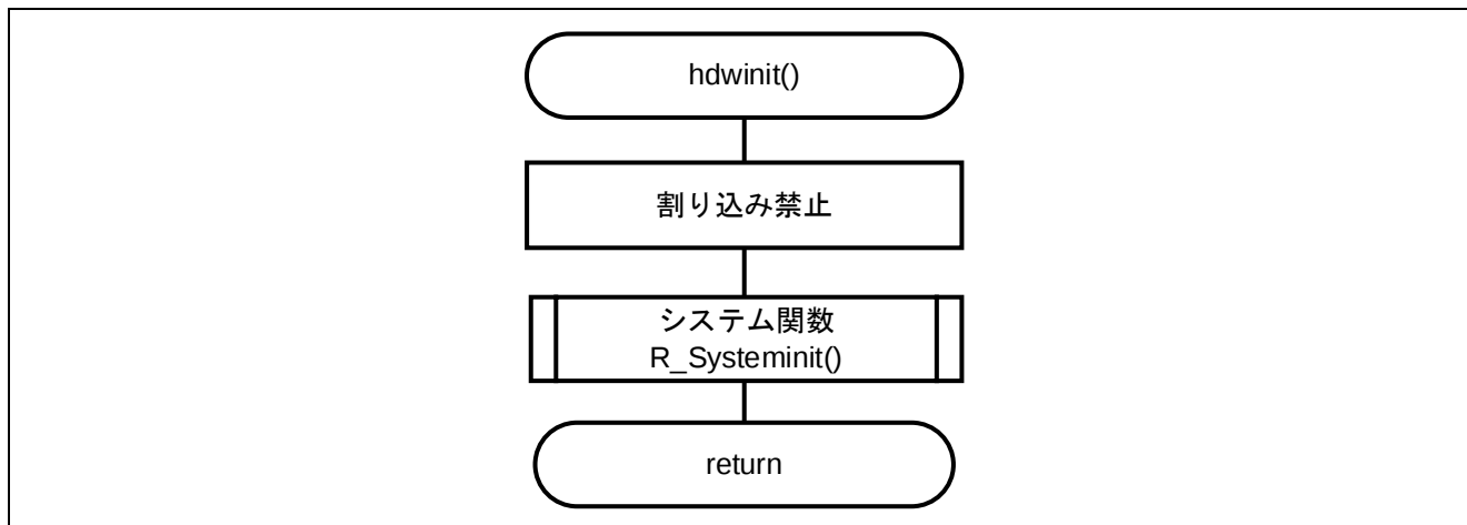
図 3.3 初期設定関数
