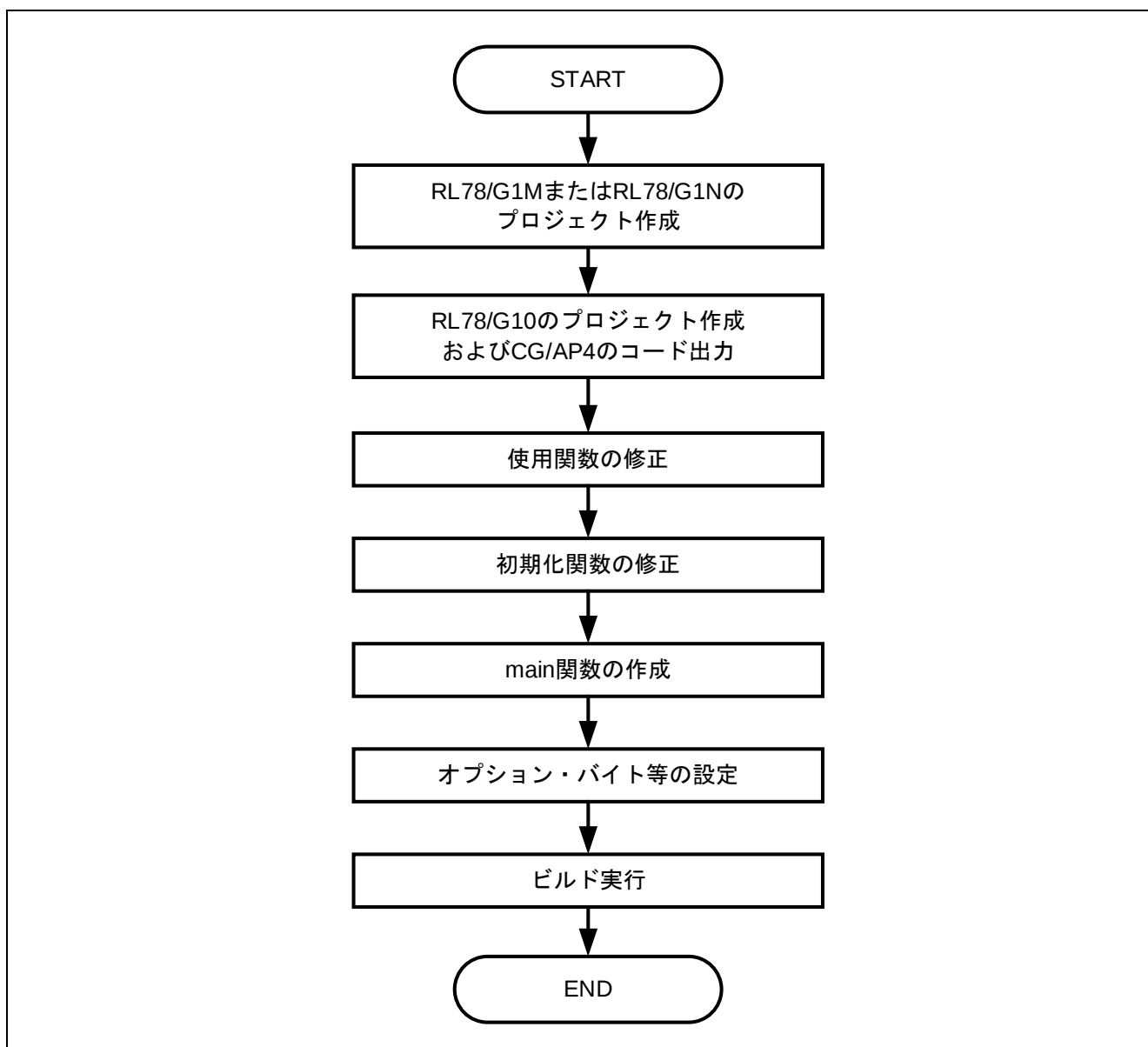
図 1.1 RL78/G10 用 CG/AP4 を使用したプログラム開発フロー
