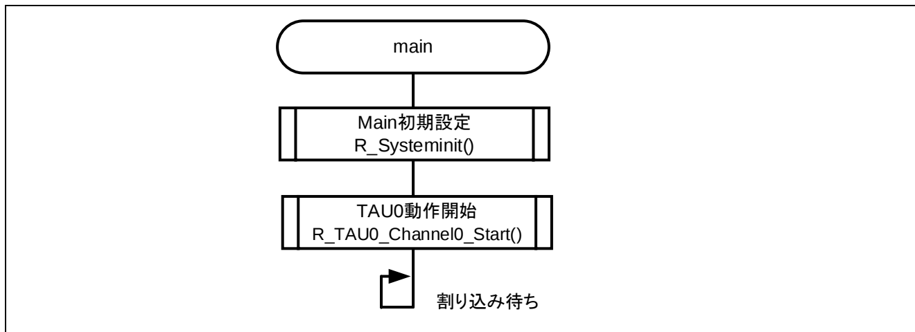
図 3.5 メイン関数
