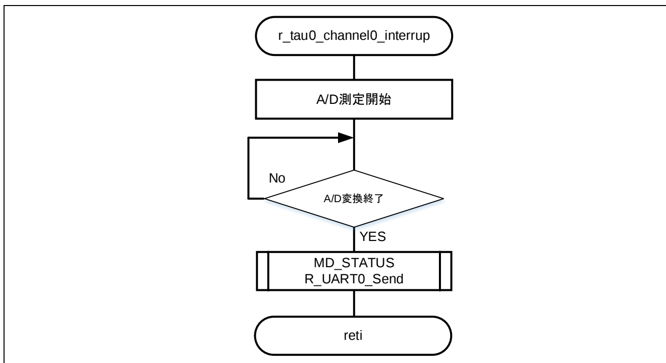
図 3.6 ユーザ関数
