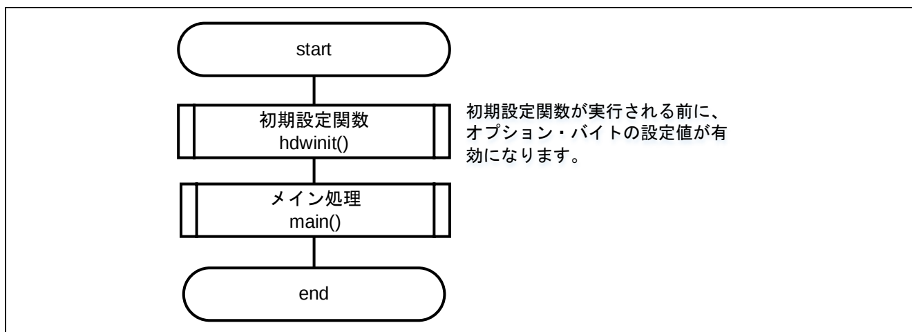
図 3.2 全体フロー
