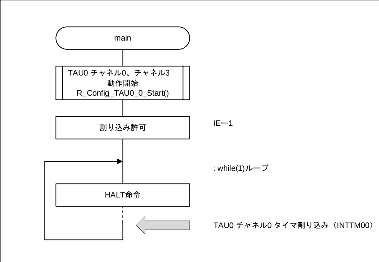
図 4-1 メイン処理
