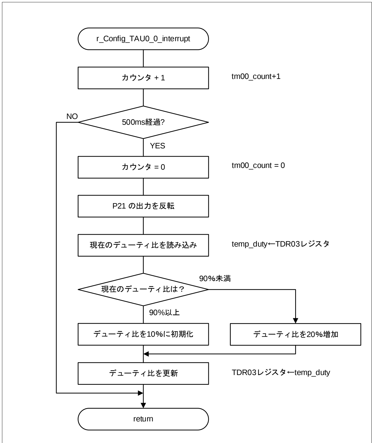
図 4-2 TAU0 チャンネル0のタイマ割り込み処理
