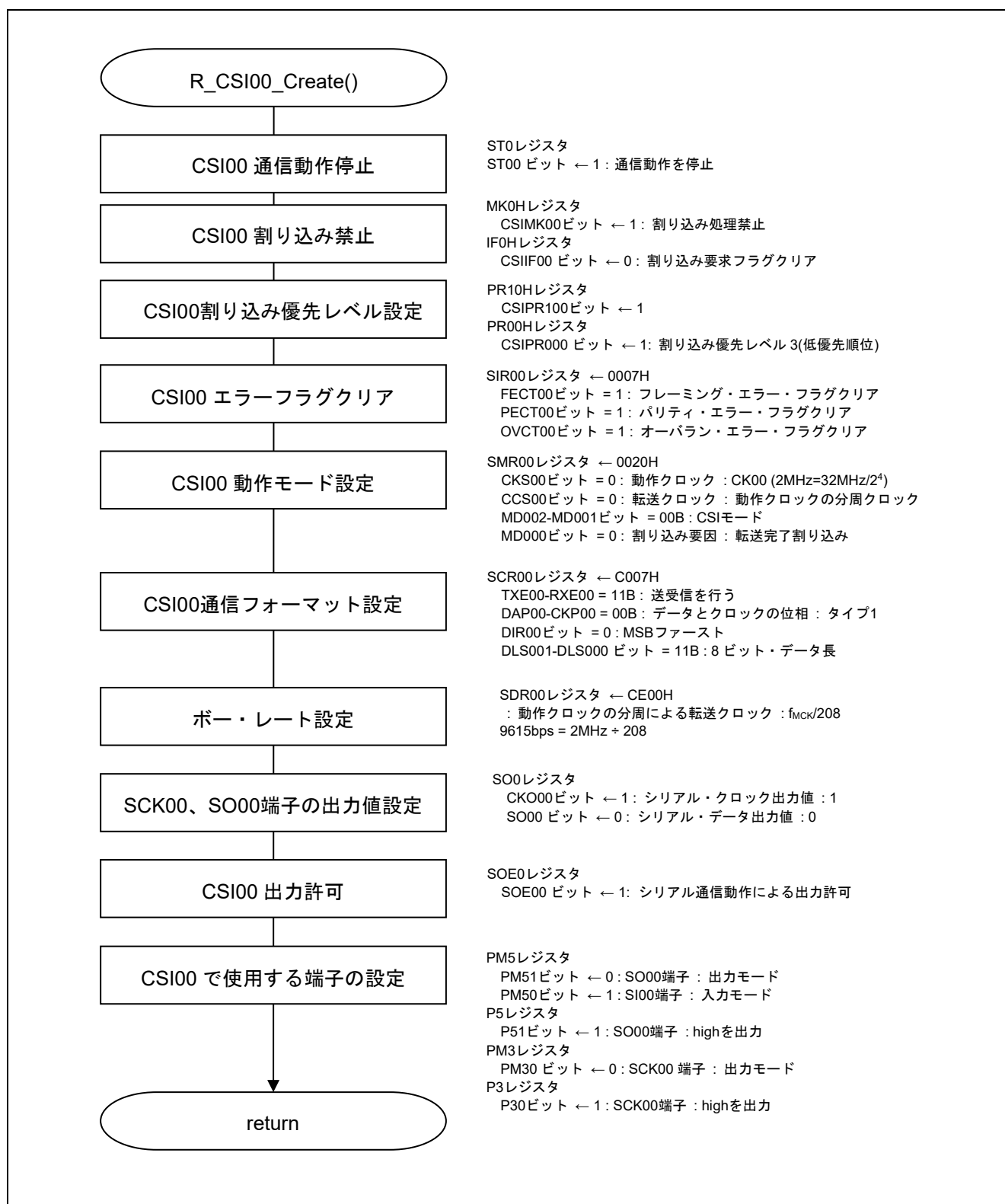
図 5.3 CSI00 初期設定
