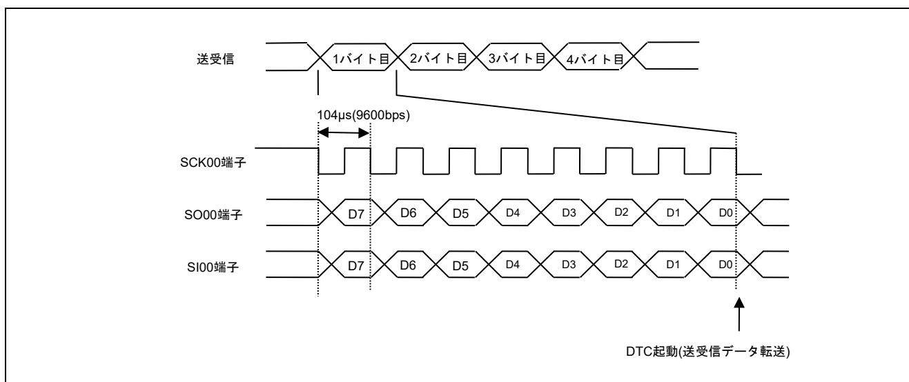
図 1.1 タイミングと通信フォーマット (送受信データ数 4 バイトの場合)
