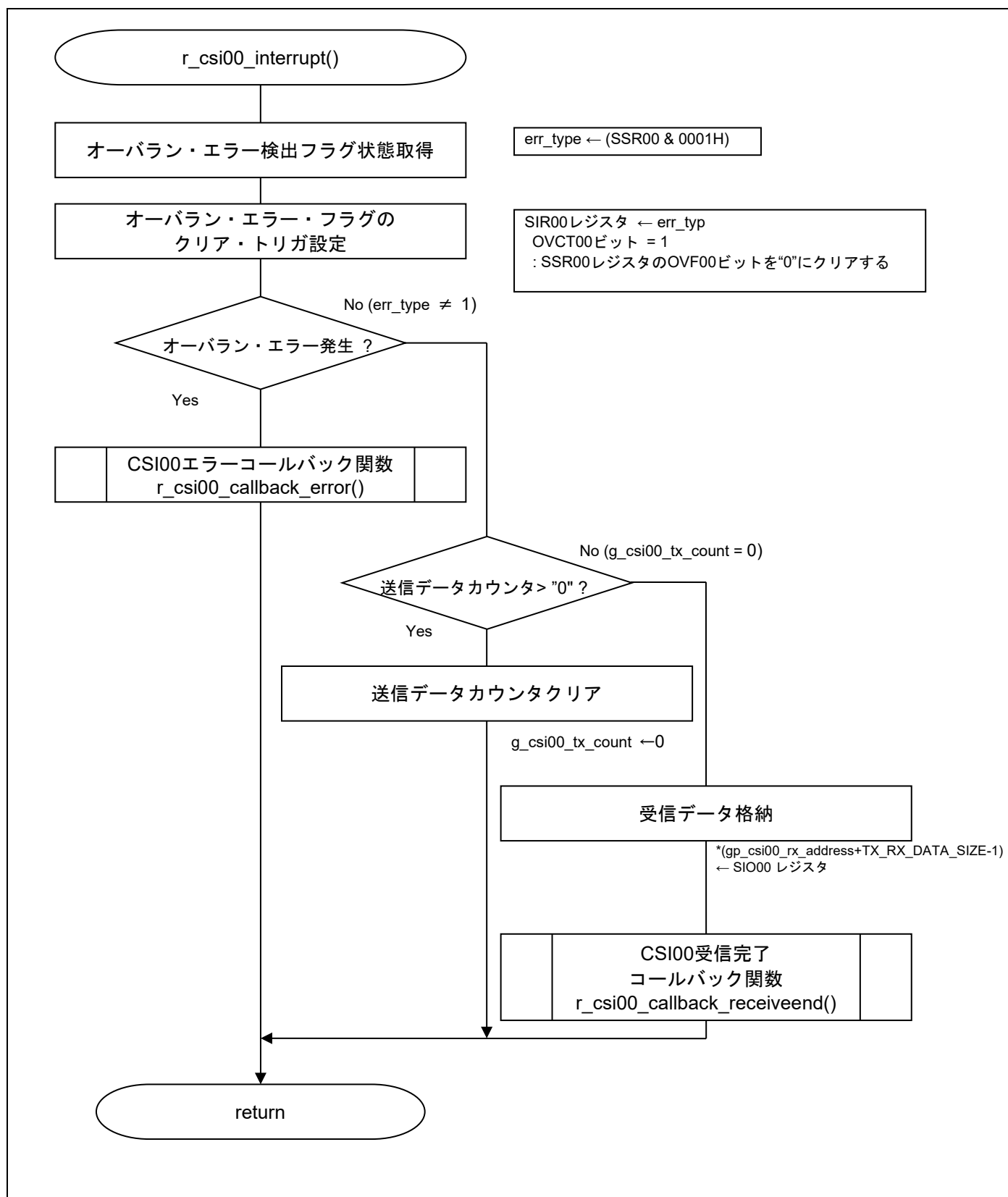
図 5.10 CSI00 転送完了割り込み
