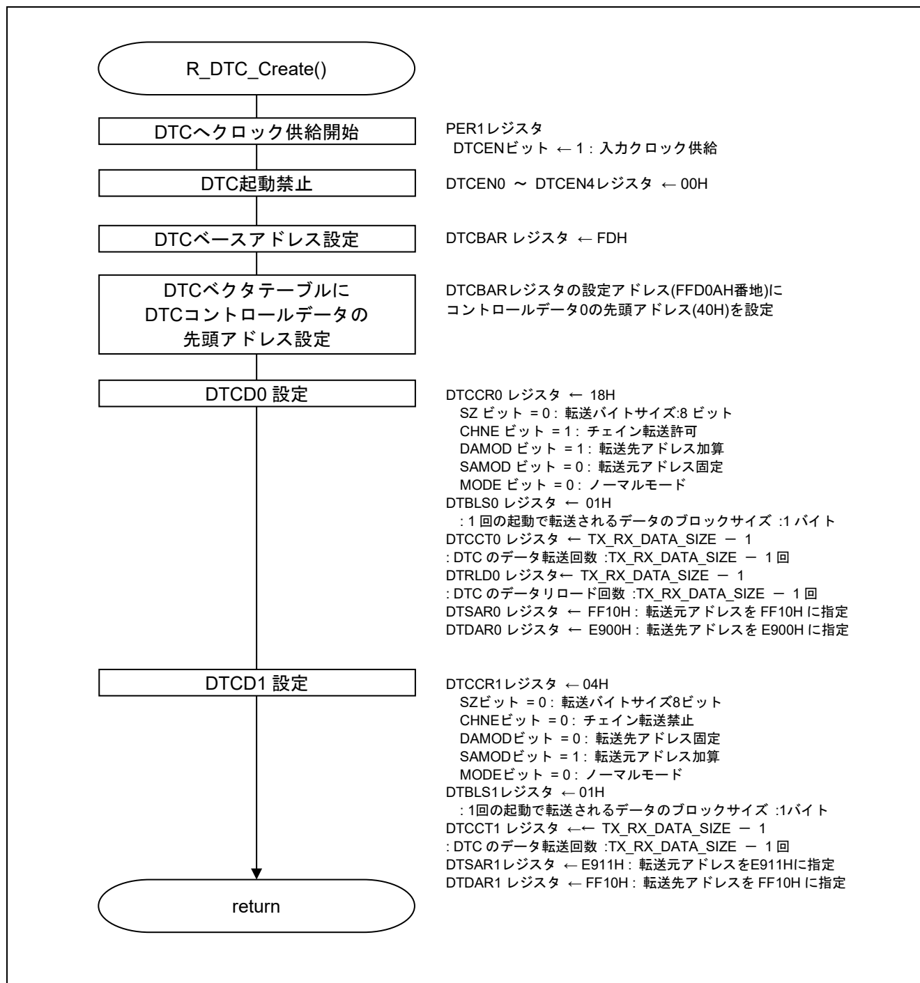
図 5.4 DTC 初期設定
