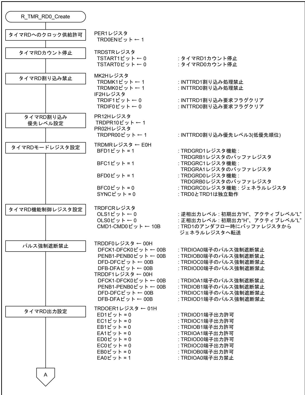
図 4.14 タイマRD初期設定(1/2)
