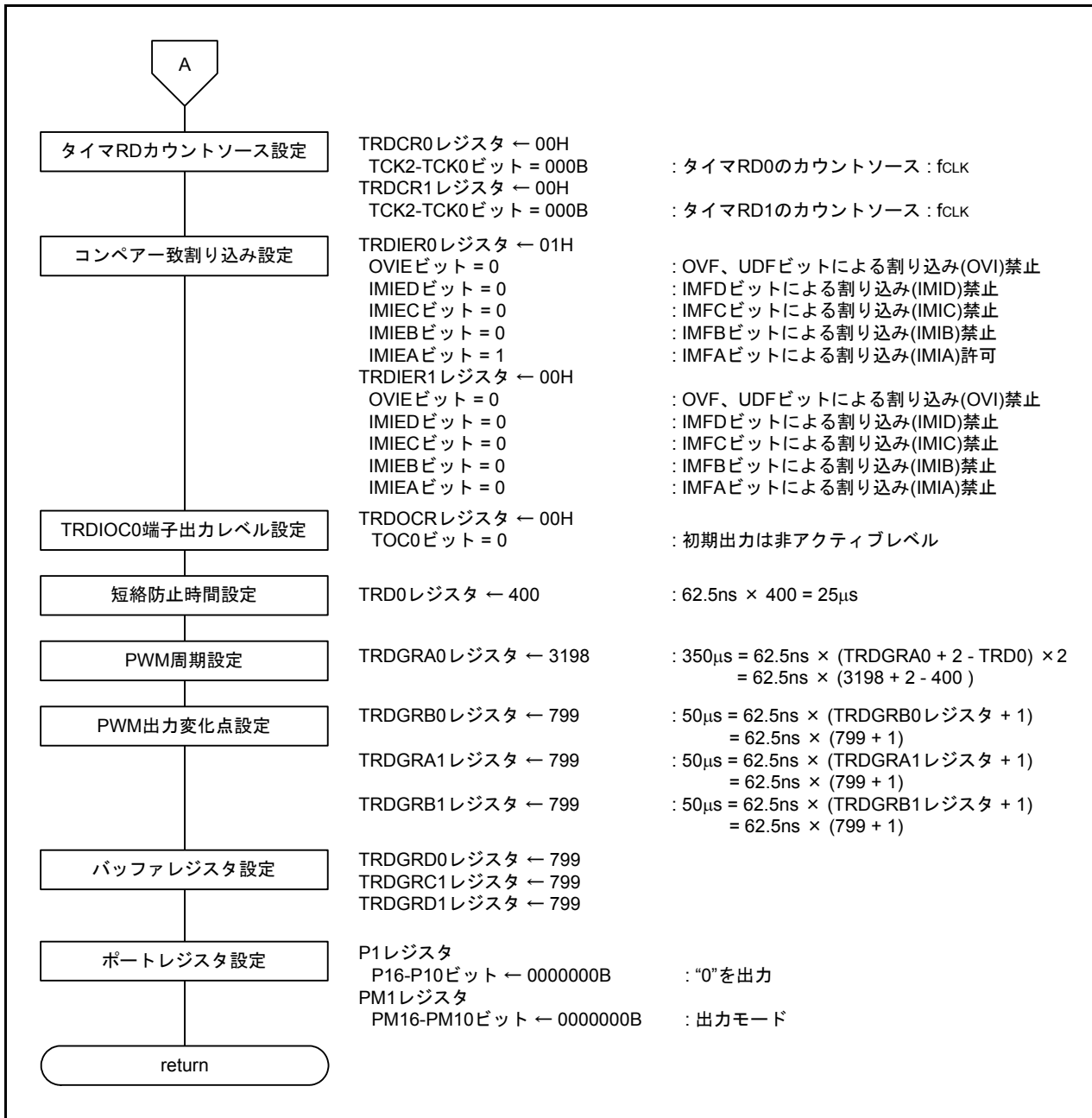
図 4.15 タイマRD初期設定(2/2)
