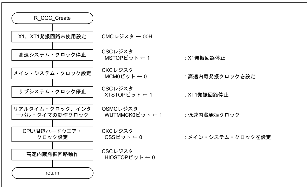
図 4.13 CPU初期設定
