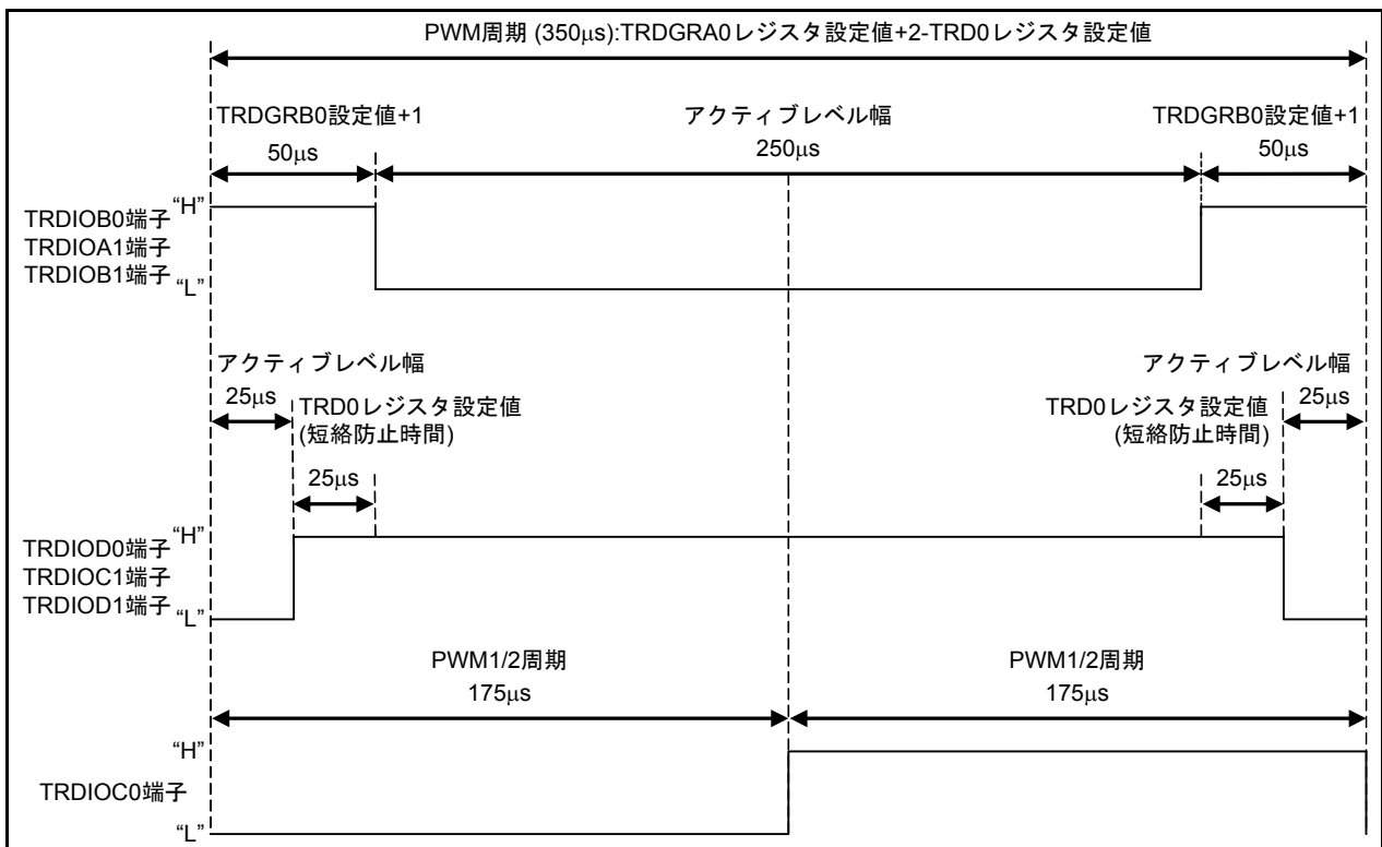
図 4.1 PWM 波形 1
