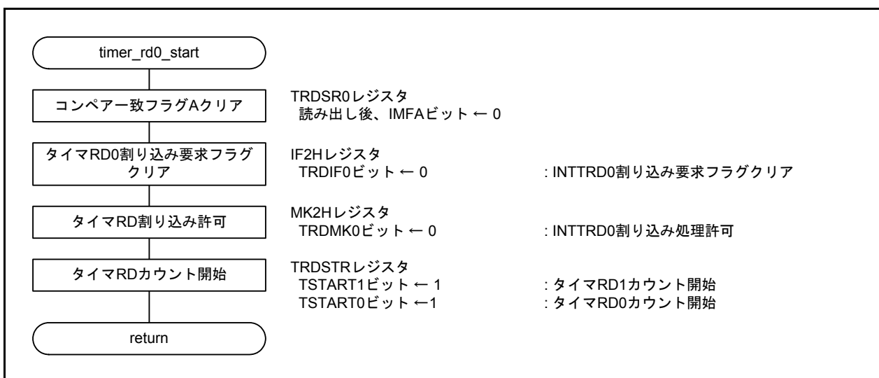
図 4.17 タイマRDカウント開始設定
