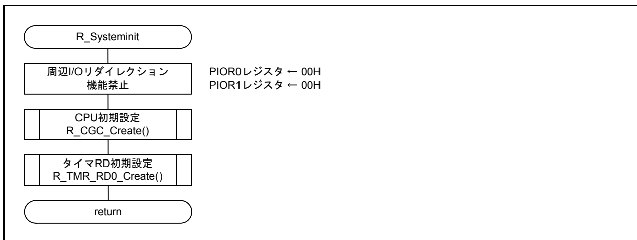
図 4.12 周辺機能初期設定
