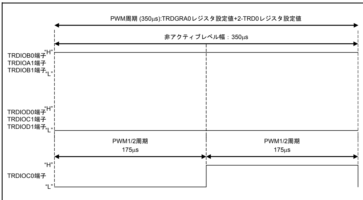
図 4.4 PWM 波形4
