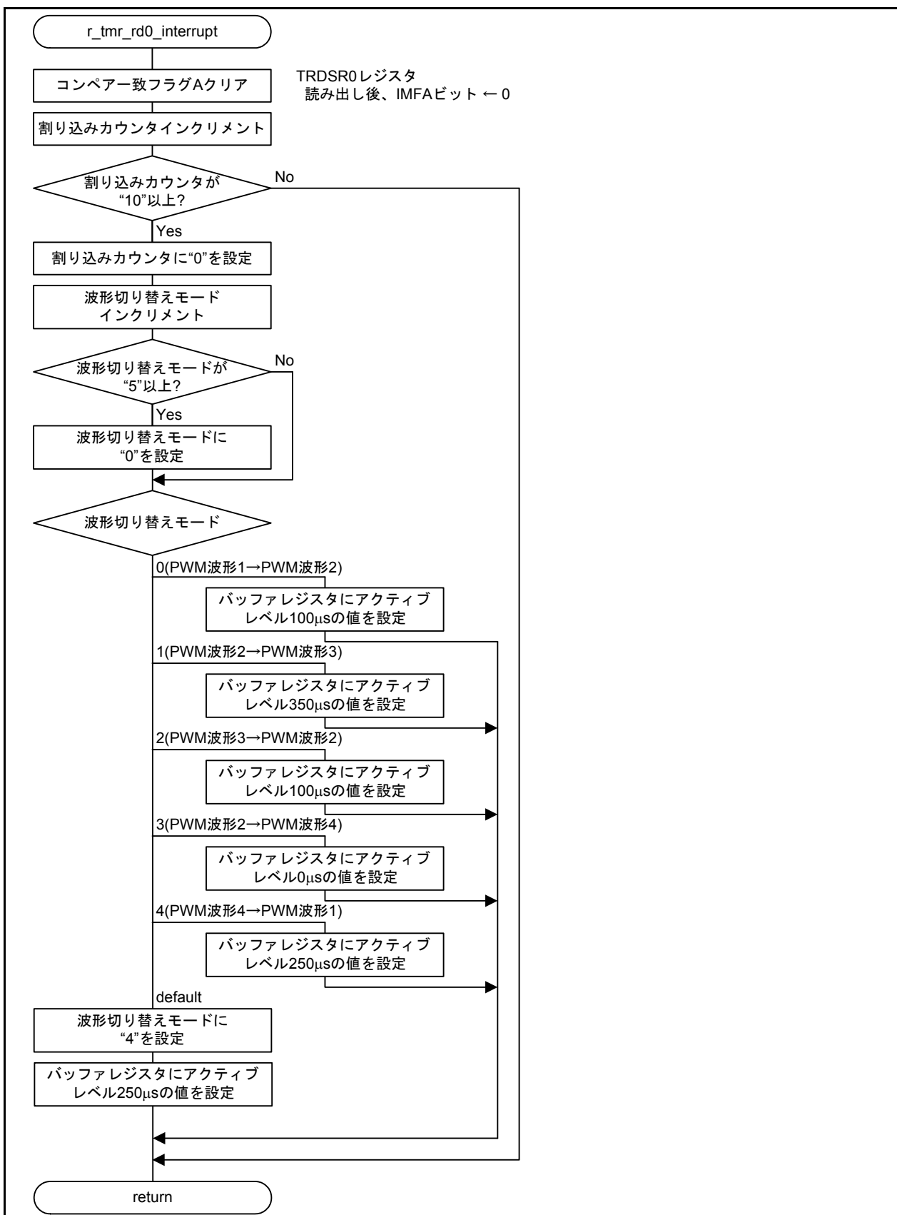
図 4.18 タイマRD0割り込み
