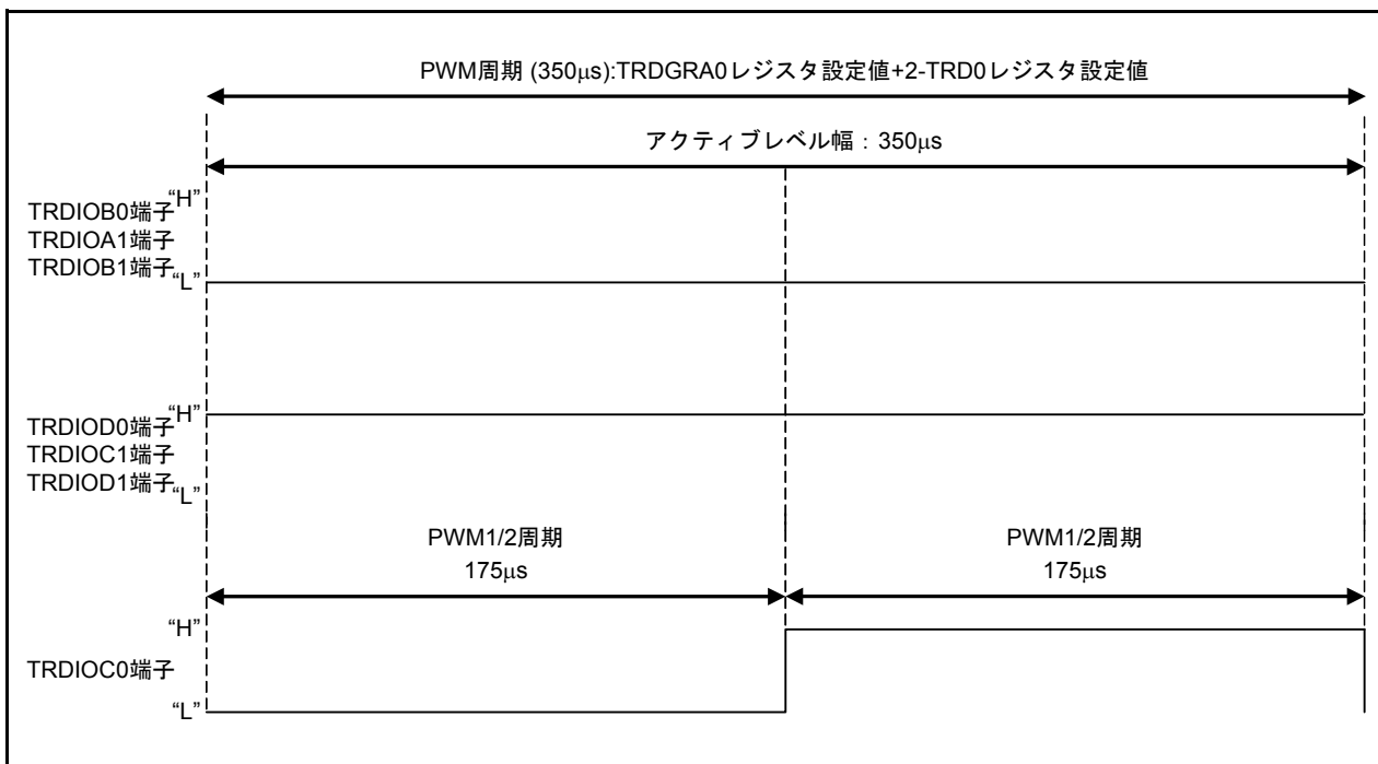
図 4.3 PWM 波形3
