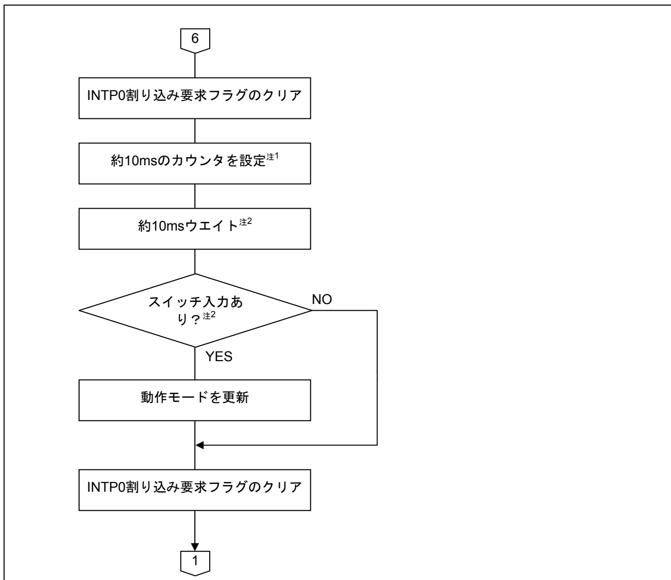
図 5.9 メイン処理 (3/3)
