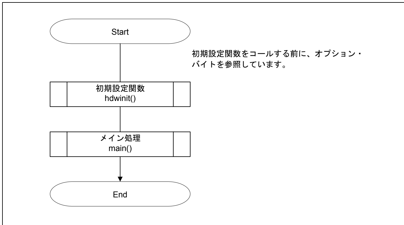
図 5.1 全体フロー
