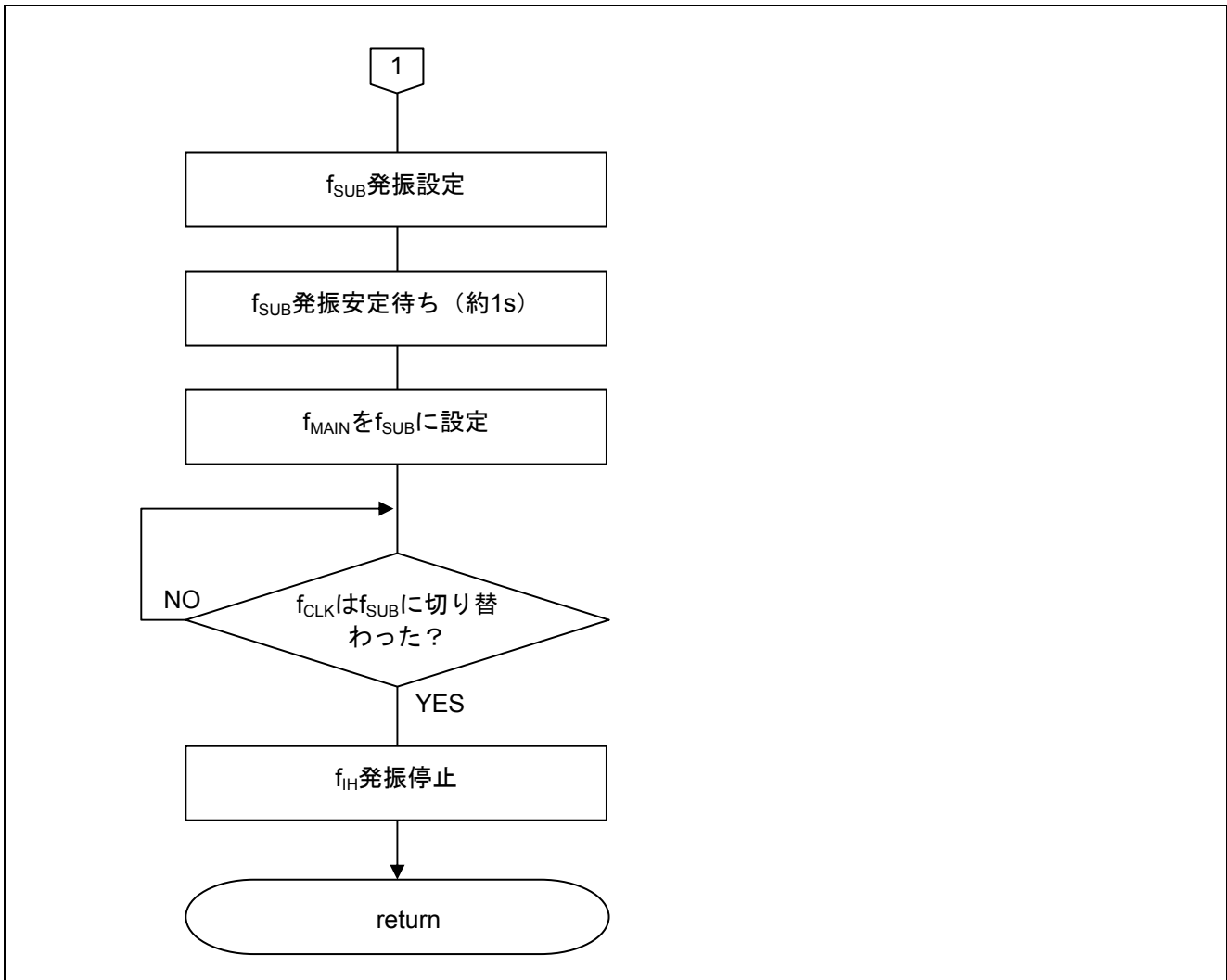
図 5.12 CPU/周辺ハードウェア・クロック切り替え処理 (2/2)
