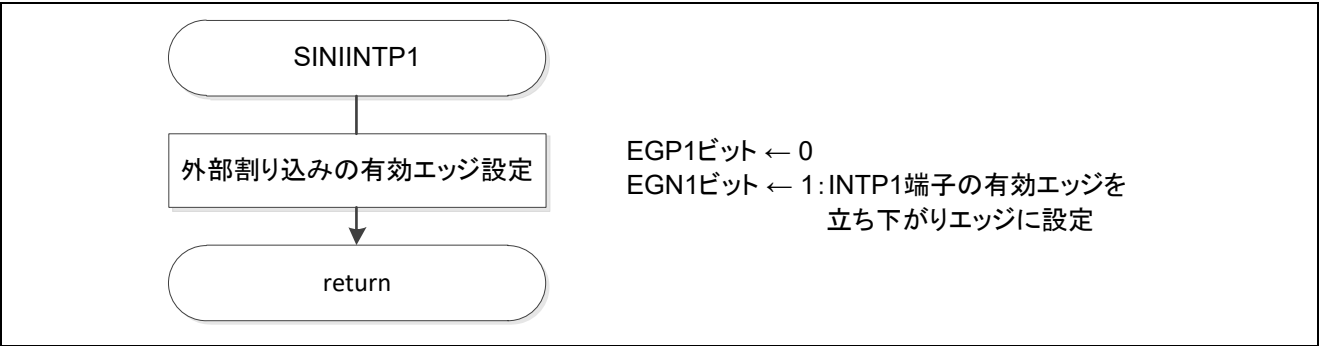
図 5.5 外部割り込みの設定
