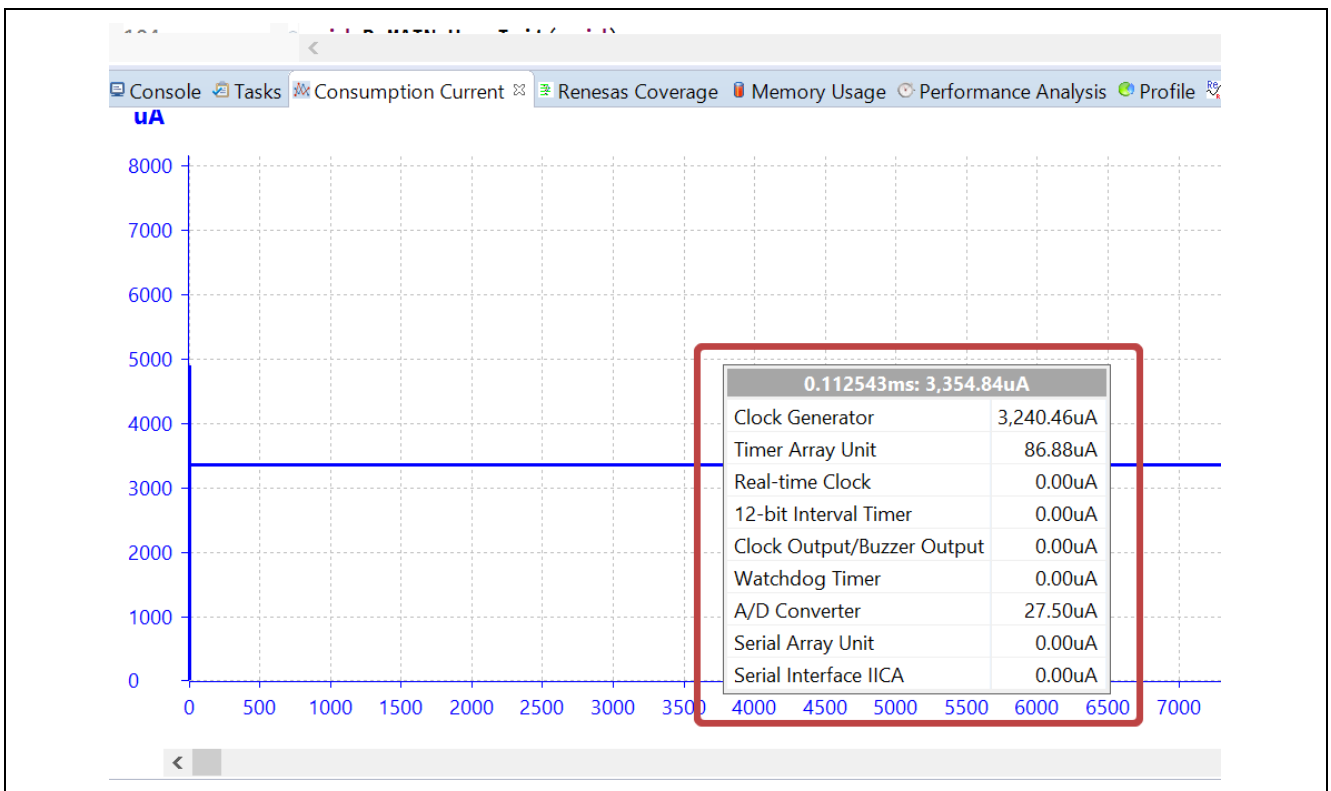
图 25 “Consumption Current”视图的具体信息
