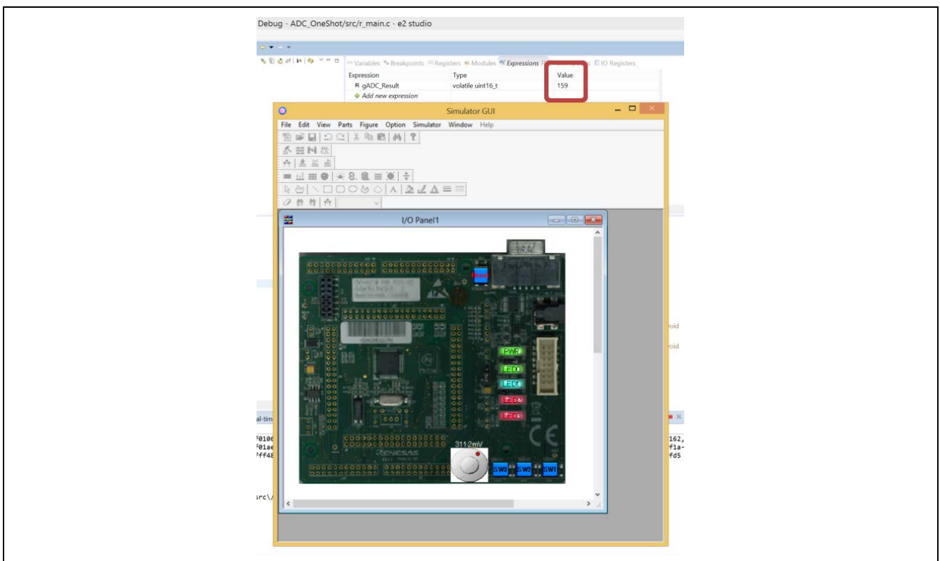
图 21 “Expressions” 面板上显示 “gADC_Result”（8 位分辨率）
