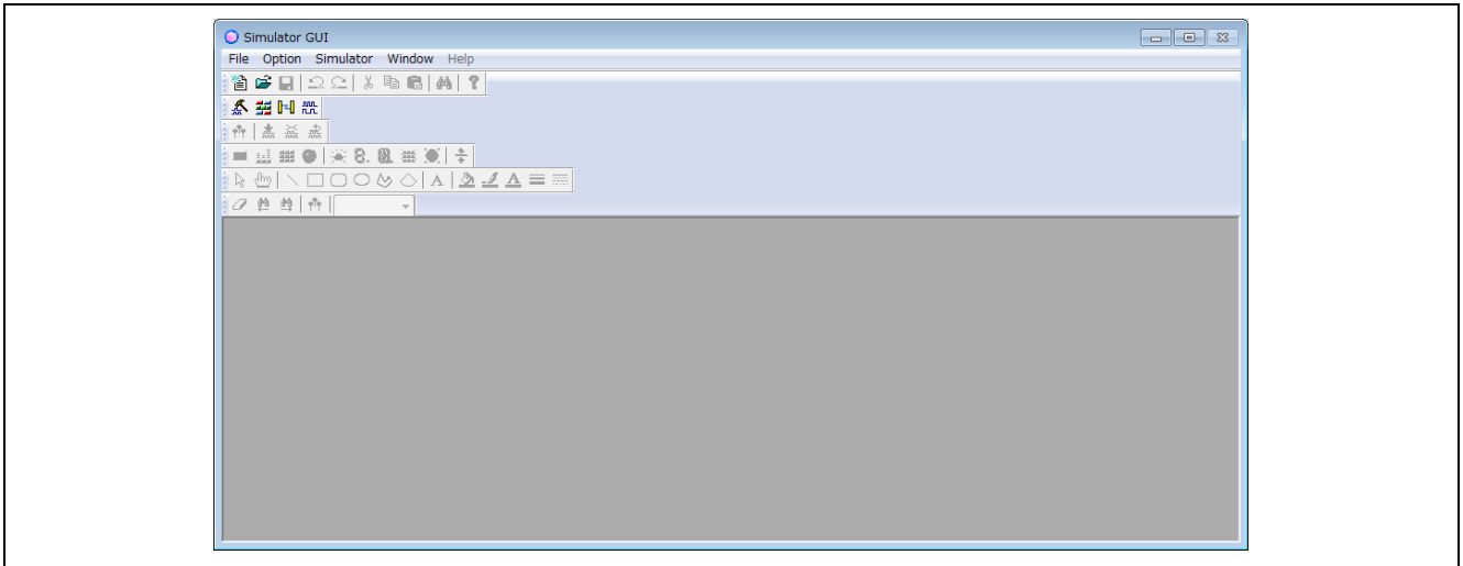
图 12 Simulator GUI
