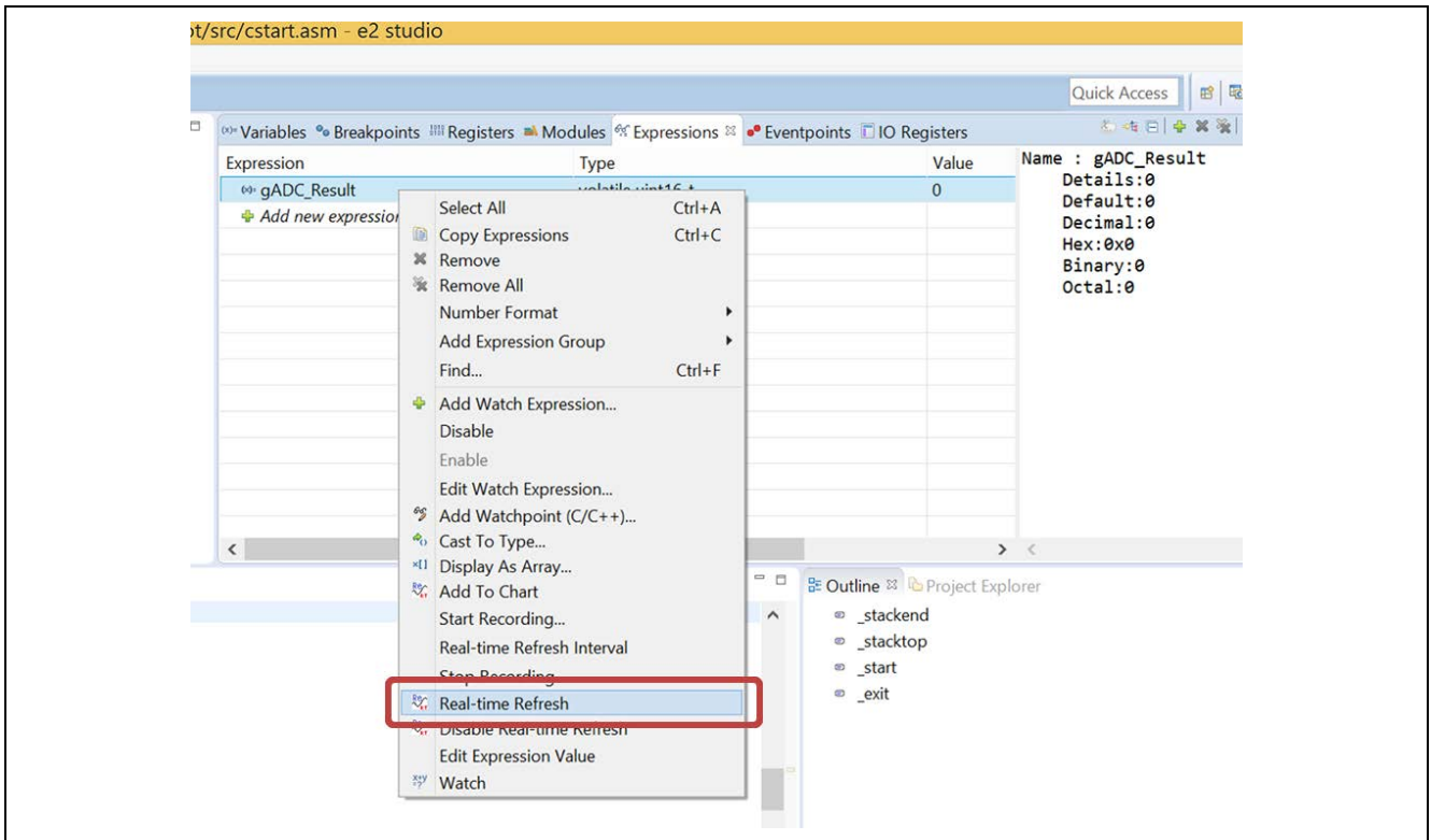
图 16 “Expressions” 菜单
