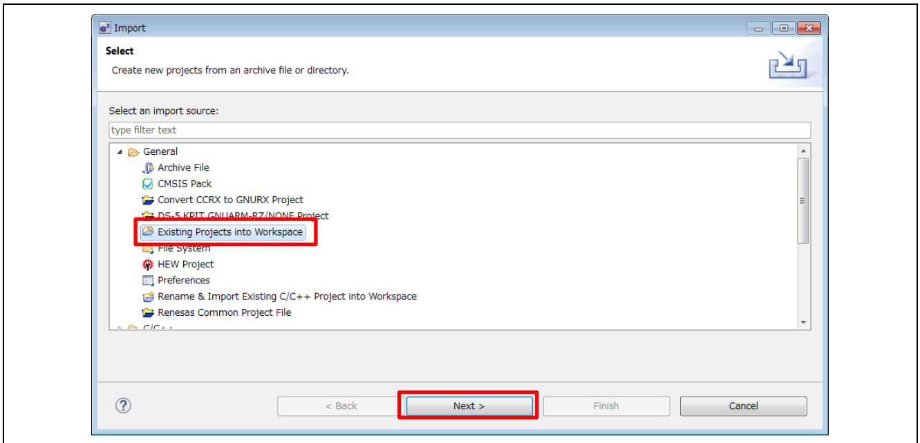
图 2 导入对话框（1/2）
