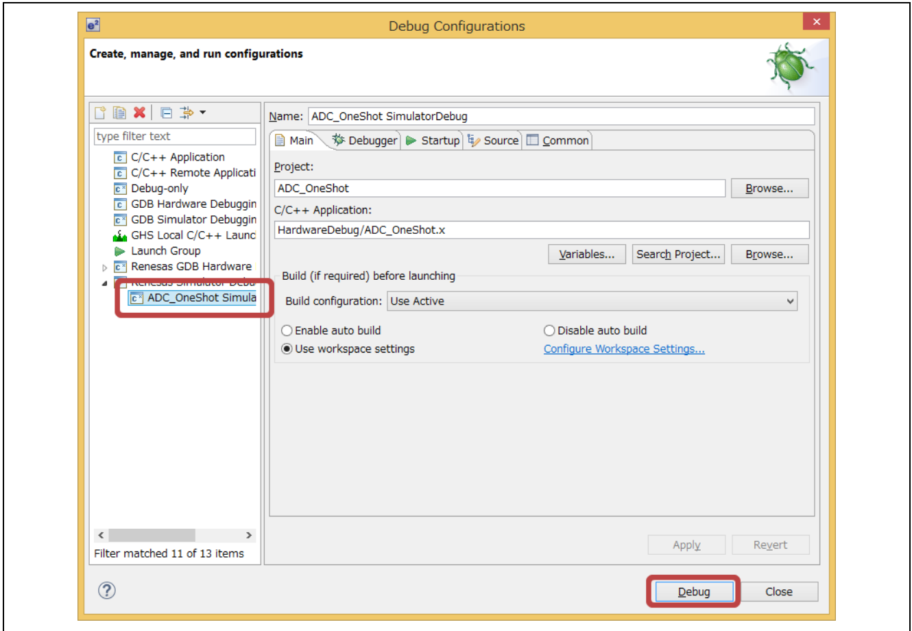
图 10 调试的配置
