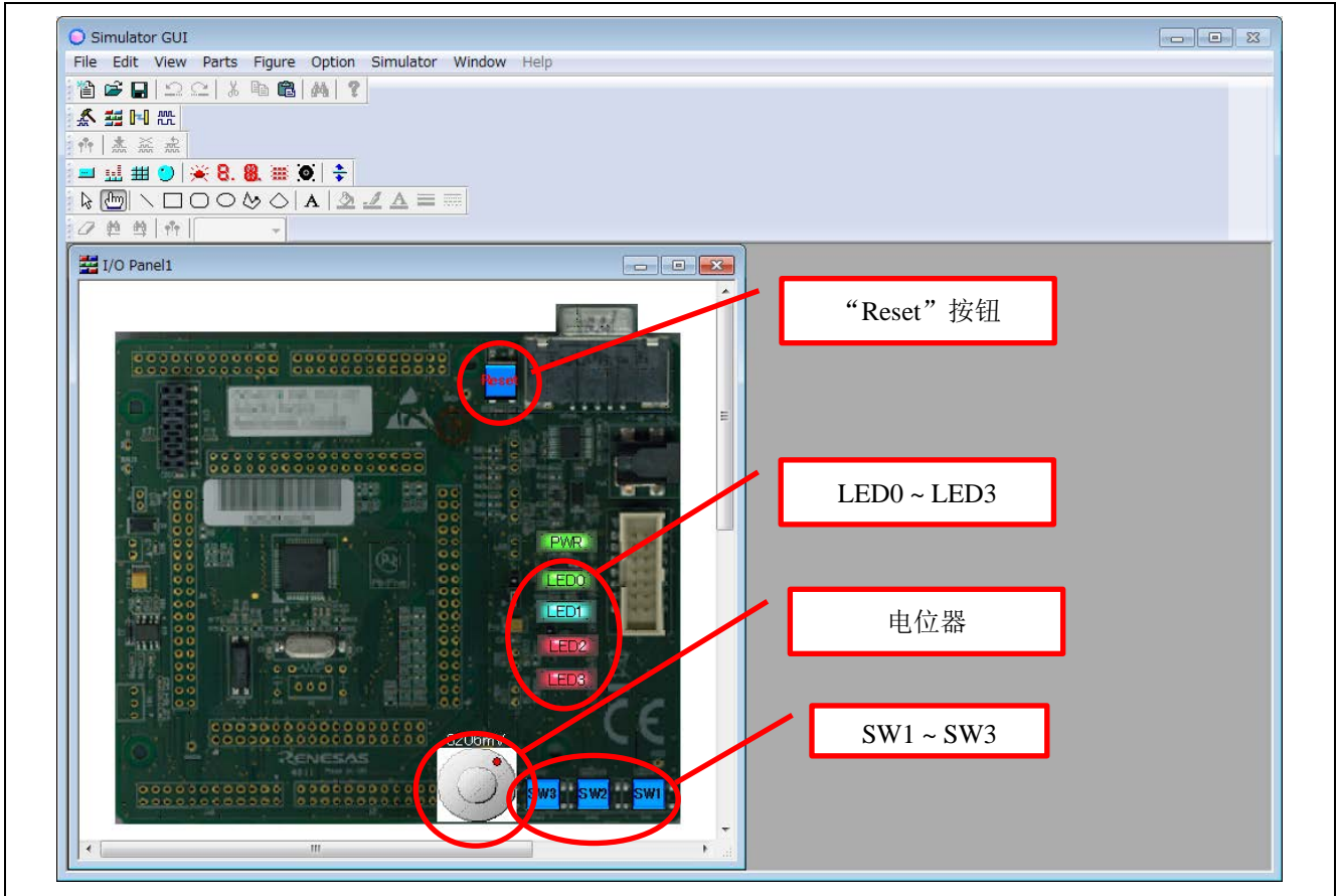
图 14 I/O Panel
