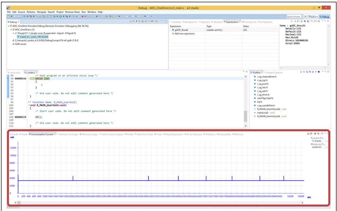
图 23 “Consumption Current” 视图中的结果
