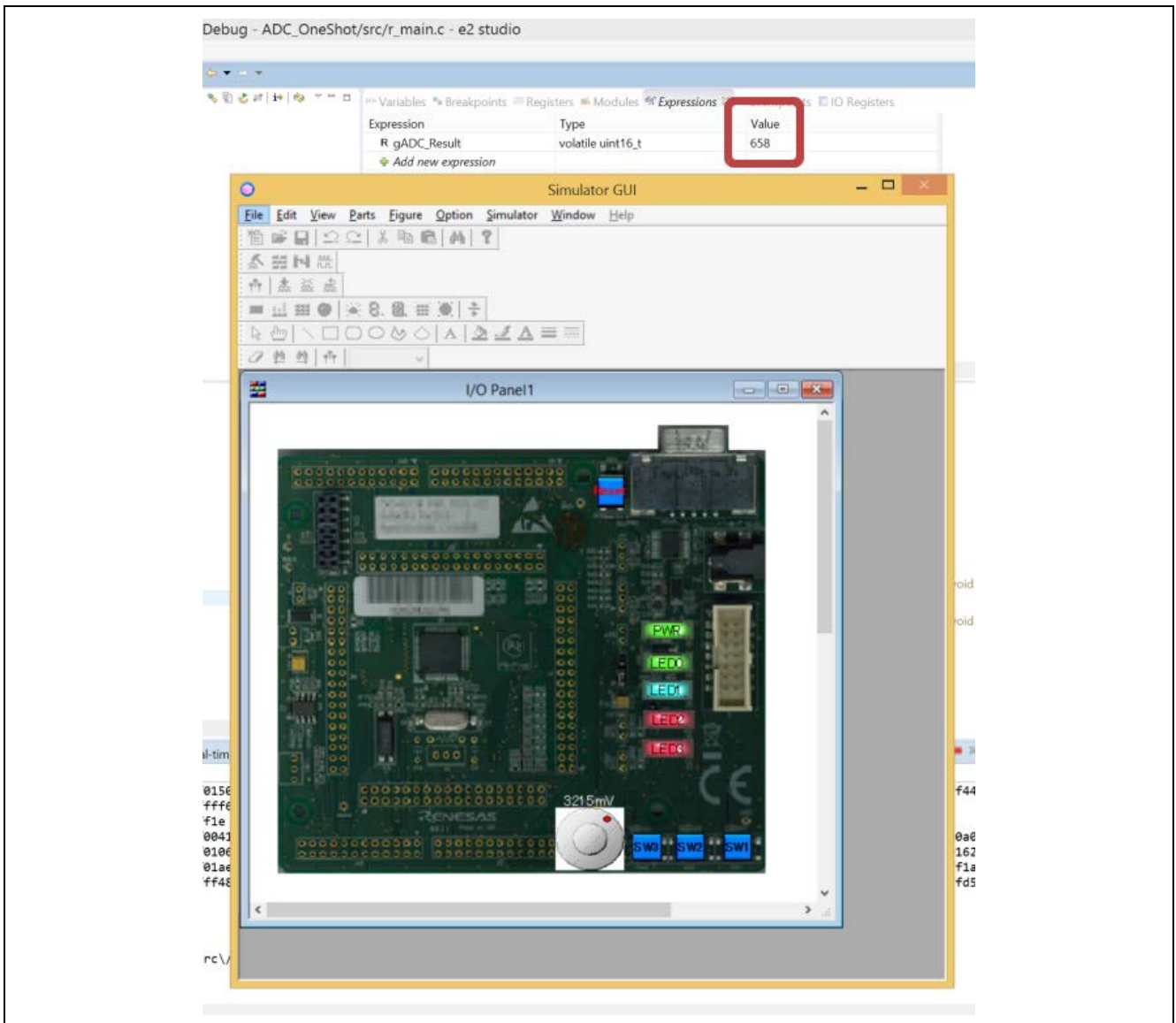
图 19 “Expressions”面板上显示“gADC_Result”（1/2）
