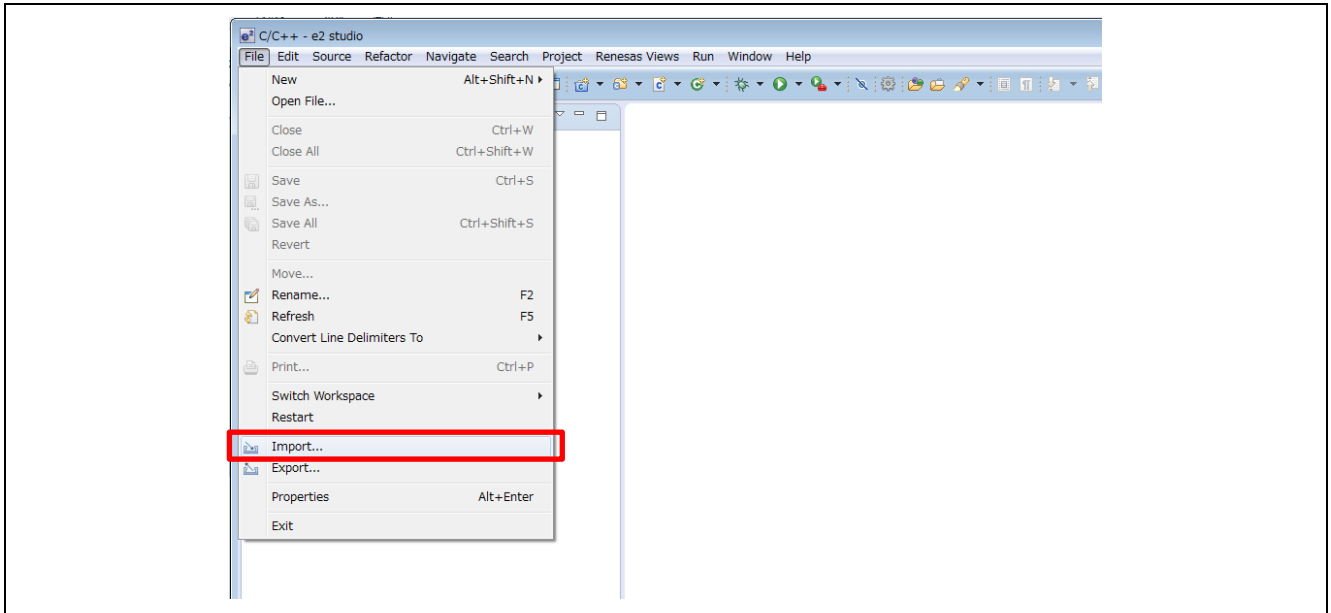
图 1 文件菜单
