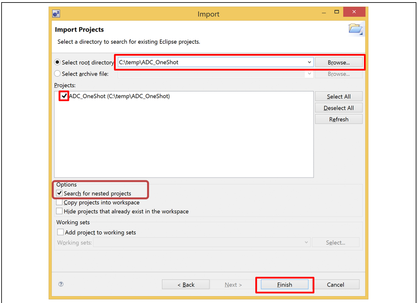
图3 导入对话框（2/2）
