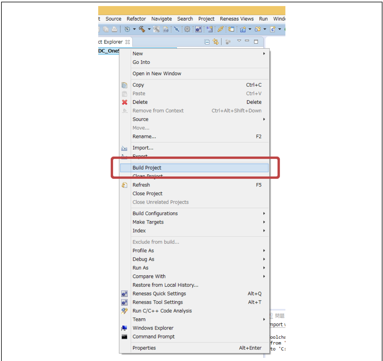
图 5 编译工程
