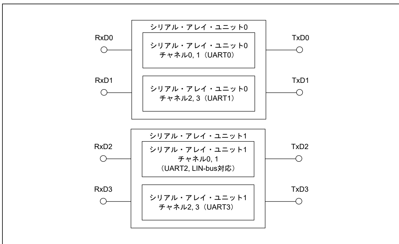
図 1.2 シリアル・アレイ・ユニット (SAU) UART のブロック図
