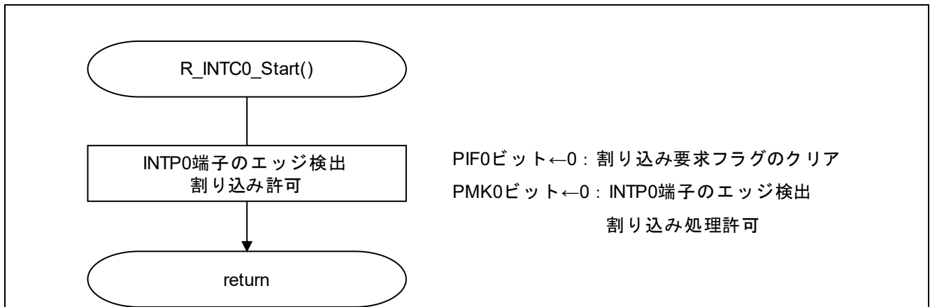
図 5.10 INTPO の動作開始
