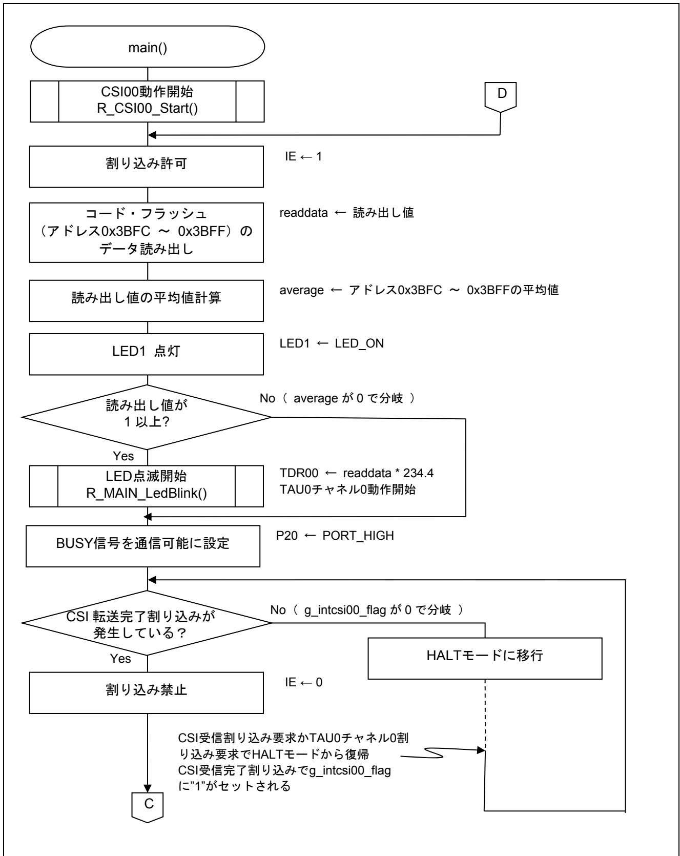
図 5.10 メイン処理(1/2)
