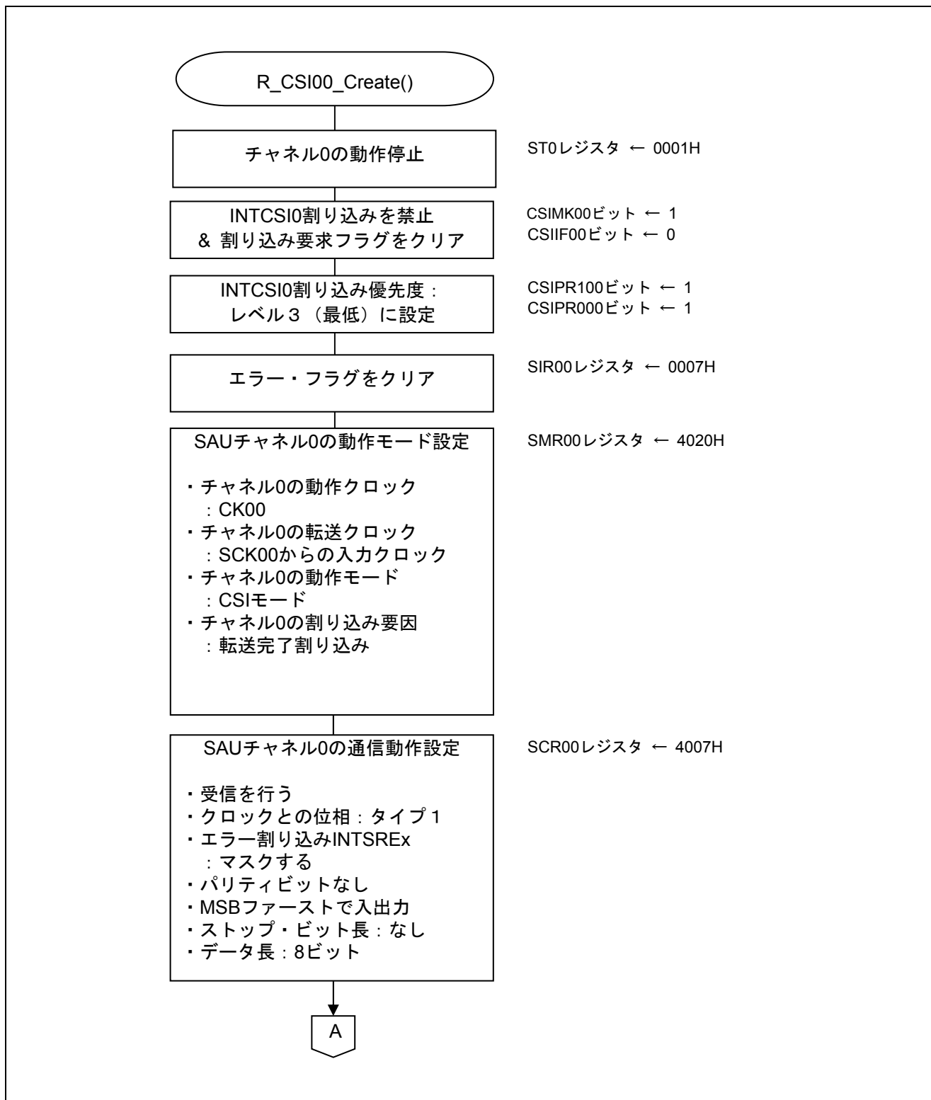
図 5.7 CSI00 の設定 (1/2)
