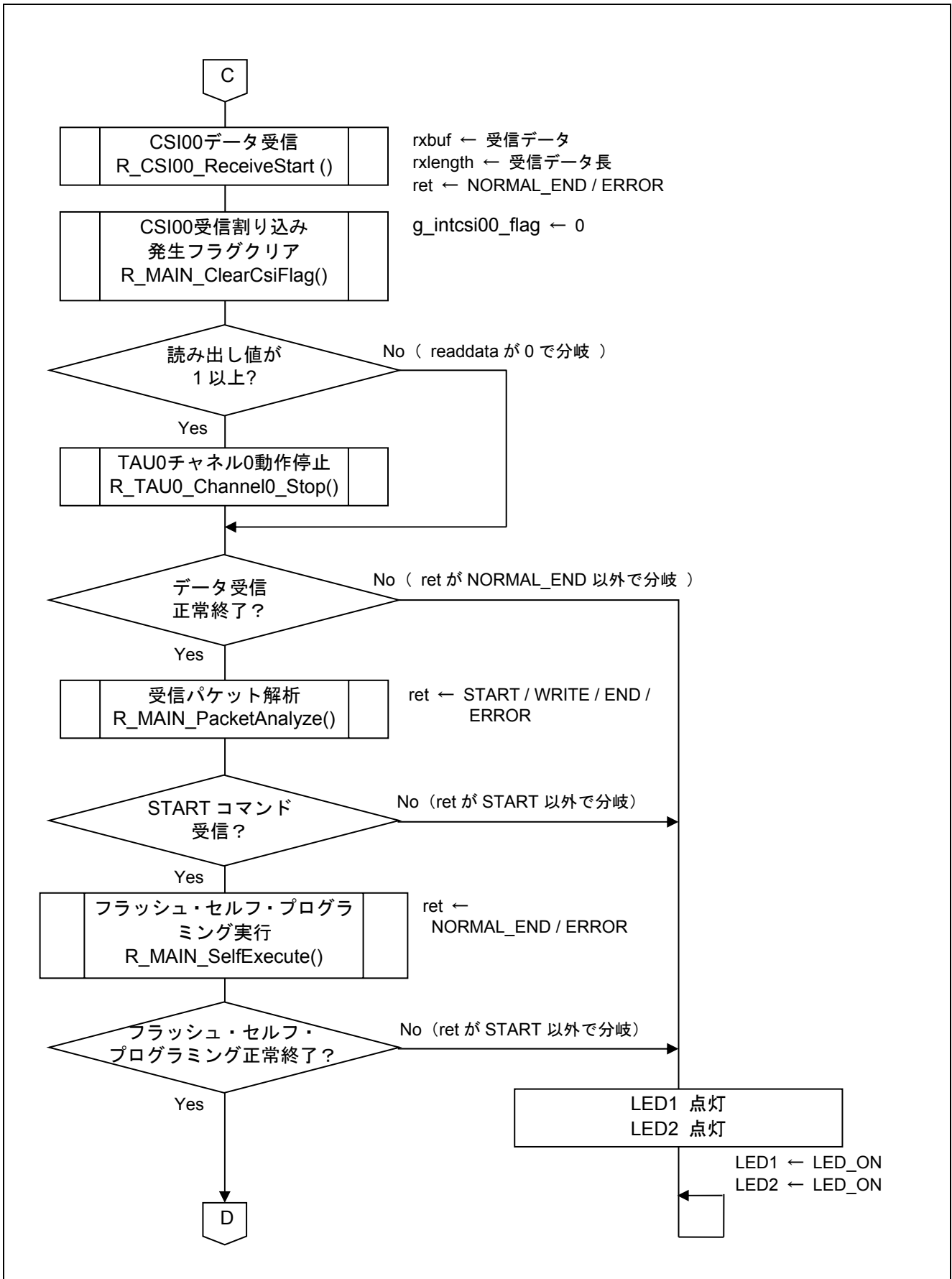
図 5.11 メイン処理(2/2)
