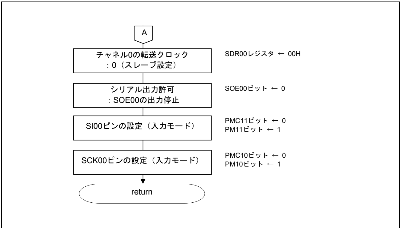
図 5.8 CSI00 の設定 (2/2)
