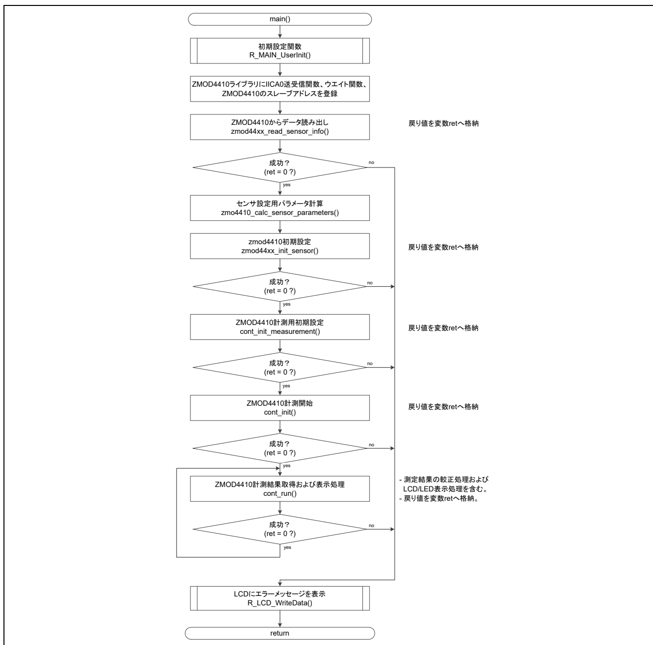
図 5.1 メイン関数
