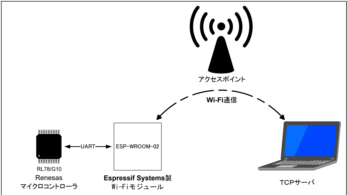
図 5.1 応用サンプルプログラム システム構成例
