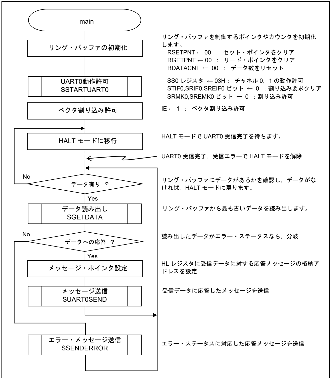
図 5.7 メイン処理
