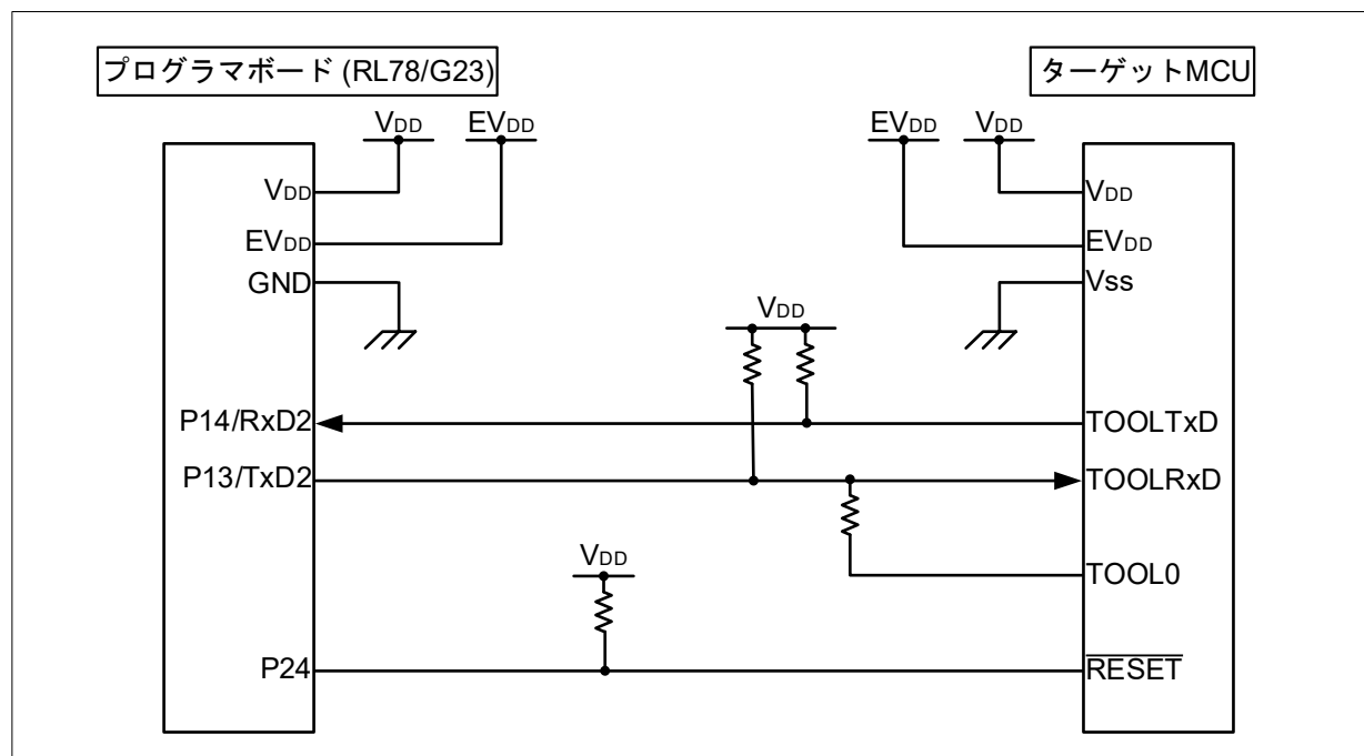
図 4-3 2 線 UART
