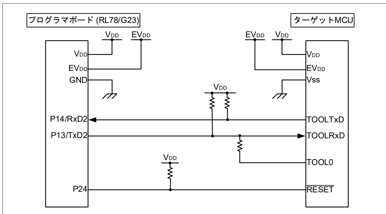
図 4-3 2 線 UART
