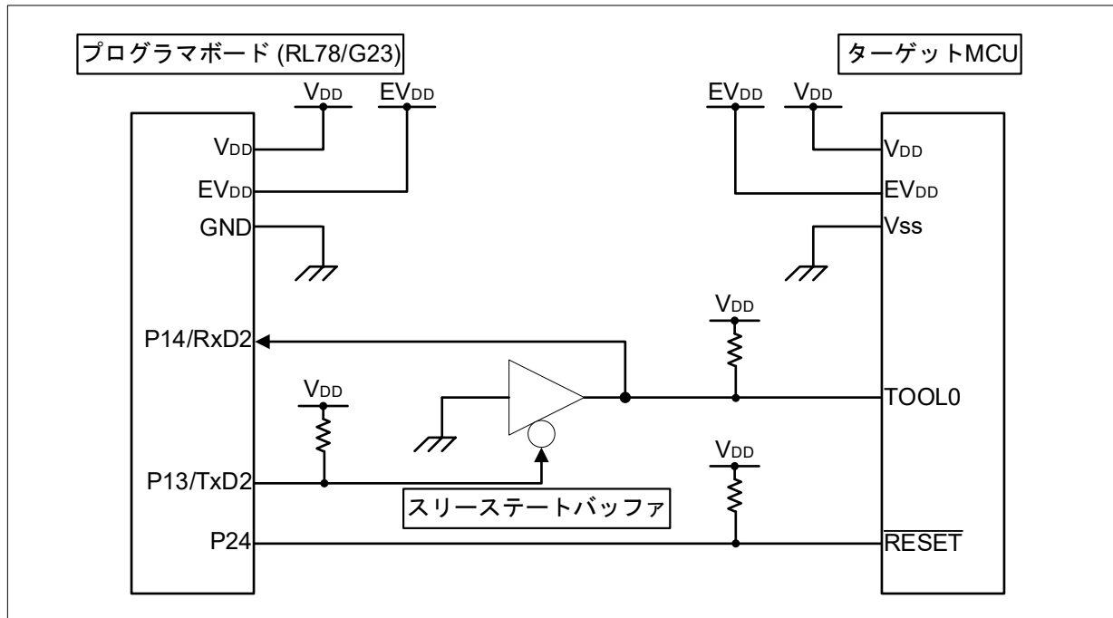
図 4-2 1 線 UART
