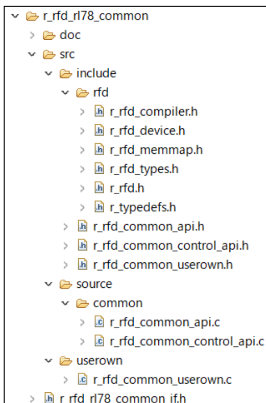
展開時の r_rfd_rl78_common フォルダ
