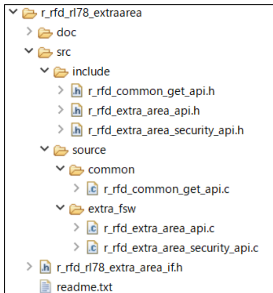
展開時の r_rfd_rl78_extrarea フォルダ
