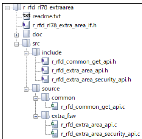
展開時の r_rfd_rl78_extraarea フォルダ
